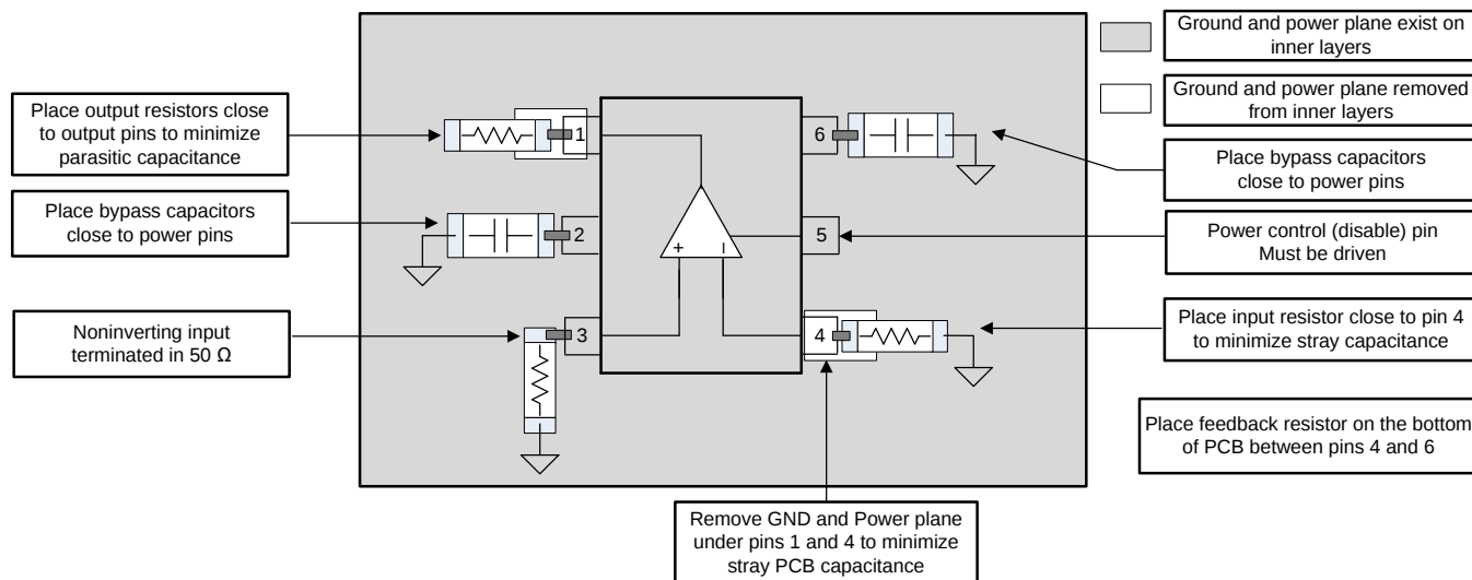
图 38. Layout Example
