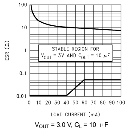
图 7-6. 3.0-V, 10- \mu\text{F} ESR Curves (Legacy Chip)
