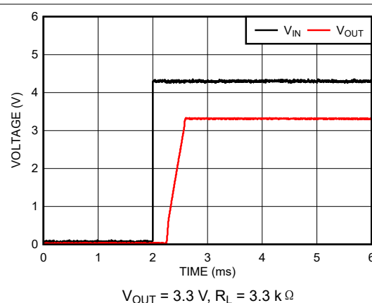
图 7-10. Turn-on Waveform (New Chip)
