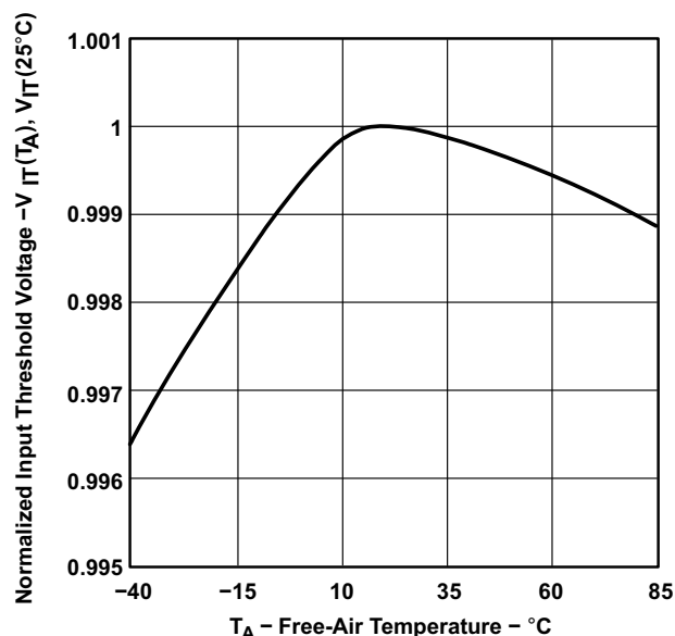
标准化输入阈值电压与大气温度间的关系
