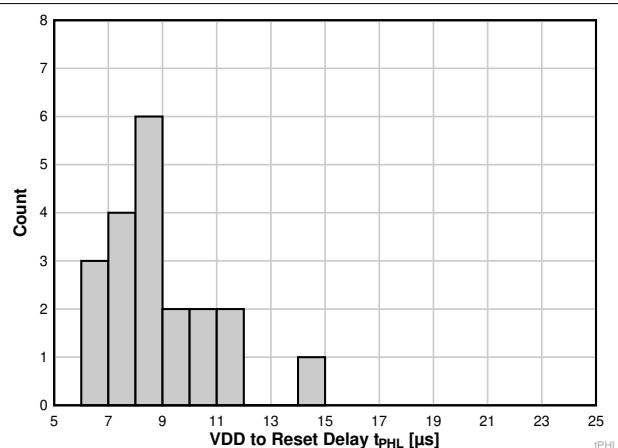
图 7-16. TPS3823A-33 器件在 25°C 时的 VDD 至复位延时直方图 (单位数 = 20)
