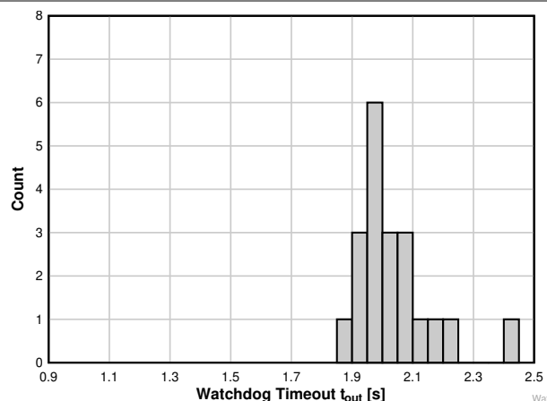
图 7-13. TPS3823A-33 器件在 25^{\circ}\text{C} 时的看门狗超时直方图 (单位数 = 20)
