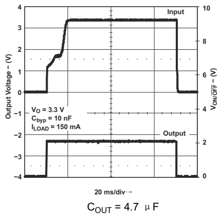
图 8-23. Turn-On Time
