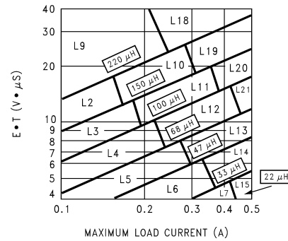
图 9-13. LM2674, Adjustable Version
