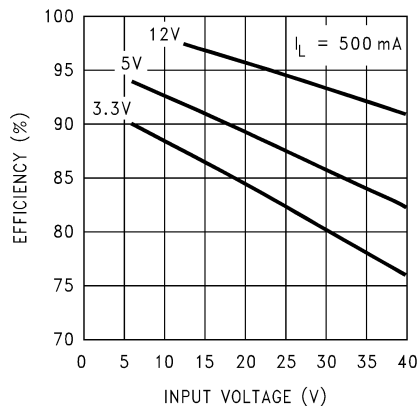
图 7-3. Efficiency
