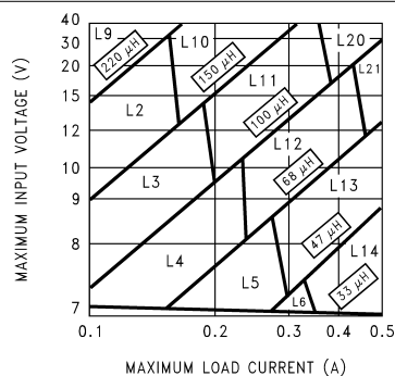
图 9-11. LM2674, 5-V Version
