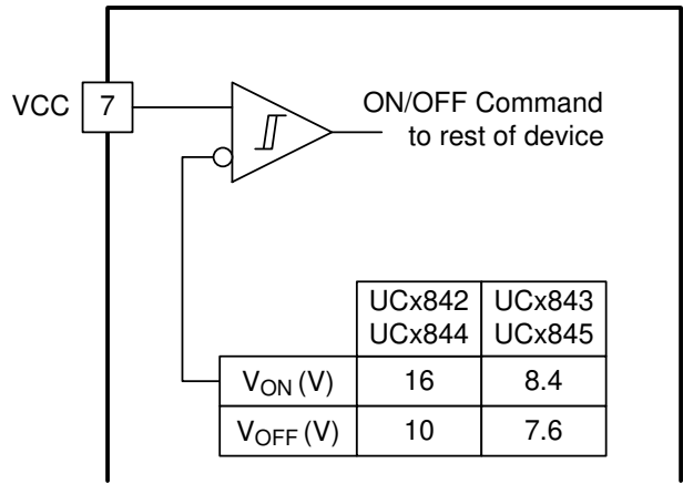
图 8-5. UVLO 阈值
