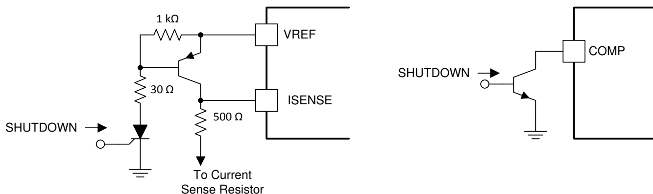
图 8-10. 关断技术
