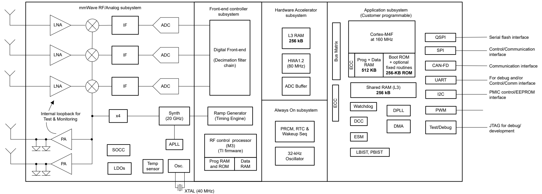
图 9-1. 功能方框图
