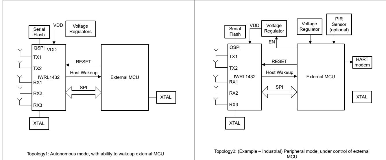
图 8-1. System Topologies
