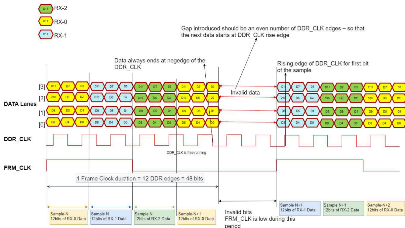
图 7-14. RDIF Data Format
