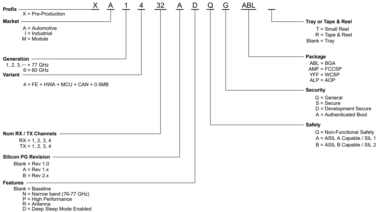
图 10-1. Device Nomenclature
