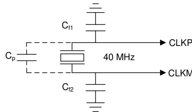
图 7-8. Crystal Implementation
