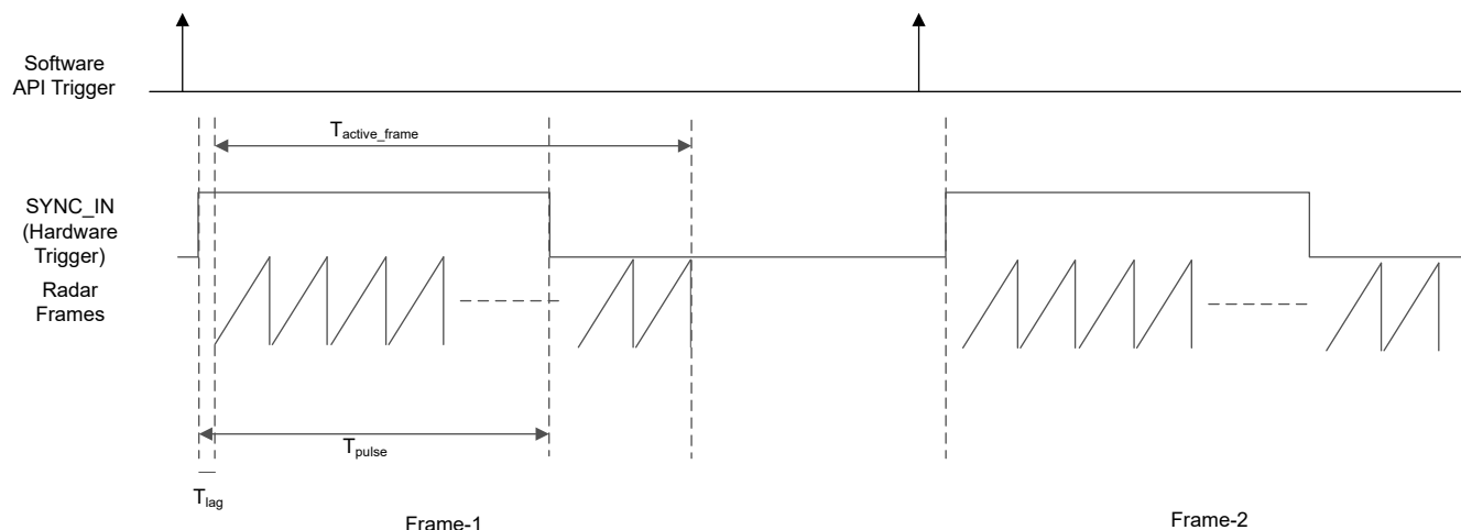
图 7-11. SYNC IN 硬件触发器
