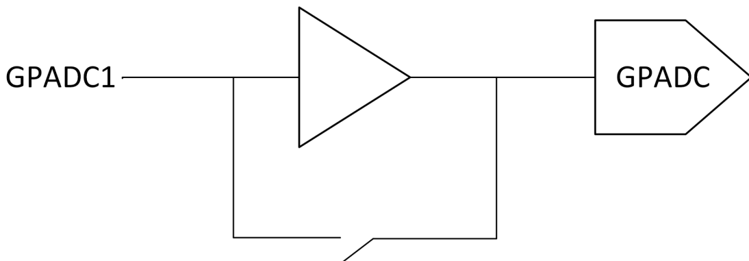
图 8-6. GPADC 路径
