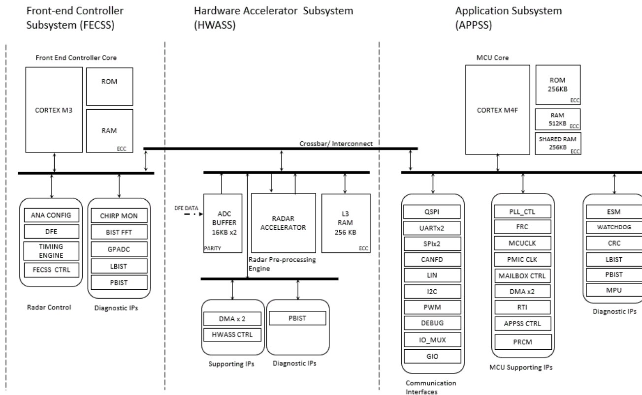
图 8-4. 处理器子系统
