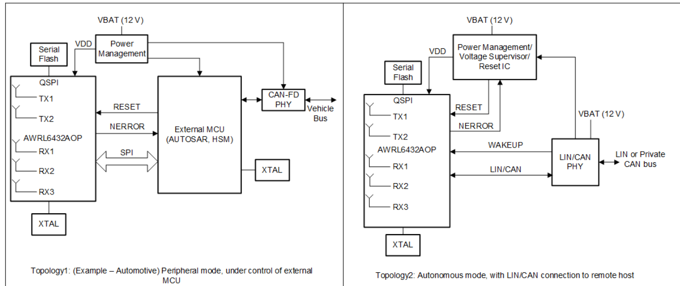
图 7-1. 系统拓扑
