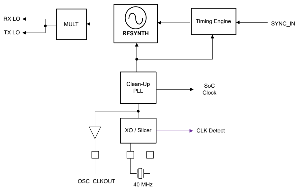
图 8-1. 时钟子系统
