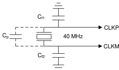
图 7-12. 晶体实现方式
