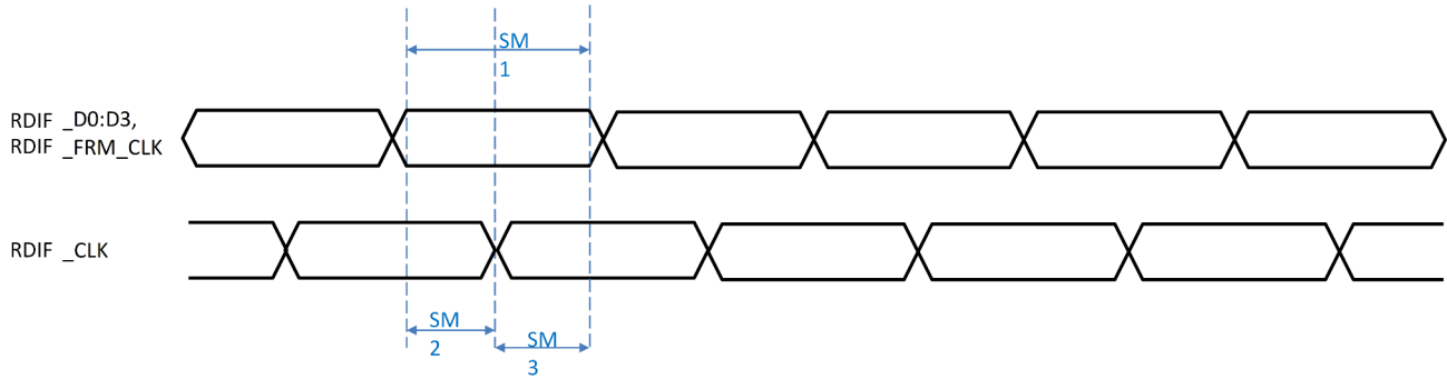
图 7-17. RDIF 时序要求
