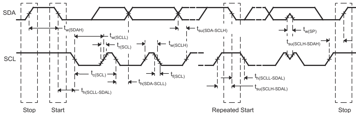
图 7-19. I2C 时序图
