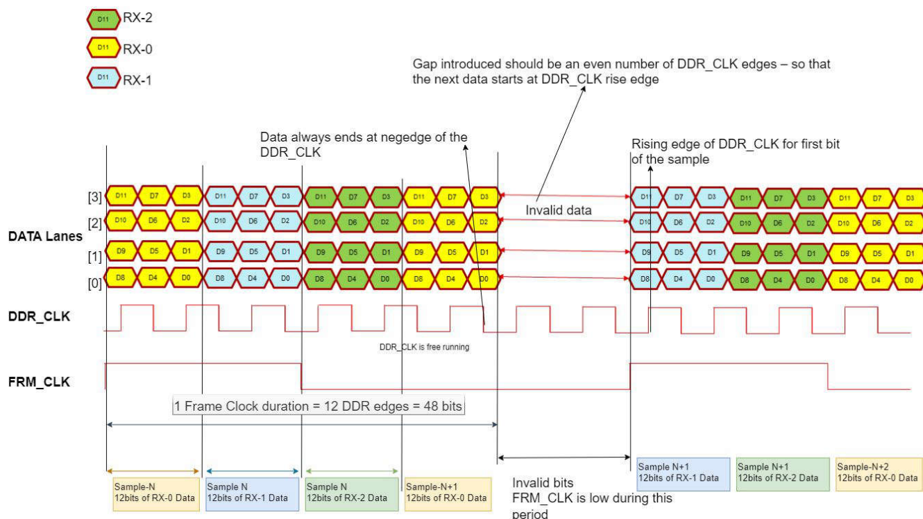
图 7-18. RDIF 数据格式
