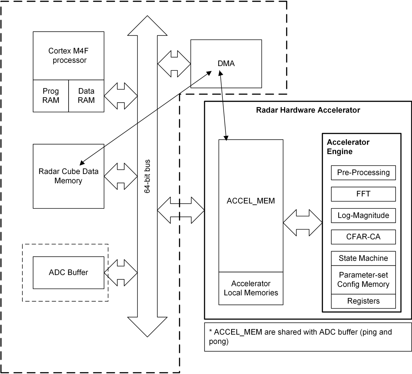
图 8-5. HWA 1.2 功能方框图
