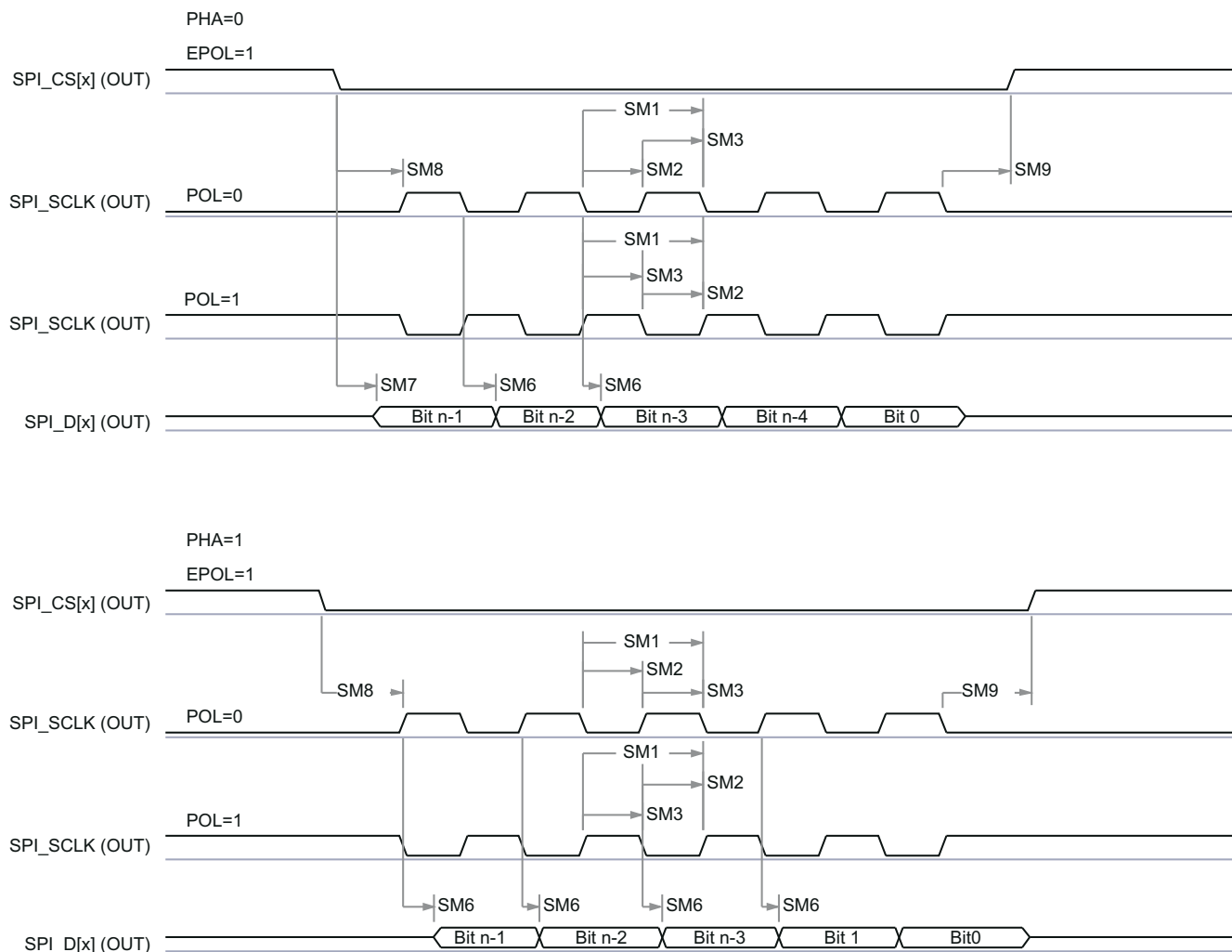
图 7-14. SPI 时序 — 控制器模式发送
