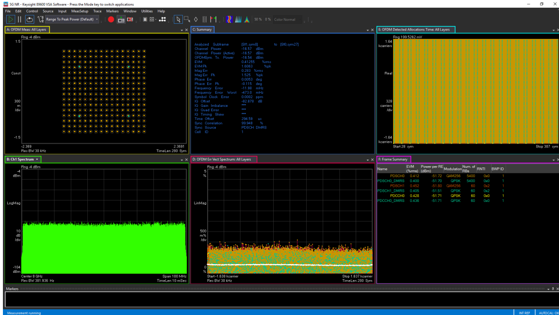
图 4-230. TX 100MHz NR EVM at 8.1GHz
