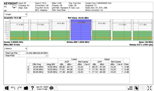
图 4-174. TX 20MHz LTE Output Spectrum at 4.9GHz
