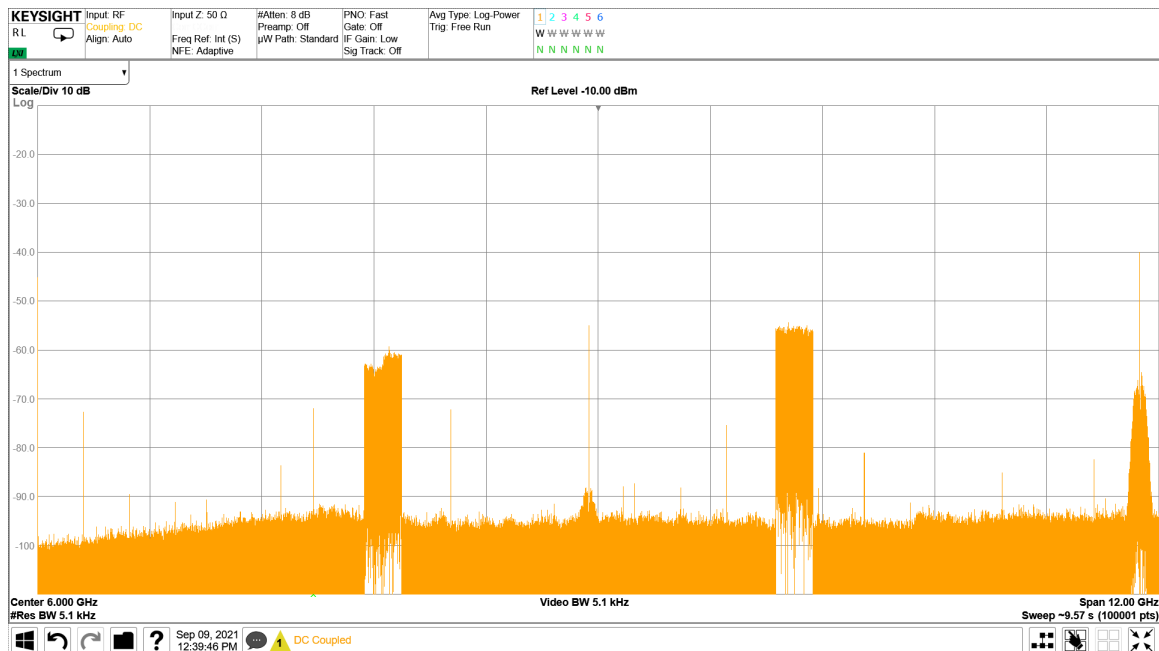
图 4-232. TX 4x100MHz NR Output Spectrum 8.1GHz
