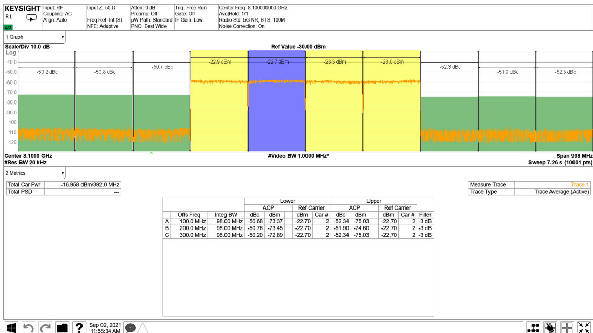
图 4-231. TX 4x100MHz NR Output Spectrum 8.1GHz
