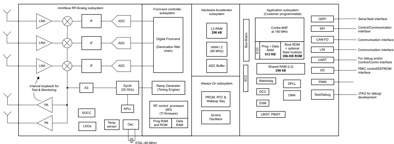
图 8-1. 功能方框图
