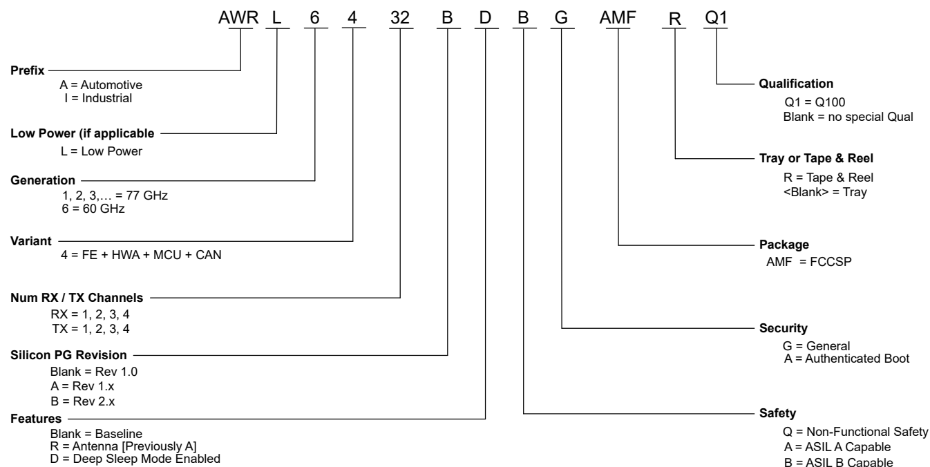
图 11-1. Device Nomenclature
