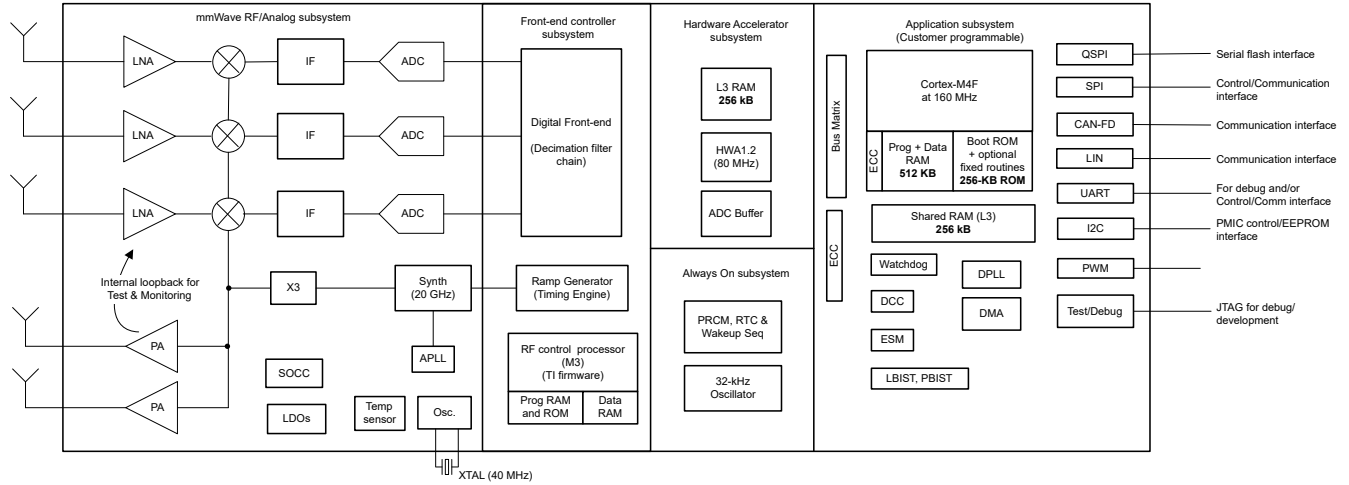
图 4-1. 功能方框图
