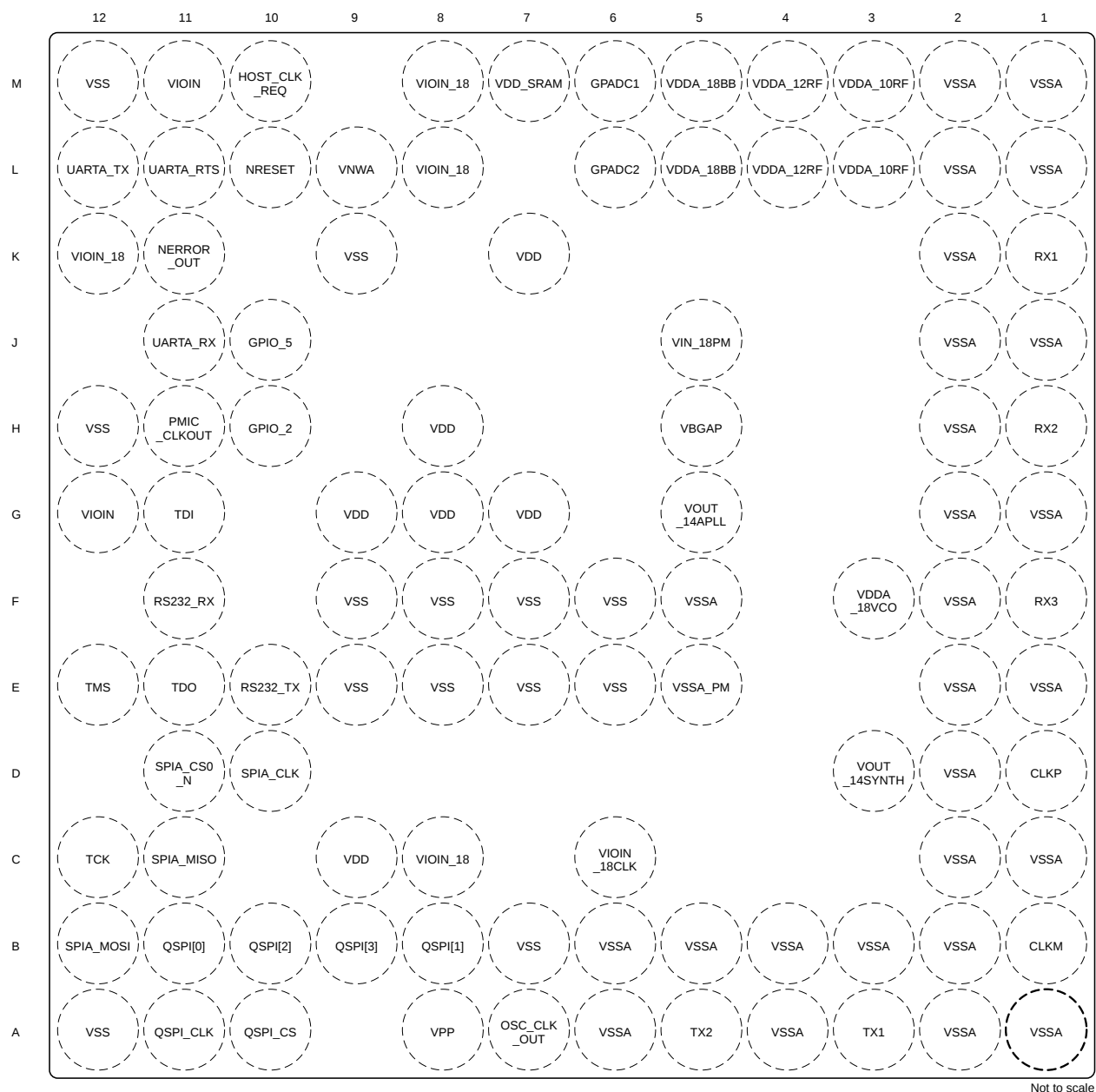
图 6-1. FCCSP Pin Diagram (Top View)
