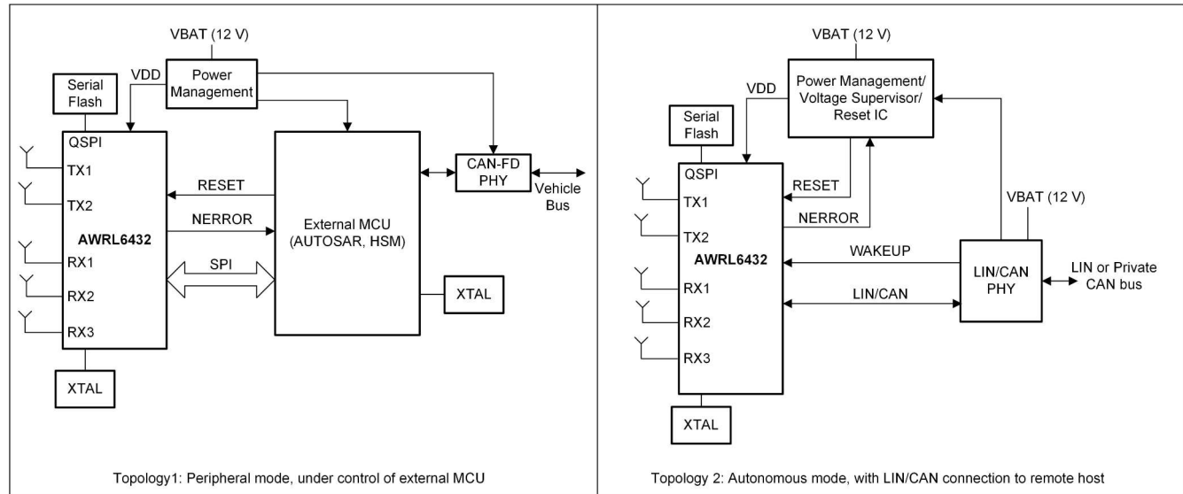
图 7-1. System Topologies
