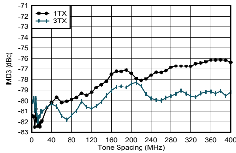
图 5-23. 0.85GHz 条件下 TX IMD3 与频率间隔和通道间的关系
