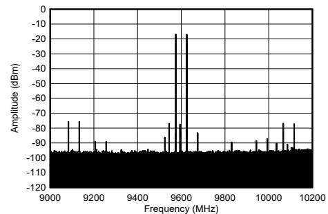
图 5-272. 9.61GHz 和 -7dBFS (1.2 GHz 带宽) 条件下 TX 双音频谱
