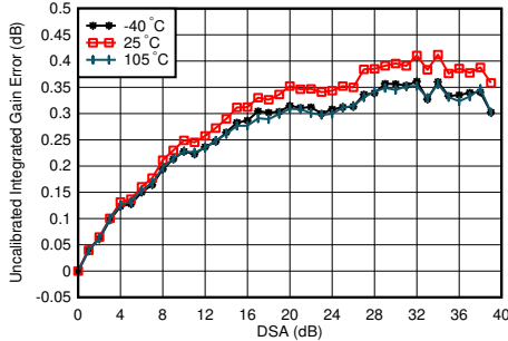
图 5-130. 3.5GHz 条件下 TX 未校准积分增益误差与 DSA 设置和温度间的关系
