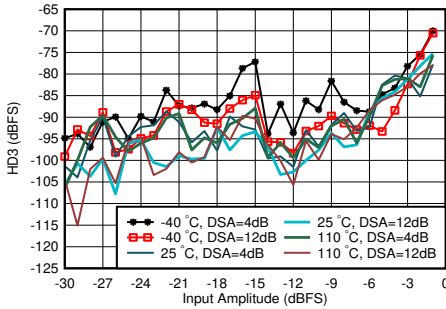
图 5-309. 800MHz 条件下 RX HD3 与 DSA 设置和温度间的关系
