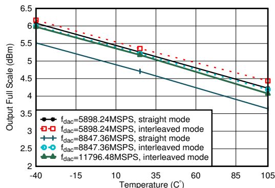
图 5-2. TX 输出满量程与温度间的关系
