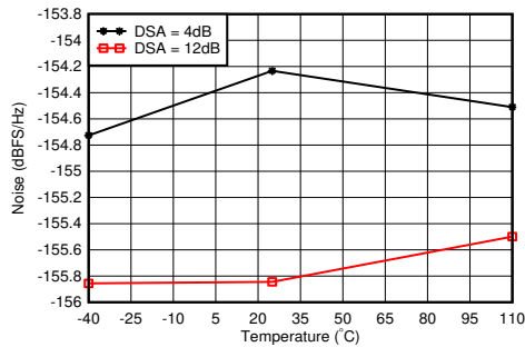
图 5-297. 0.8GHz 条件下 RX 噪声频谱密度与温度间的关系
