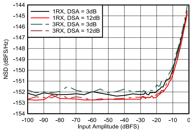
图 5-432. 8.1GHz 条件下 RX NSD 与数字振幅间的关系
