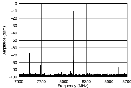
图 5-204. 8.1GHz 条件下 TX 单音输出频谱
