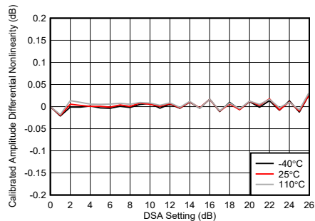
图 5-239. TX DSA 已校准振幅微分非线性
