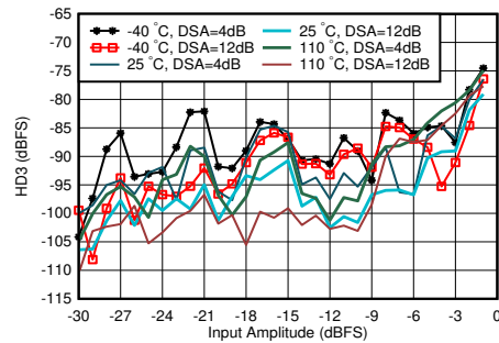
图 5-341. 1.9GHz 条件下 RX HD3 与输入电平和温度间的关系
