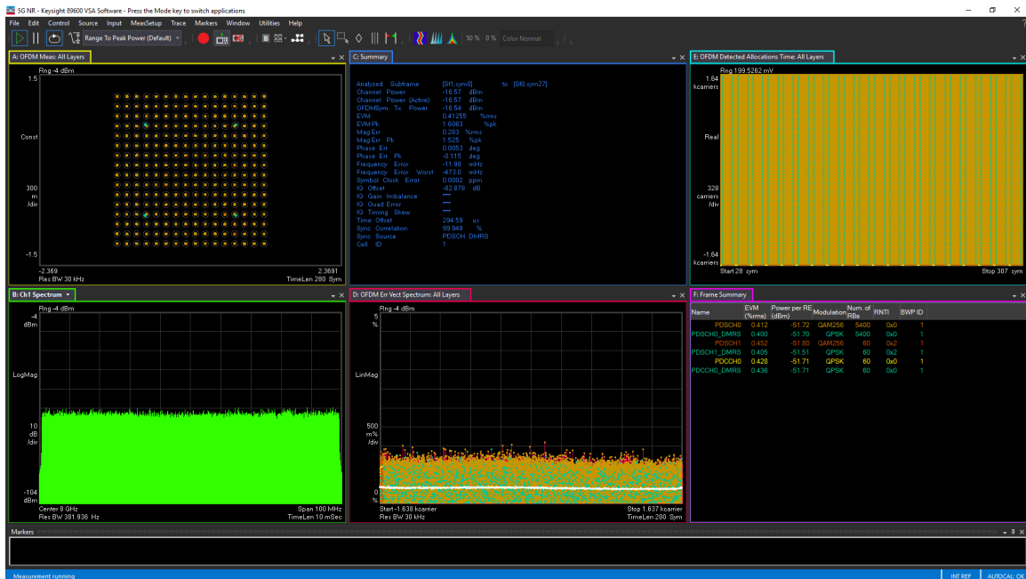
图 5-230. 8.1GHz 条件下 TX 100MHz NR EVM
