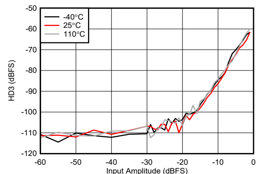
图 5-463. 9.6GHz 条件下 RX HD3 与数字电平间的关系
