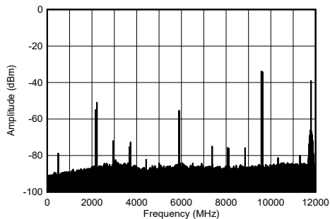
图 5-275. 9.61GHz 和单频 -30dBFS (宽带) 条件下 TX 双音频谱
