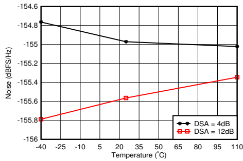
图 5-328. 1.75GHz 条件下 RX 噪声频谱密度与温度间的关系
