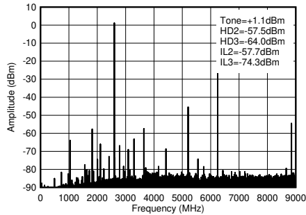
图 5-114. 2.6GHz (0 - f_{\text{DAC}} ) 条件下的 TX 单音 (-12dBFS) 输出频谱
