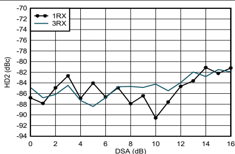
图 5-411. 4.9GHz 条件下 RX HD2 与 DSA 设置和通道间的关系
