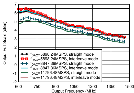
图 5-1. TX 输出满量程与输出频率间的关系
