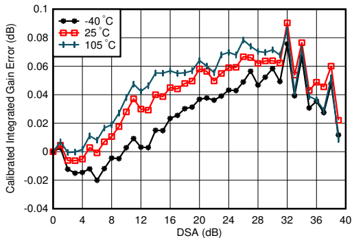
图 5-9. 0.85GHz 条件下 TX 校准差分增益误差与 DSA 设置和温度间的关系
