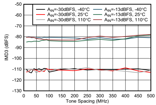
图 5-457. 9.6 GHz 条件下 RX IMD3 与频率间隔间的关系
