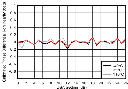
图 5-247. TX DSA 已校准相位微分非线性
