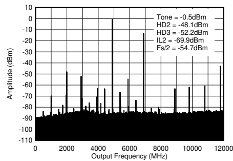
图 5-181. 4.9GHz (0 - f_{\text{DAC}} ) 条件下的 TX 单频 (-12dBFS) 输出频谱
