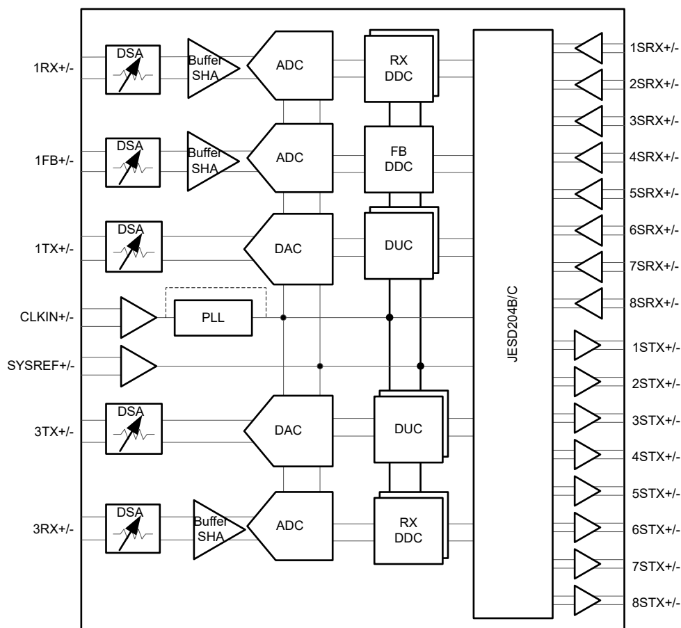
功能方框图
