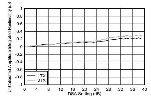
图 5-191. 8.11GHz 条件下 TX DSA 未校准振幅积分非线性
