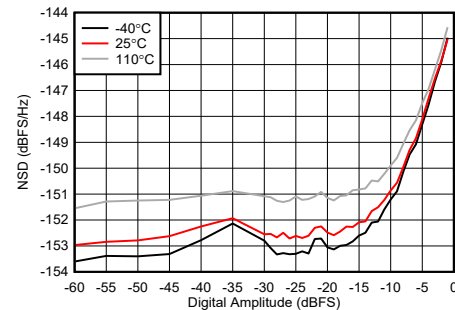
图 5-260. 9.61GHz 条件下 TX NSD 与数字振幅间的关系
