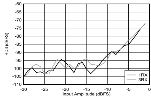
图 5-385. 3.6GHz 条件下 RX HD3 与输入电平和通道间的关系
