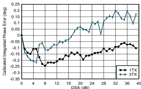
图 5-161. 4.9GHz 条件下 TX 校准差分相位误差与 DSA 设置和通道间的关系
