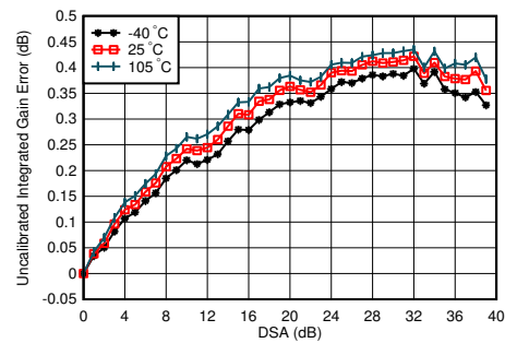
图 5-156. 4.9GHz 条件下 TX 未校准差分增益误差与 DSA 设置和温度间的关系
