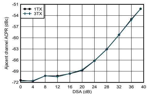
图 5-71. 1.8GHz 条件下 TX 20MHz LTE ACPR 与 DSA 间的关系
