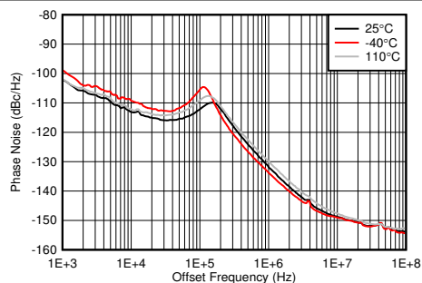
图 5-504. f_{OUT} = 1910\text{MHz} 时 8GHz VCO 相位噪声与偏移频率和温度间的关系
