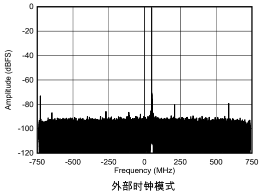
图 5-440. 8.1GHz 条件下 RX 单频输出 FFT，-1dBFS
