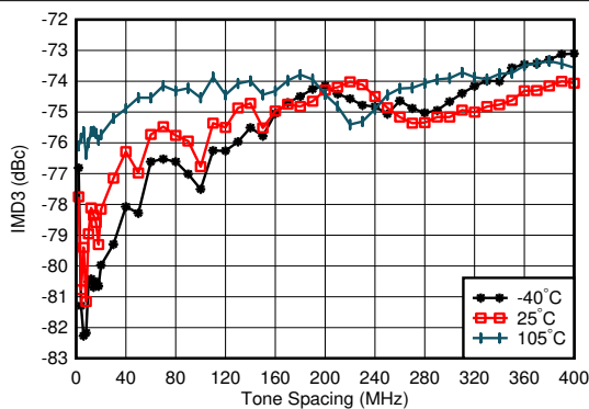
图 5-25. 0.85GHz 条件下 TX IMD3 与频率间隔和温度间的关系
