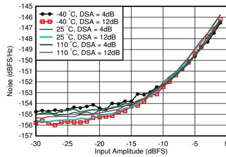
图 5-329. 1.75GHz 条件下 RX 噪声频谱密度与输入振幅和温度间的关系
