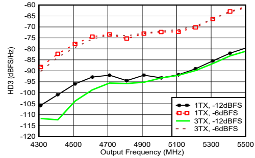
图 5-180. 4.9GHz 条件下 TX HD3 与数字振幅和输出频率间的关系
