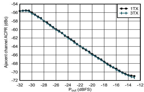
图 5-69. 1.8425GHz 条件下 TX 20MHz LTE ACPR 与数字电平间的关系
