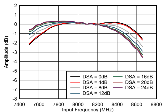
图 5-423. RX 振幅与频率和 DSA 设置间的关系
