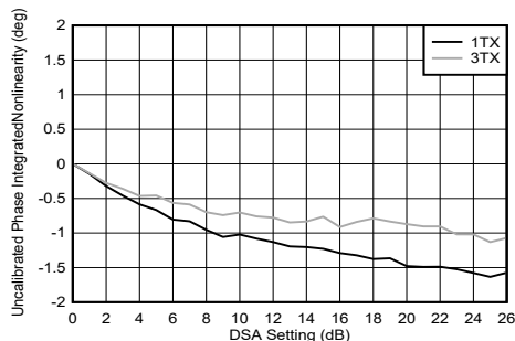
图 5-248. TX DSA 未校准相位积分非线性
