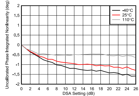
图 5-250. TX DSA 未校准相位积分非线性
