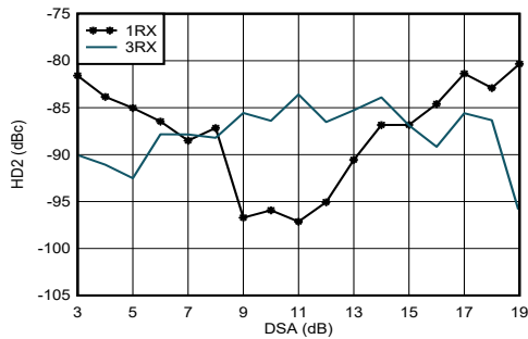
图 5-334. 1.9GHz 条件下 RX HD2 与 DSA 设置和通道间的关系
