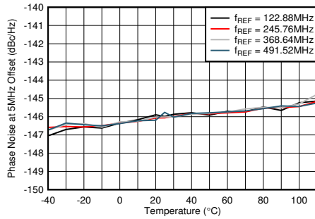
图 5-486. f_{OUT} = 2.6\text{GHz} 时 12GHz VCO 相位噪声 (5MHz 偏移条件下) 与温度和 f_{REF} 间的关系
