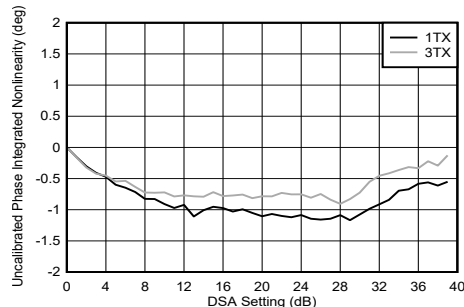
图 5-199. 8.1GHz 条件下 TX DSA 未校准相位积分非线性
