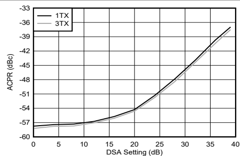
图 5-226. 8.11GHz 条件下 TX NR100MHz ACPR 与 DSA 设置间的关系
