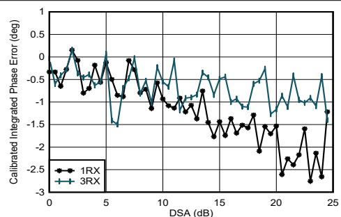
图 5-401. 4.9GHz 条件下 RX 校准差分相位误差与 DSA 设置间的关系
