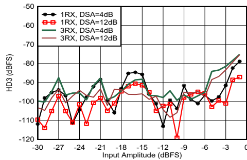
图 5-340. 1.9GHz 条件下 RX HD3 与输入电平和通道间的关系
