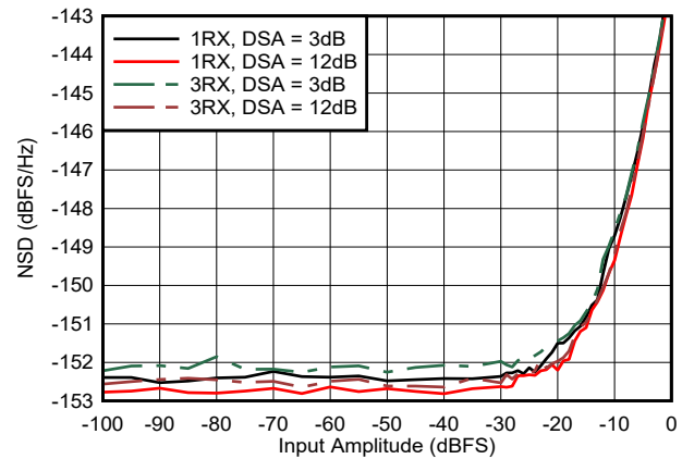
图 5-459. 9.6GHz 条件下 RX NSD 与数字振幅间的关系
