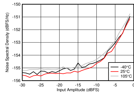
图 5-351. 2.6GHz 条件下 RX 噪声频谱密度与输入振幅和温度间的关系
