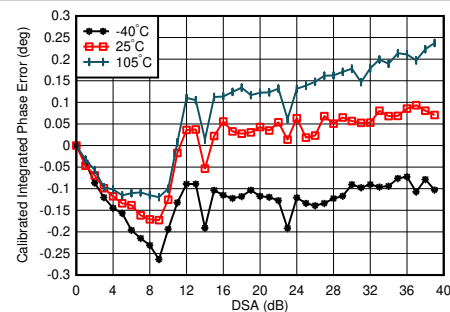
图 5-93. 2.6GHz 条件下 TX 校准差分相位误差与 DSA 设置和温度间的关系
