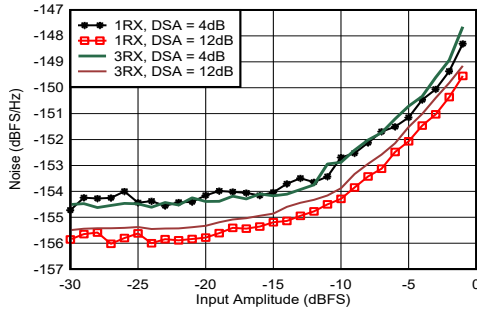
图 5-299. 0.8GHz 条件下 RX 噪声频谱密度与输入振幅和通道间的关系
