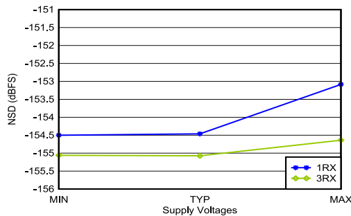
图 5-420. 4.9GHz 条件下 RX IMD3 与电源和通道间的关系
