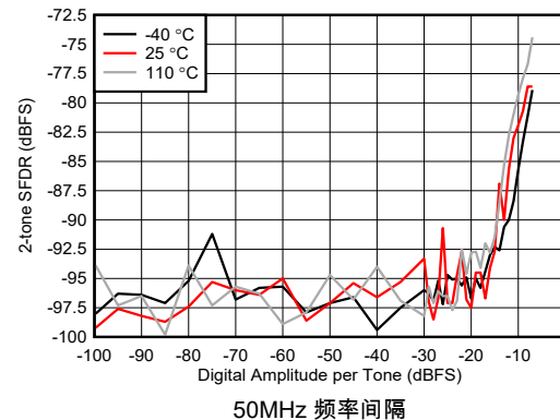
图 5-439. 8.1GHz 条件下 RX 双音 SFDR 与数字振幅间的关系
