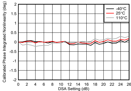
图 5-251. TX DSA 已校准振幅积分非线性
