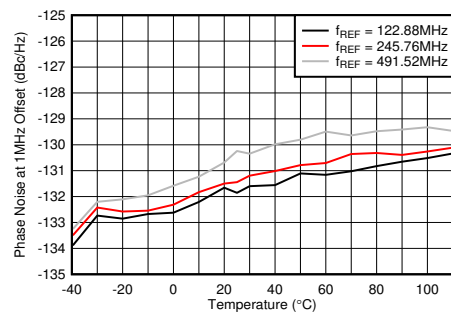
图 5-495. f_{OUT} = 2.6\text{GHz} 时 10GHz VCO 相位噪声 (1MHz 条件下) 与温度和 f_{REF} 间的关系
