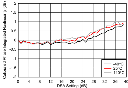
图 5-202. 8.1GHz 条件下 TX DSA 已校准相位积分非线性
