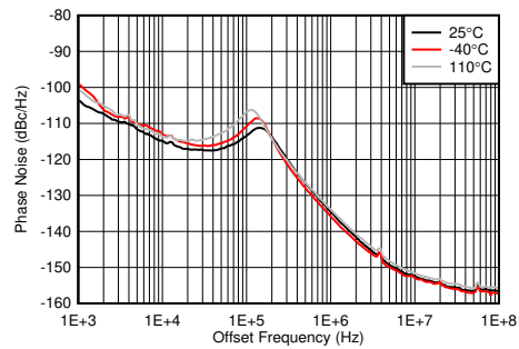
图 5-474. 12GHz 条件下 PLL 和外部时钟的相位噪声与偏移频率间的关系
