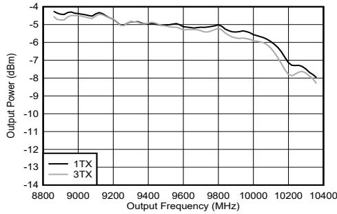
图 5-233. 9.61GHz 条件下 TX 输出功率与频率间的关系
