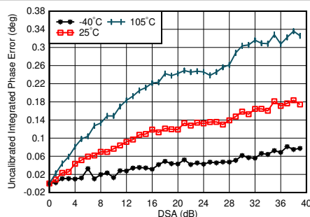
图 5-58. 1.8 GHz 条件下 TX 未校准差分相位误差与 DSA 设置和温度间的关系
