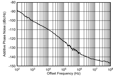
图 5-279. 9.61GHz 条件下 TX 附加相位噪声与偏移频率间的关系
