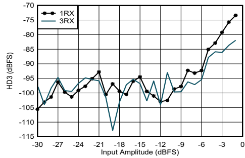
图 5-310. 800MHz 条件下 RX HD3 与输入电平和通道间的关系
