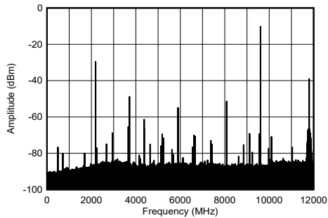
图 5-265. 9.61GHz 和 -1dBFS (宽带) 条件下 TX 单音频谱
