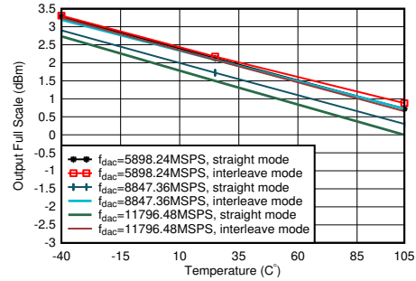
图 5-45. 1.8GHz 条件下 TX 输出功率与温度间的关系
