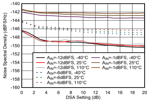
图 5-460. 9.6 GHz 条件下 RX NSD 与 DSA 设置间的关系
