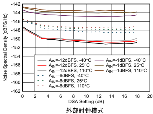
图 5-434. 8.1GHz 条件下 RX NSD 与 DSA 设置间的关系
