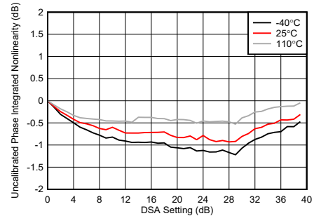
图 5-201. 8.1GHz 条件下 TX DSA 未校准相位积分非线性
