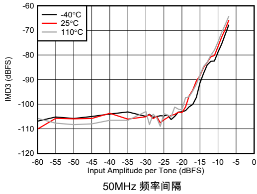
图 5-428. 8.1GHz 条件下 RX IMD3 与输入振幅间的关系
