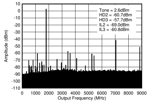
图 5-75. 1.8GHz ( 0 - f_{\text{DAC}} ) 条件下的 TX 单音 (-12dBFS) 输出频谱
