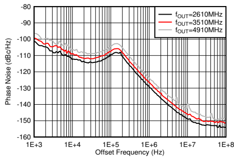
图 5-500. 25°C 条件下 9GHz VCO 相位噪声与偏移频率和 f_{OUT} 间的关系
