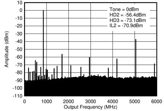
图 5-42. 0.85GHz (0- f_{\text{DAC}} ) 条件下的 TX 单频 (-6dBFS) 输出频谱
