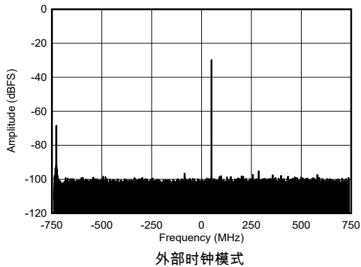
图 5-442. 8.1GHz 条件下 RX 单频输出 FFT，-30dBFS
