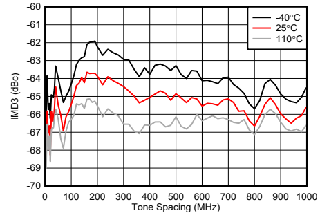
图 5-258. 9.61GHz 条件下 TX IMD3 与频率间隔间的关系
