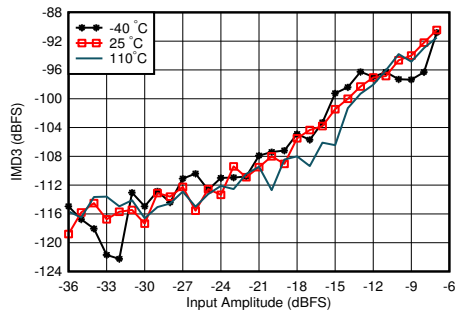
图 5-332. 1.75GHz 条件下 RX IMD3 与输入电平和温度间的关系
