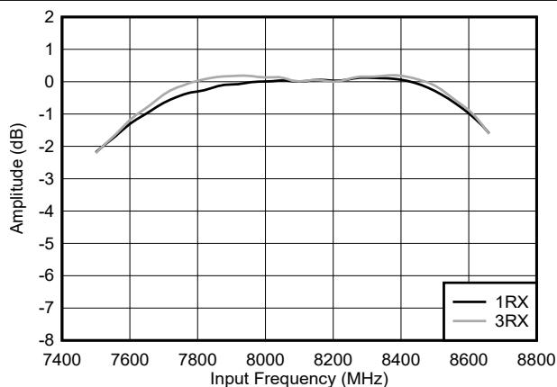
图 5-422. RX 振幅与频率和通道间的关系
