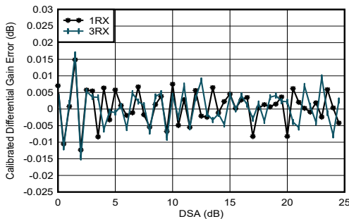
图 5-397. 4.9GHz 条件下 RX 校准差分振幅误差与 DSA 设置间的关系
