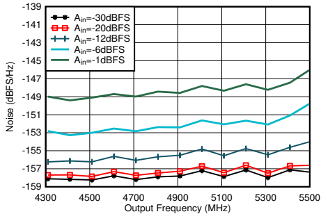
图 5-173. 4.9 GHz 条件下 TX 单频输出噪声与频率和振幅间的关系
