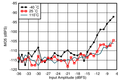
图 5-304. 0.8GHz 条件下 Rx IMD5 与输入电平和温度间的关系
