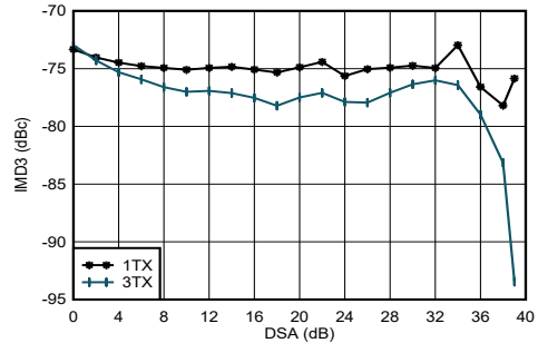
图 5-97. 2.6GHz 条件下 TX IMD3 与 DSA 设置间的关系
