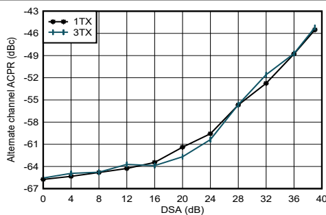
图 5-227. 8.11GHz 条件下 TX NR100MHz alt-ACPR 与 DSA 设置间的关系
