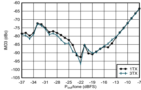
图 5-30. 0.85GHz 条件下 TX IMD3 与数字电平间的关系
