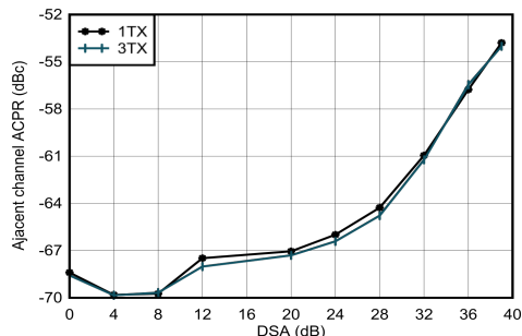
图 5-35. 0.85GHz 条件下 TX 20MHz LTE ACPR 与 DSA 间的关系
