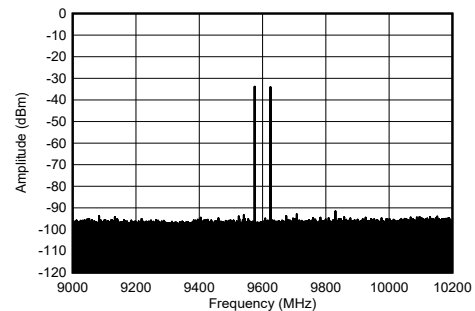
图 5-276. 9.61GHz 和单频 -30dBFS (1.2GHz 带宽) 条件下 TX 双音频谱
