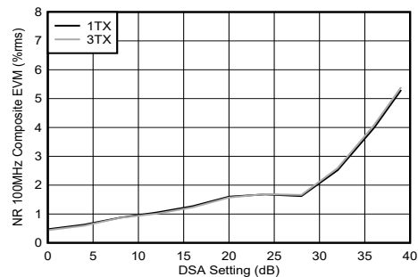
图 5-282. 9.61GHz 条件下 TX NR100MHz EVM 与 DSA 设置间的关系
