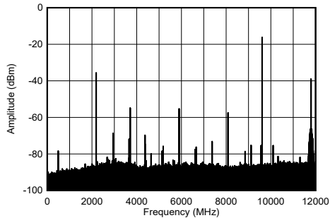
图 5-267. 9.61GHz 和 -6dBFS (宽带) 条件下 TX 单音频谱
