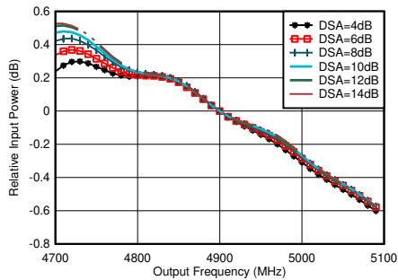
图 5-393. RX 带内增益平坦度， f_{\text{IN}} = 4900\text{MHz}
