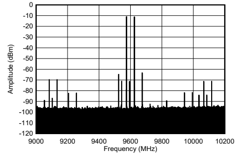
图 5-272. 9.61GHz 和 -7dBFS (1.2 GHz 带宽) 条件下 TX 双音频谱
