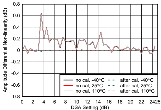
图 5-450. 9.6GHz 条件下 RX 振幅微分非线性
