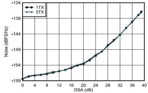
图 5-20. 0.85GHz 条件下 TX 输出噪声与通道和衰减间的关系
