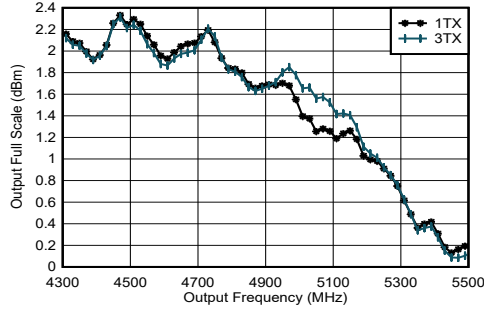
图 5-149. 11796.48MSPS 条件下的 TX 满量程与射频频率和通道间的关系
