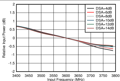
图 5-366. RX 带内增益平坦度， f_{\text{IN}} = 3600\text{MHz}
