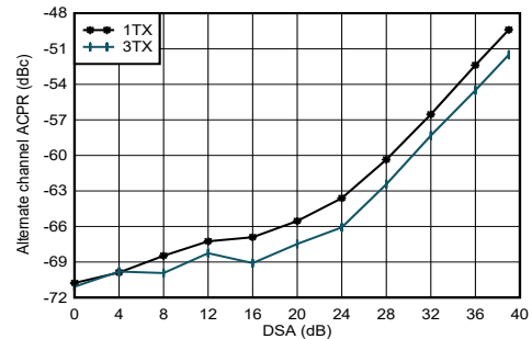
图 5-176. 4.9GHz 条件下 TX 20MHz LTE alt-ACPR 与数字电平间的关系
