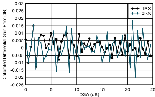
图 5-289. 0.8GHz 条件下 RX 校准差分振幅误差与 DSA 设置间的关系
