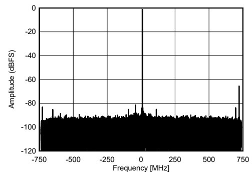
图 5-465. 9.61GHz 条件下 RX 单音输出 FFT
