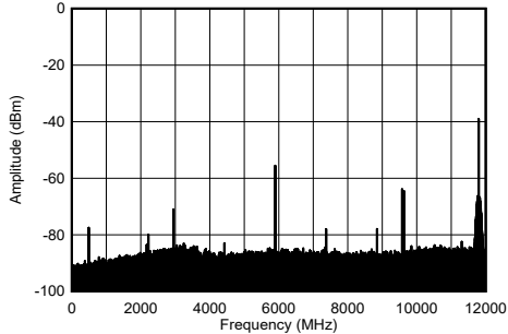
图 5-277. 9.61GHz 和单频 -60dBFS (宽带) 条件下 TX 双频频谱
