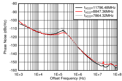
图 5-475. f_{\text{OUT}} = 2610\text{MHz} 时相位噪声与偏移频率和 f_{\text{VCO}} 间的关系
