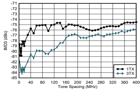
图 5-24. 0.85GHz 条件下 TX IMD3 与频率间隔和通道间的关系
