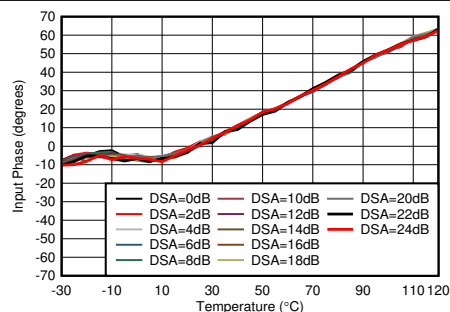
图 5-367. 3.6GHz 条件下 RX 输入相位与温度间的关系
