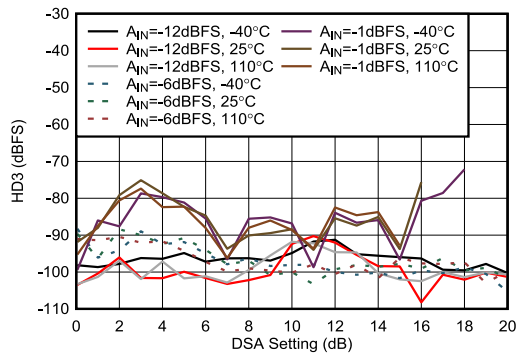
图 5-438. 8.1GHz 条件下 RX HD3 与 DSA 设置间的关系
