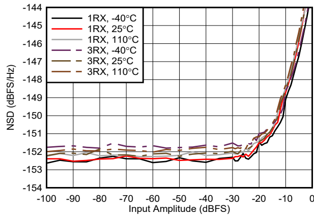
图 5-458. 9.6GHz 条件下 RX NSD 与数字振幅间的关系
