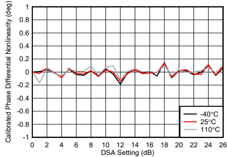
图 5-249. TX DSA 已校准相位积分非线性
