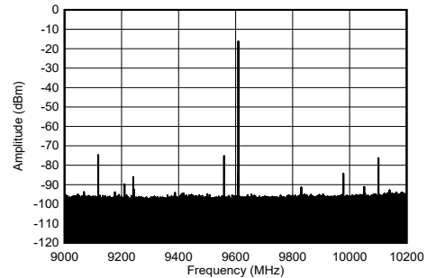
图 5-268. 9.61GHz 和 -6dBFS (1.2 GHz 带宽) 条件下 TX 单音频谱
