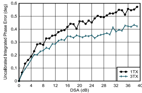
图 5-126. 3.5GHz 条件下 TX 未校准积分相位误差与 DSA 设置和通道间的关系
