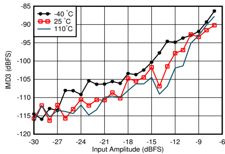
图 5-303. 0.8GHz 条件下 RX IMD3 与输入电平和温度间的关系
