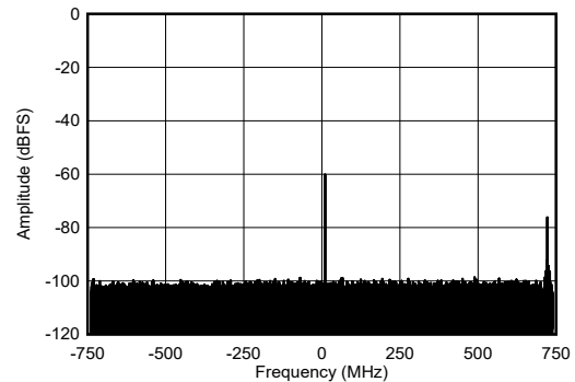
图 5-467. 9.61GHz 条件下 RX 单音输出 FFT
