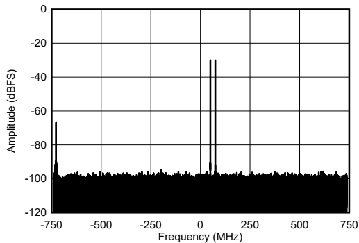
外部时钟模式，单频幅度为 -30dBFS 图 5-446. 8.1GHz 条件下 RX 双音输出 FFT
