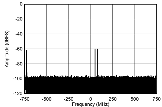
外部时钟模式，单频幅度为 -60dBFS 图 5-447. 8.1GHz 条件下 RX 双音输出 FFT
