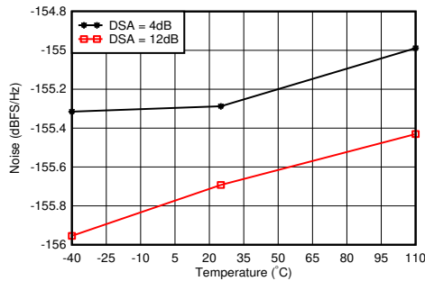
图 5-405. 4.9GHz 条件下 RX 噪声频谱密度与温度间的关系
