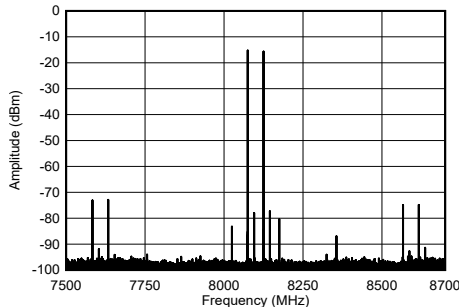
图 5-210. 8.1GHz 条件下 TX 双音输出频谱
