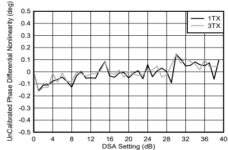
图 5-195. 8.1GHz 条件下 TX DSA 未校准相位微分非线性
