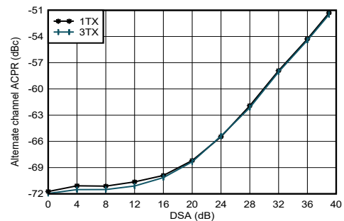
图 5-105. 2.6GHz 条件下 TX 20MHz LTE alt-ACPR 与数字电平间的关系
