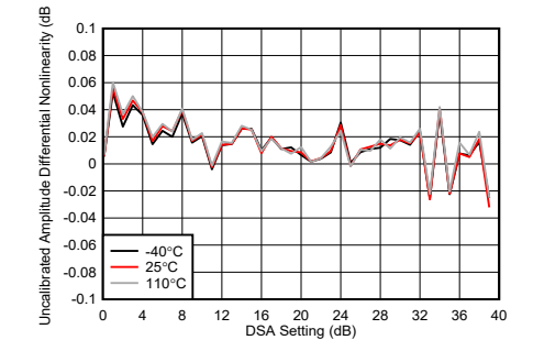
图 5-189. 8.11GHz 条件下 TX DSA 未校准振幅微分非线性
