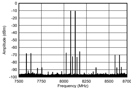
图 5-208. 8.1GHz 条件下 TX 单音输出频谱
