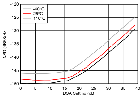
图 5-263. 9.61 GHz 条件下 TX NSD 与 DSA 设置间的关系
