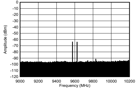
图 5-278. 9.61GHz 和单频 -60dBFS (1.2GHz 带宽) 条件下 TX 双频频谱
