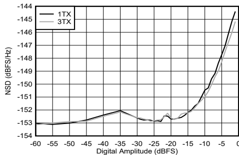
图 5-259. 9.61GHz 条件下 TX NSD 与数字振幅间的关系
