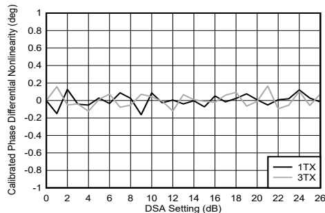
图 5-245. TX DSA 已校准相位微分非线性
