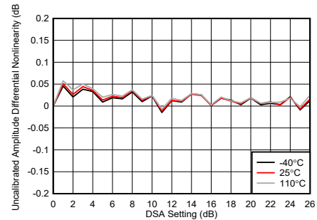
图 5-238. TX DSA 未校准振幅微分非线性
