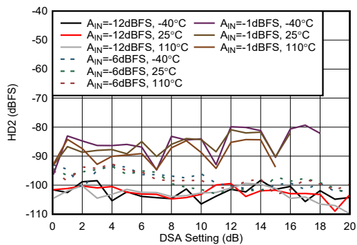
图 5-436. 8.1GHz 条件下 RX HD2 与 DSA 设置间的关系
