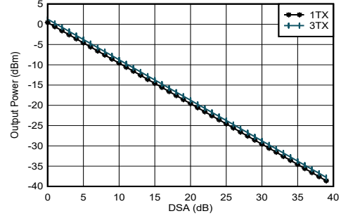
图 5-119. 3.5GHz 条件下 TX 输出功率与 DSA 设置间的关系
