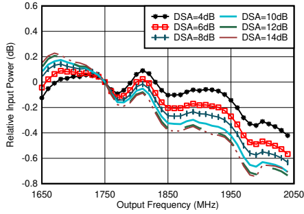
图 5-316. RX 带内增益平坦度， f_{\text{IN}} = 1750\text{MHz}
