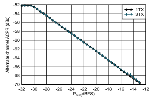
图 5-34. 0.85GHz 条件下 TX 20MHz LTE alt-ACPR 与数字电平间的关系
