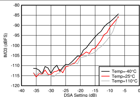
图 5-378. 3.6GHz 条件下 RX IMD3 与输入电平和温度间的关系
