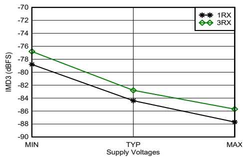
使用 3.6GHz 匹配时，单音幅度为 -7dBFS，频率间隔为 20MHz，所有电源均处于 MIN、TYP 或 MAX 推荐工作电压 图 5-390. 3.6GHz 条件下 RX IMD3 与电源电压和通道间的关系
