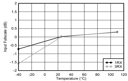
图 5-347. 2.6GHz 条件下 RX 输入满量程与温度和通道间的关系
