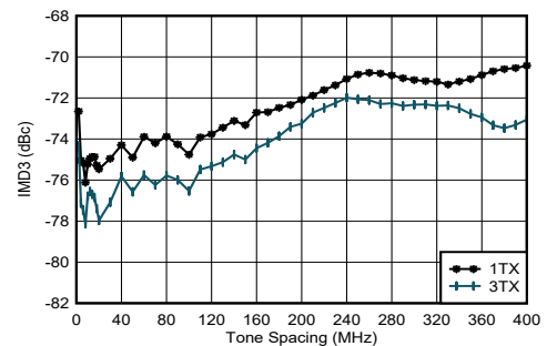
图 5-22. 0.85GHz 条件下 TX IMD3 与频率间隔和通道间的关系
