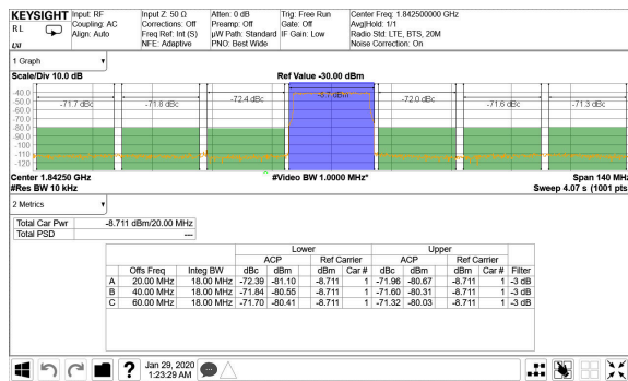
图 5-68. 1.8425GHz 条件下的 TX 20MHz LTE 输出频谱
