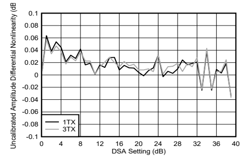
图 5-187. 8.11GHz 条件下 TX DSA 未校准振幅微分非线性
