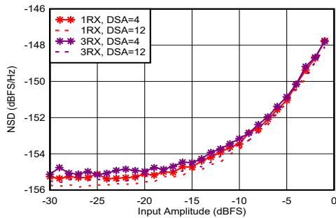
图 5-352. 2.6GHz 条件下 RX 噪声频谱密度与输入振幅和通道间的关系
