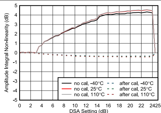
图 5-425. 8.1GHz 条件下 RX 振幅积分非线性
