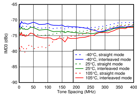
图 5-99. 2.6GHz 条件下 TX IMD3 与频率间隔和温度间的关系
