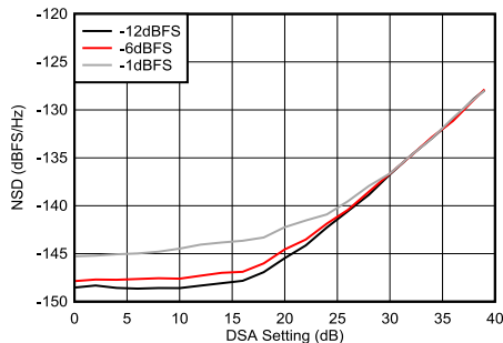
图 5-261. 9.61 GHz 条件下 TX NSD 与 DSA 设置间的关系
