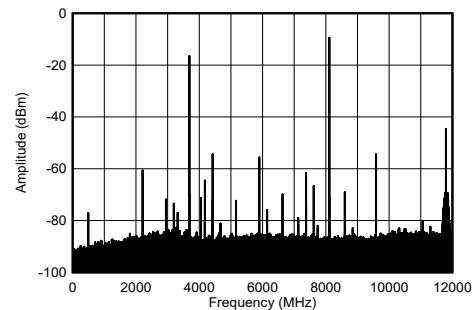
图 5-203. 8.1GHz 条件下 TX 单音输出频谱
