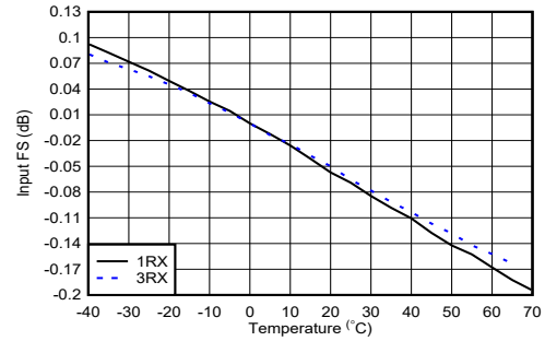
图 5-286. 800MHz 条件下 RX 输入满量程与温度和通道间的关系
