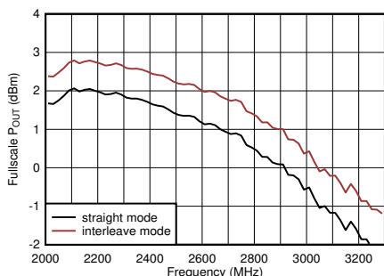
图 5-78. 11796.48MSPS 条件下 TX 满量程与射频频率间的关系
