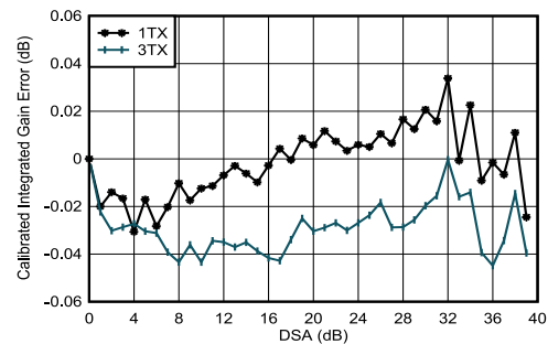
图 5-47. 1.8 GHz 条件下 TX 校准差分增益误差与 DSA 设置和通道间的关系
