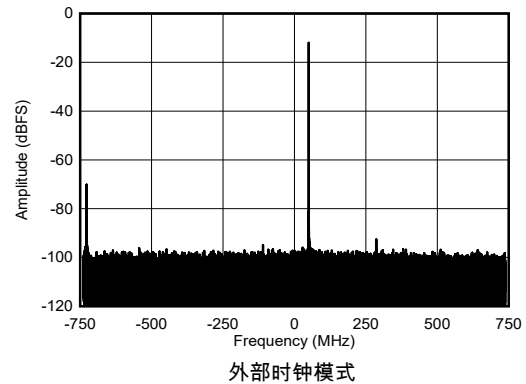
图 5-441. 8.1GHz 条件下 RX 单频输出 FFT，-12dBFS
