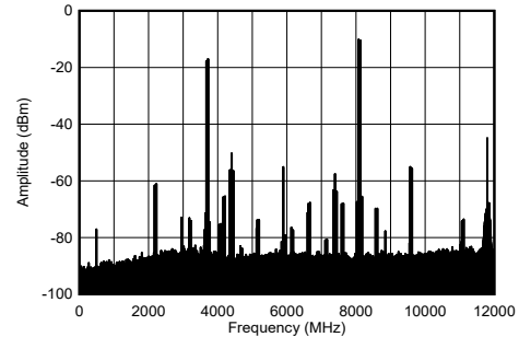
图 5-209. 8.1GHz 条件下 TX 双音输出频谱
