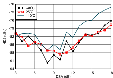
图 5-412. 4.9GHz 条件下 RX HD2 与 DSA 和温度间的关系
