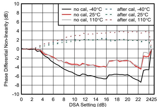
图 5-427. 8.1GHz 条件下 RX 相位积分非线性
