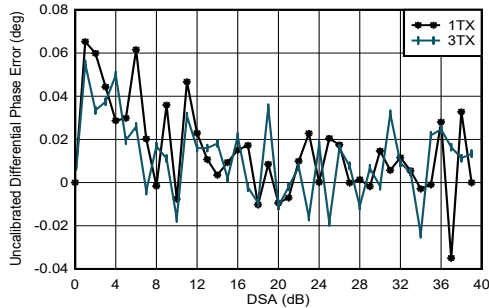
图 5-124. 3.5GHz 条件下 TX 未校准差分相位误差与 DSA 设置和通道间的关系
