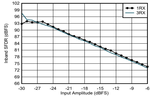
图 5-418. 4.9GHz 条件下 RX 带内 SFDR ( \pm 400\text{MHz} ) 与输入振幅和通道间的关系
