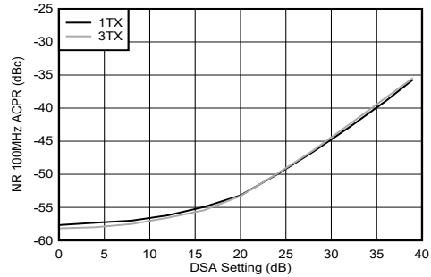
图 5-280. 9.61GHz 条件下 TX NR100 MHz ACPR 与 DSA 设置间的关系
