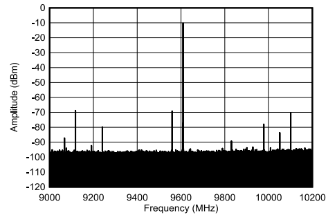
图 5-266. 9.61GHz 和 -1dBFS (1.2 GHz 带宽) 条件下 TX 单音频谱
