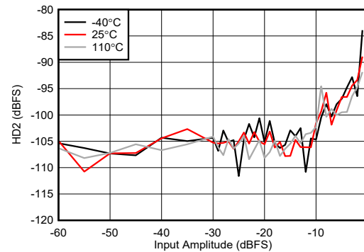
图 5-435. 8.1GHz 条件下 RX HD2 与数字振幅间的关系
