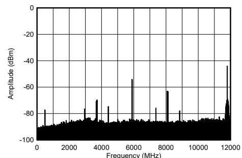
图 5-213. 8.1GHz 条件下 TX 双音输出频谱
