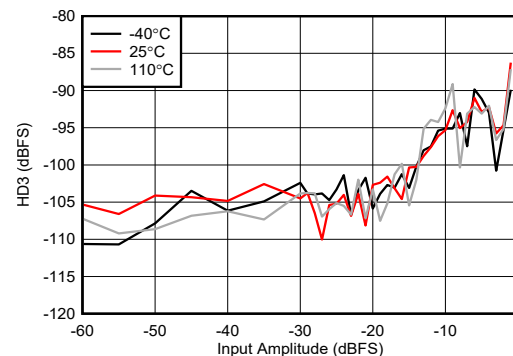
图 5-437. 8.1GHz 条件下 RX HD3 与数字振幅间的关系
