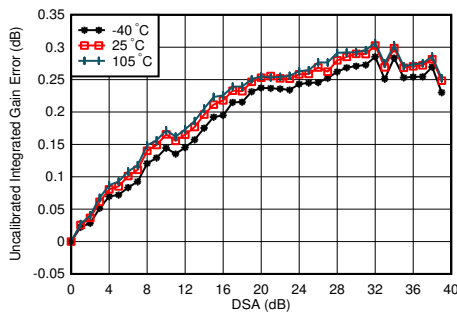
图 5-50. 1.8 GHz 条件下 TX 未校准差分增益误差与 DSA 设置和温度间的关系
