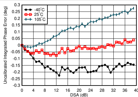
图 5-92. 2.6GHz 条件下 TX 未校准差分相位误差与 DSA 设置和温度间的关系
