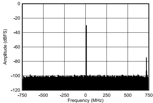
图 5-468. 9.61GHz 条件下 RX 单音输出 FFT
