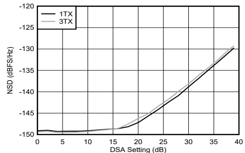
图 5-262. 9.61 GHz 条件下 TX NSD 与 DSA 设置间的关系
