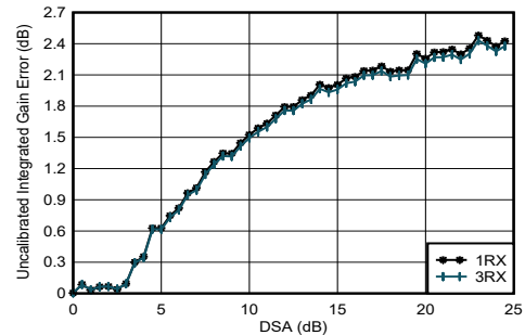
图 5-288. 0.8GHz 条件下 RX 未校准差分振幅误差与 DSA 设置间的关系
