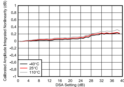
图 5-194. 8.1GHz 条件下 TX DSA 已校准振幅积分非线性
