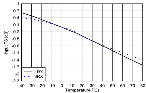
图 5-394. 4.9GHz 条件下 RX 输入满量程与温度和通道间的关系
