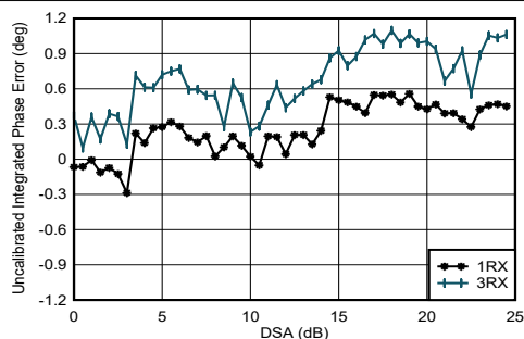
图 5-292. 0.8GHz 条件下 RX 未校准差分相位误差与 DSA 设置间的关系
