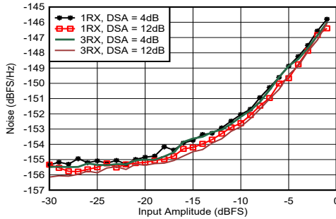
图 5-407. 4.9GHz 条件下 RX 噪声频谱密度与输入振幅和通道间的关系
