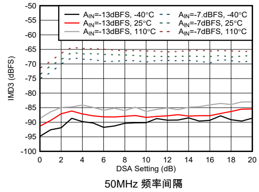
图 5-429. 8.1GHz 条件下 RX IMD3 与 DSA 设置间的关系
