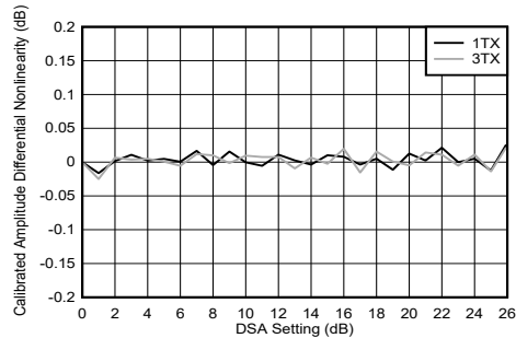
图 5-237. TX DSA 已校准振幅微分非线性
