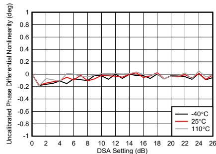
图 5-246. TX DSA 未校准相位微分非线性
