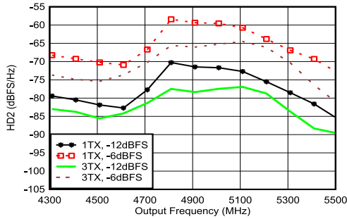
图 5-179. 4.9GHz 条件下 TX HD2 与数字振幅和输出频率间的关系
