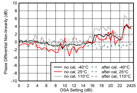
图 5-453. 9.6GHz 条件下 RX 相位微分非线性
