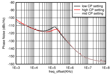
图 5-480. f_{OUT} = 2.6\text{GHz} 时 12GHz VCO 相位噪声与偏移频率和 CP 设置间的关系
