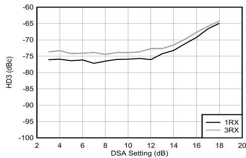
图 5-358. 2.6GHz 条件下 RX HD3 与 DSA 设置和通道间的关系
