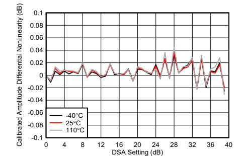
图 5-190. 8.11GHz 条件下 TX DSA 已校准振幅微分非线性
