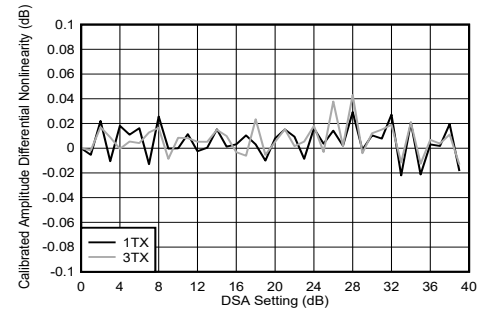
图 5-188. 8.11GHz 条件下 TX DSA 已校准振幅微分非线性
