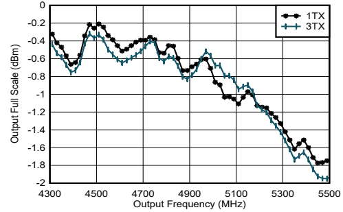
图 5-150. 5898.24MSPS、直接模式、第二奈奎斯特区域条件下的 TX 满量程与射频频率和通道间的关系
