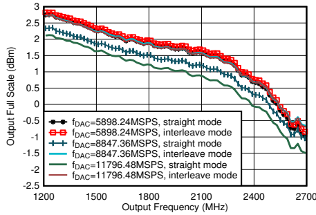
图 5-44. TX 输出满量程与输出频率间的关系
