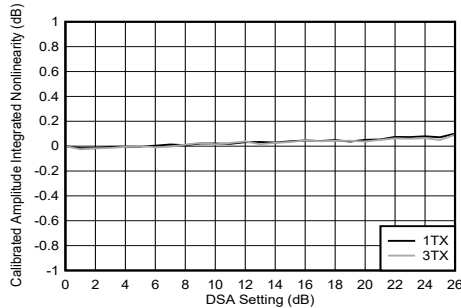
图 5-241. TX DSA 已校准振幅积分非线性
