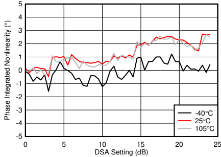
图 5-372. 3.6GHz 条件下 RX 未校准相位误差与 DSA 设置间的关系
