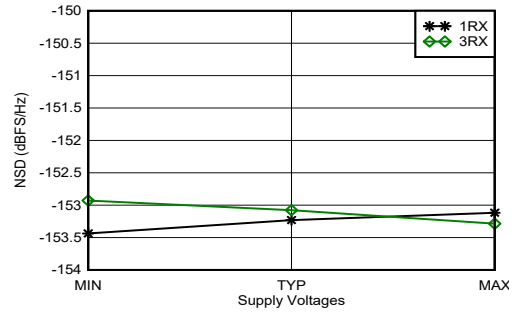
图 5-365. 2.6GHz 条件下 RX 噪声频谱密度与电源和通道间的关系
