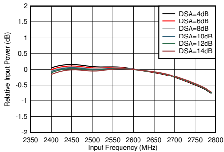
图 5-346. RX 带内增益平坦度， f_{\text{IN}} = 2600\text{MHz}
