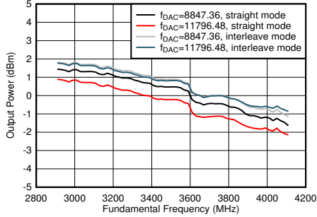
图 5-118. TX 输出功率与频率间的关系
