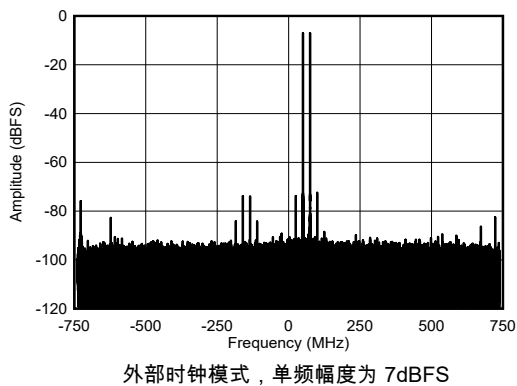
图 5-444. 8.1GHz 条件下 RX 双音输出 FFT
