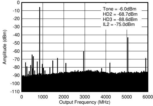
图 5-41. 0.85GHz (0- f_{\text{DAC}} ) 条件下的 TX 单音 (-12dBFS) 输出频谱
