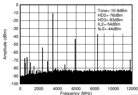
图 5-148. 3.5GHz (0 - f_{\text{DAC}} ) 条件下的 TX 单音 (-12dBFS) 输出频谱
