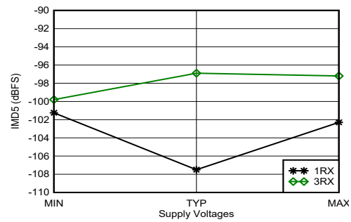
使用 3.6GHz 匹配时，单音幅度为 -7dBFS，频率间隔为 20MHz，所有电源均处于 MIN、TYP 或 MAX 推荐工作电压 图 5-391. 3.6GHz 条件下 RX IMD5 与电源电压和通道间的关系
