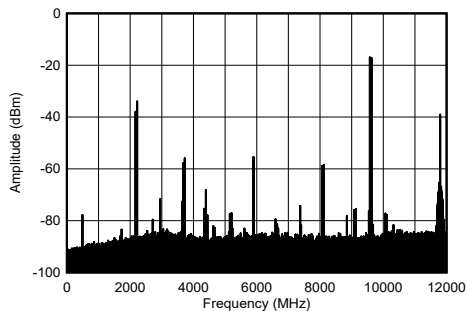
图 5-271. 9.61GHz 和 -7dBFS (宽带) 条件下 TX 双音频谱
