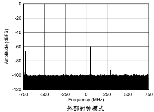
图 5-443. 8.1GHz 条件下 RX 单频输出 FFT，-60dBFS
