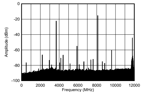
图 5-205. 8.1GHz 条件下 TX 单音输出频谱
