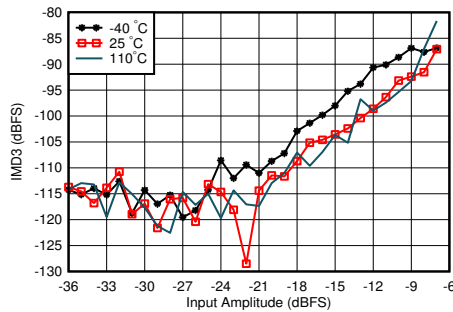
图 5-409. 4.9GHz 条件下 RX IMD3 与输入电平和温度间的关系
