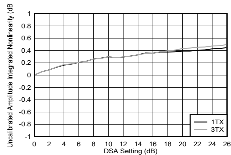
图 5-240. TX DSA 未校准振幅积分非线性
