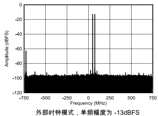
图 5-445. 8.1GHz 条件下 RX 双音输出 FFT
