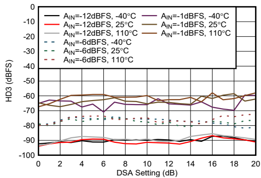
图 5-464. 9.6 GHz 条件下 RX HD3 与 DSA 设置间的关系
