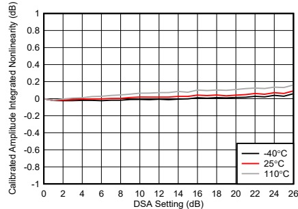
图 5-243. TX DSA 已校准振幅积分非线性
