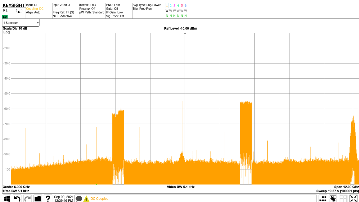
图 5-232. 8.11GHz 条件下 TX 4x100MHz NR 输出频谱
