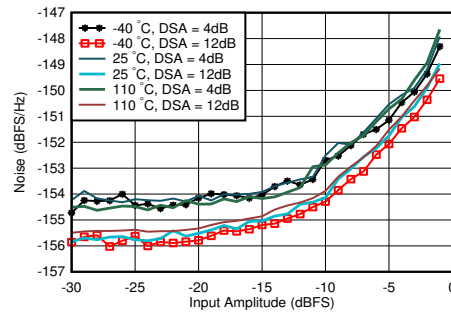
图 5-298. 0.8GHz 条件下 RX 噪声频谱密度与输入振幅和温度间的关系
