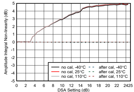
图 5-451. 9.6GHz 条件下 RX 振幅积分非线性
