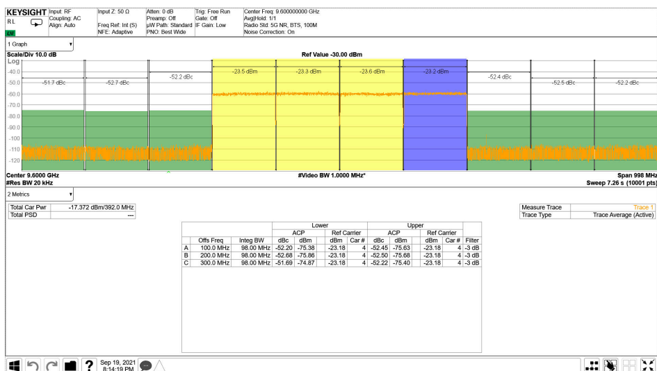
图 5-283. 9.61GHz 条件下 TX NR100MHz 输出频谱
