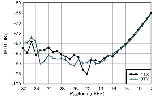
图 5-29. 0.85GHz 条件下 TX IMD3 与数字电平间的关系
