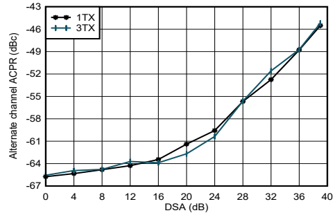
图 5-109. 2.6GHz 条件下 TX 20MHz LTE alt-ACPR 与 DSA 间的关系
