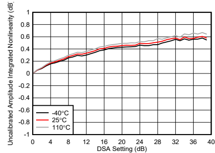
图 5-193. 8.1GHz 条件下 TX DSA 未校准振幅积分非线性
