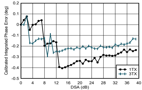
图 5-125. 3.5GHz 条件下 TX 校准差分相位误差与 DSA 设置和通道间的关系
