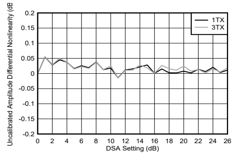
图 5-236. TX DSA 未校准振幅微分非线性
