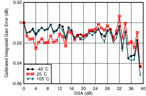
图 5-131. 3.5GHz 条件下 TX 校准积分增益误差与 DSA 设置和温度间的关系
