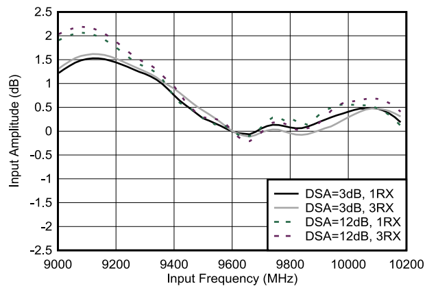
标准化为 9.6 GHz 图 5-448. RX 输入振幅与频率间的关系
