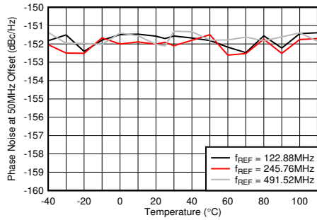
图 5-498. f_{OUT} = 2.6\text{GHz} 时 10GHz VCO 相位噪声 (50MHz 条件下) 与温度和 f_{REF} 间的关系
