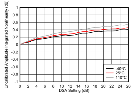
图 5-242. TX DSA 未校准振幅积分非线性
