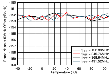
图 5-487. f_{OUT} = 2.6\text{GHz} 时 12GHz VCO 相位噪声 (50MHz 偏移条件下) 与温度和 f_{REF} 间的关系
