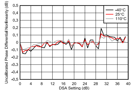
图 5-197. 8.1GHz 条件下 TX DSA 未校准相位微分非线性
