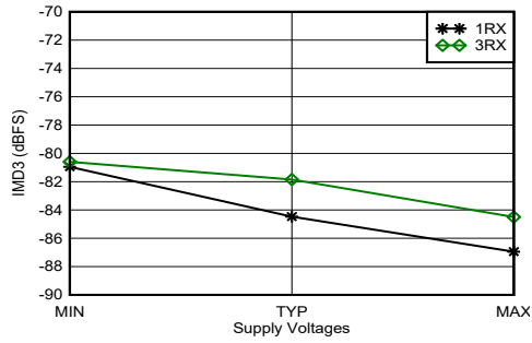
图 5-364. 2.6GHz 条件下 RX IMD3 与电源和通道间的关系
