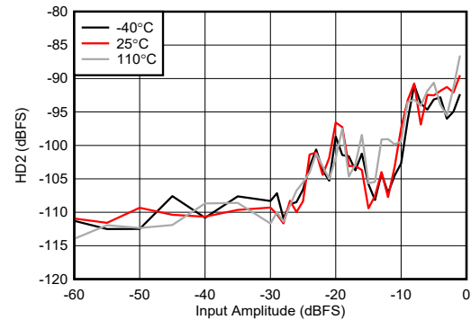
图 5-461. 9.6GHz 条件下 RX HD2 与数字电平间的关系
