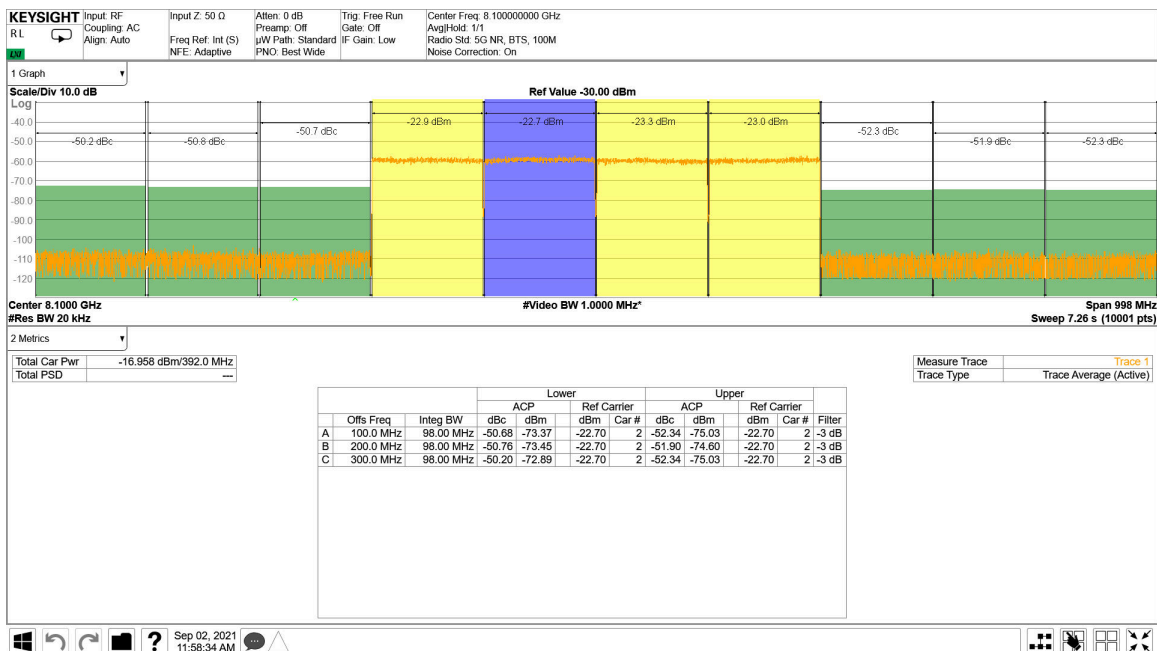
图 5-231. 8.11GHz 条件下 TX 4x100MHz NR 输出频谱
