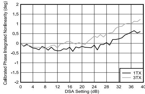
图 5-200. 8.1GHz 条件下 TX DSA 已校准相位积分非线性
