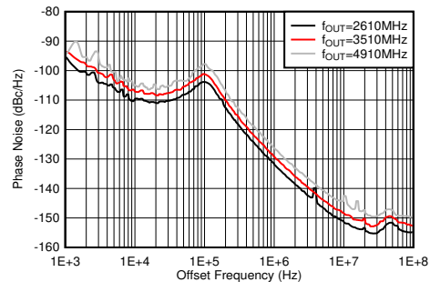
图 5-477. 25^\circ\text{C} 条件下 12GHz VCO 相位噪声与偏移频率和 f_{\text{OUT}} 间的关系
