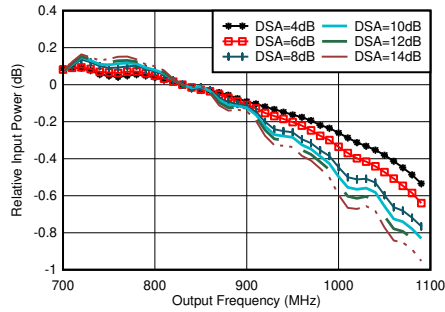
图 5-285. 通道 1RX 的 RX 带内增益平坦度， f_{\text{IN}} = 830\text{MHz}
