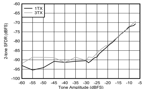
50MHz 频率间隔 图 5-264. 9.61GHz 条件下 TX 双音 SFDR 与数字振幅间的关系
