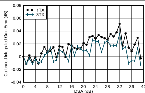
图 5-81. 2.6GHz 条件下 TX 校准差分增益误差与 DSA 设置和通道间的关系
