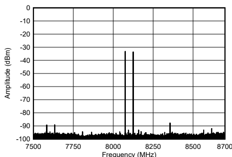
图 5-212. 8.1GHz 条件下 TX 双音输出频谱
