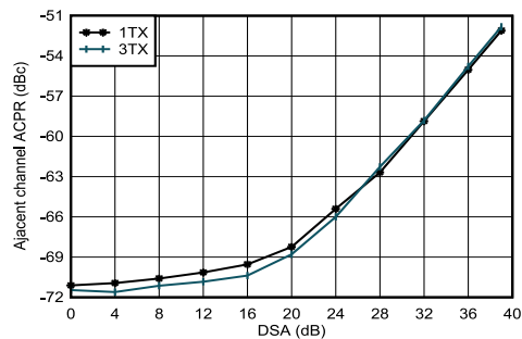
图 5-104. 2.6GHz 条件下 TX 20MHz LTE ACPR 与数字电平间的关系
