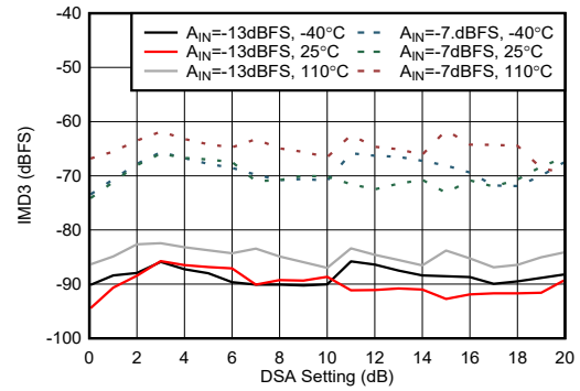
图 5-455. 9.6 GHz 条件下 RX IMD3 与 DSA 设置间的关系
