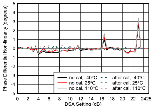
图 5-426. 8.1GHz 条件下 RX 相位微分非线性
