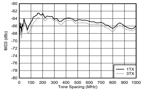
图 5-256. 9.61GHz 条件下 TX IMD3 与频率间隔间的关系
