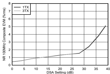
图 5-228. 8.11GHz 条件下 TX NR100MHz EVM 与 DSA 设置间的关系
