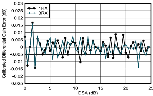
图 5-320. 1.75GHz 条件下 RX 校准差分振幅误差与 DSA 设置间的关系
