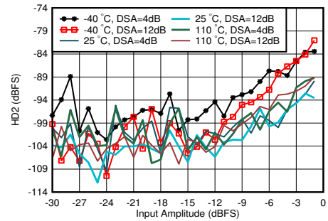
图 5-335. 1.9GHz 条件下 RX HD2 与 DSA 设置和温度间的关系
