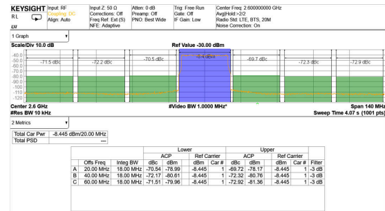
图 5-103. 2.6GHz (频带 41) 条件下的 TX 20MHz LTE 输出频谱
