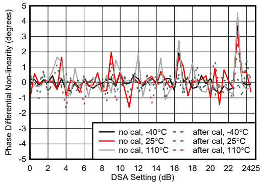
图 5-452. 9.6GHz 条件下 RX 相位微分非线性
