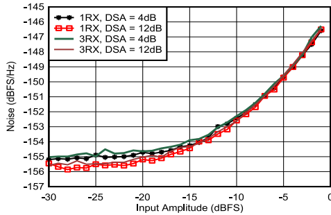
图 5-330. 1.75GHz 条件下 RX 噪声频谱密度与输入振幅和通道间的关系
