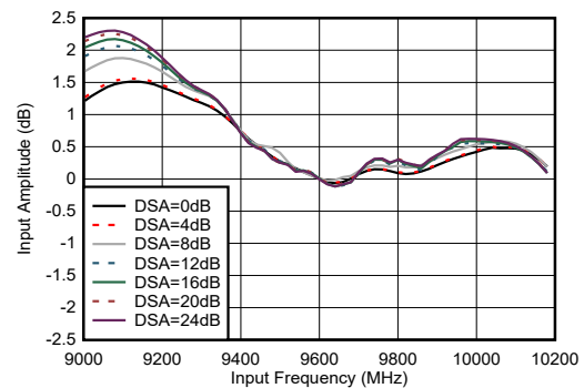
标准化为 9.6 GHz 图 5-449. 9.6GHz 条件下 RX 输入振幅与频率间的关系
