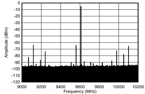
图 5-266. 9.61GHz 和 -1dBFS (1.2 GHz 带宽) 条件下 TX 单音频谱
