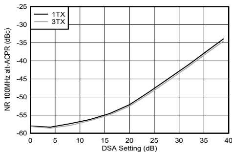
图 5-281. 9.61GHz 条件下 TX NR100MHz alt-ACPR 与 DSA 设置间的关系
