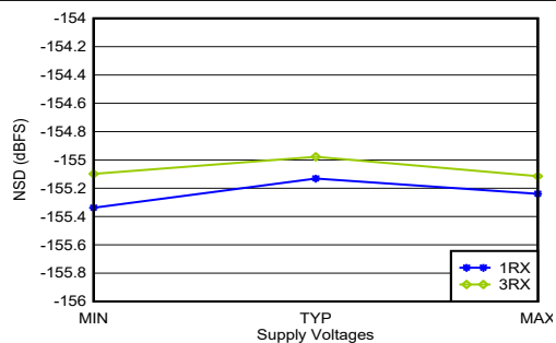
图 5-315. 0.8GHz 条件下 RX 噪声频谱密度与电源和通道间的关系
