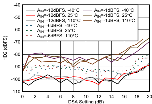
图 5-462. 9.6 GHz 条件下 RX HD2 与 DSA 设置间的关系
