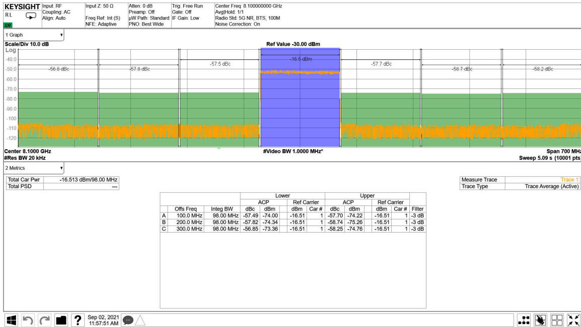
图 5-229. 8.1GHz 条件下 TX 100MHz NR 输出频谱
