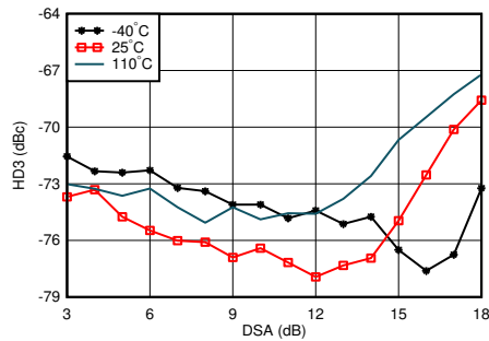
图 5-384. 3.6GHz 条件下 RX HD3 与 DSA 设置和温度间的关系
