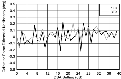
图 5-196. 8.1GHz 条件下 TX DSA 已校准相位微分非线性
