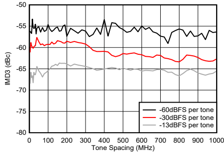
图 5-257. 9.61GHz 条件下 TX IMD3 与频率间隔间的关系
