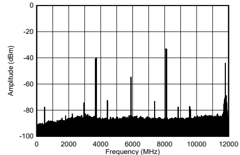
图 5-211. 8.1GHz 条件下 TX 双音输出频谱
