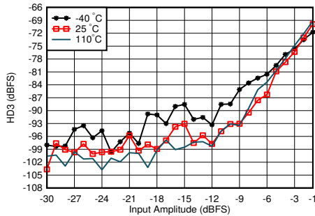
图 5-417. 4.9GHz 条件下 RX HD3 与输入电平和温度间的关系
