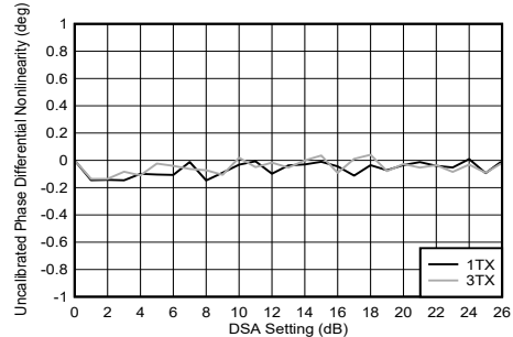
图 5-244. TX DSA 未校准相位微分非线性
