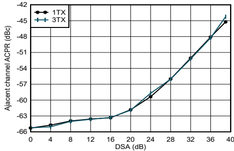
图 5-108. 2.6GHz 条件下 TX 20MHz LTE ACPR 与 DSA 间的关系
