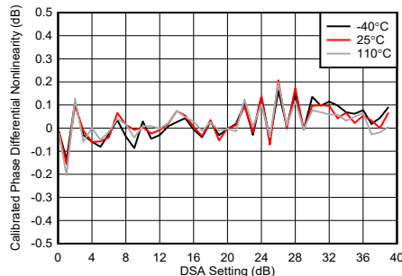
图 5-198. 8.1GHz 条件下 TX DSA 已校准相位微分非线性
