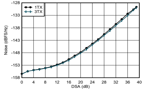
图 5-168. 2.6GHz 条件下 TX 输出噪声与通道和衰减间的关系
