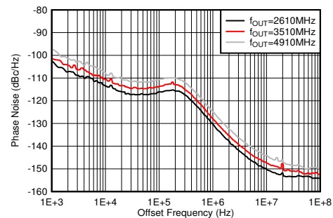
图 5-489. 25°C 条件下的 10GHz VCO 相位噪声与偏移频率和 f_{OUT} 间的关系
