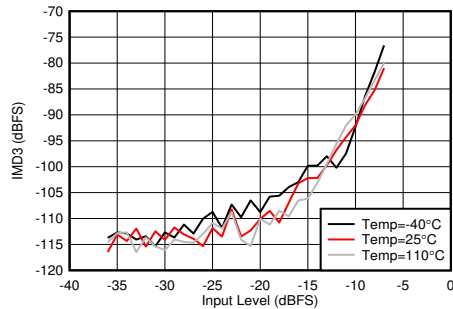
图 5-354. 2.6GHz 条件下 RX IMD3 与输入电平和温度间的关系
