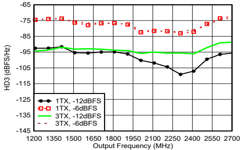
图 5-74. 1.8GHz 条件下 TX HD3 与数字振幅和输出频率间的关系
