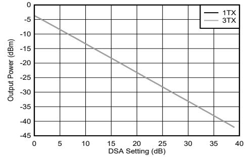
图 5-185. 8.11 GHz 条件下 TX 输出功率与 DSA 设置间的关系
