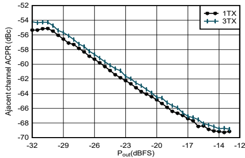
图 5-175. 4.9GHz 条件下 TX 20MHz LTE ACPR 与数字电平间的关系
