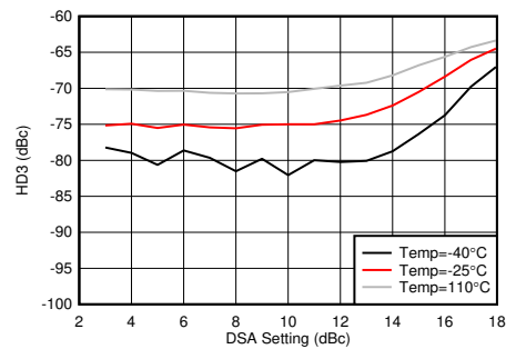
图 5-359. 2.6GHz 条件下 RX HD3 与 DSA 设置和温度间的关系
