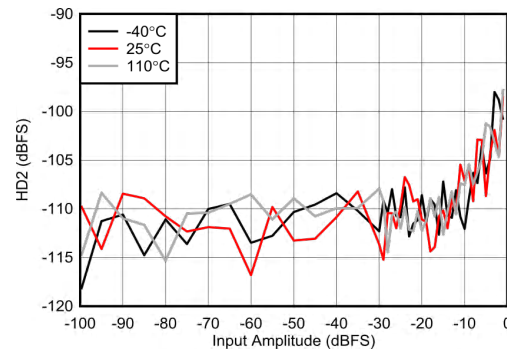
图 7-156. 3.76GHz 条件下 RX HD2 与输入电平间的关系
