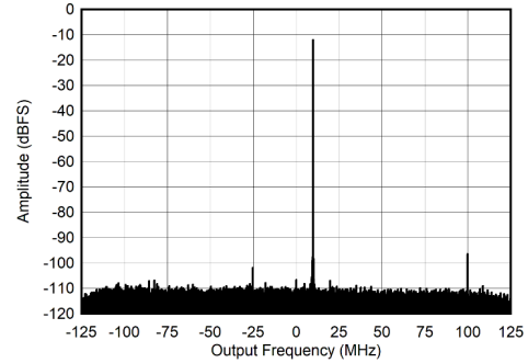
图 7-40. 405MHz 和 -12dBFS 条件下的 RX 输出 FFT
