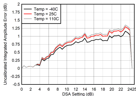
图 7-32. 400MHz 条件下 RX 未校准积分振幅误差与 DSA 设置间的关系
