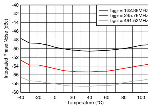
图 7-616. f_{OUT} = 2.6\text{GHz} 时 10GHz VCO 积分相位噪声与温度和 f_{REF} 间的关系
