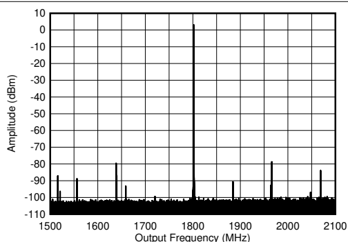
图 7-375. 1.8GHz ( \pm 300\text{MHz} ) 条件下的 TX 单音 ( -6\text{dBFS} ) 输出频谱
