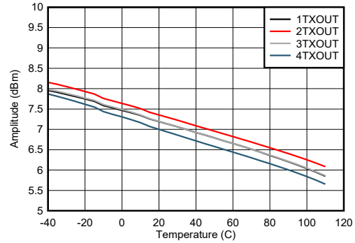
图 7-234. 30MHz 条件下 TX 输出满量程与温度间的关系
