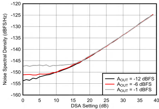
图 7-581. 7.1GHz 条件下 NSD 与 DSA 设置和振幅间的关系
