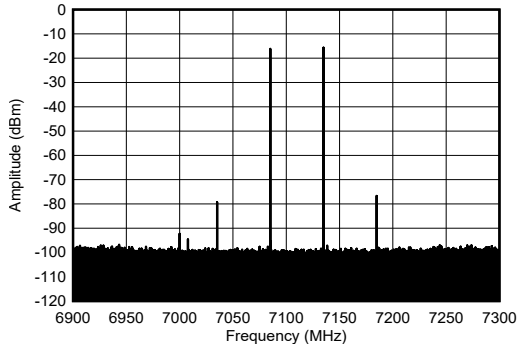
图 7-593. 7.1GHz、单音幅值为 -7dBFS (带内) 条件下的双音输出频谱
