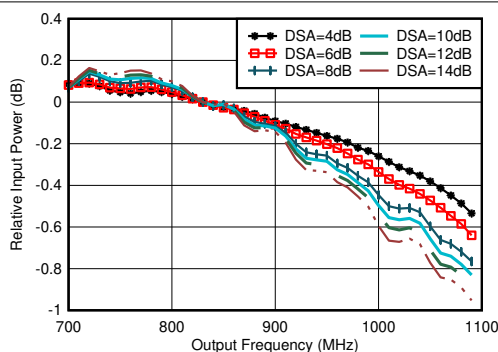
图 7-50. 通道 1RX 的 RX 带内增益平坦度， f_{\text{IN}} = 830\text{MHz}
