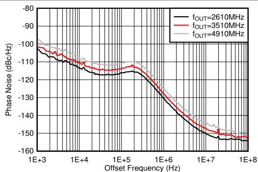
图 7-615. 110°C 条件下 10GHz VCO 相位噪声与偏移频率和 f_{OUT} 间的关系
