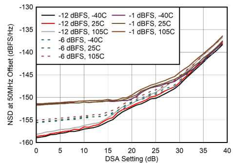
图 7-298. 400MHz 条件下的噪声频谱密度与 DSA 设置间的关系
