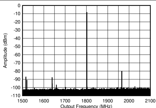
图 7-377. 1.8GHz ( \pm 300\text{MHz} ) 条件下的 TX 单音 ( -1\text{dBFS} ) 输出频谱
