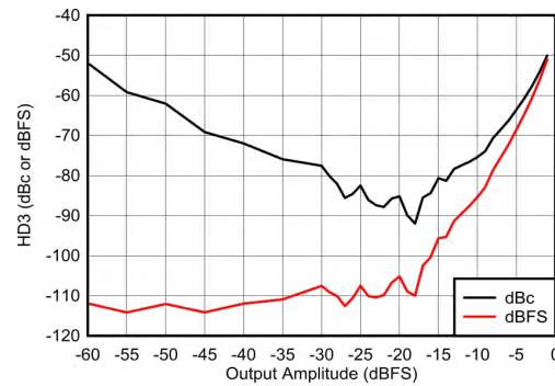
图 7-302. 400MHz 条件下 HD3 与振幅间的关系
