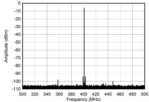
图 7-284. 400MHz 和 -12dBFS (±100MHz) 条件下的单音频谱
