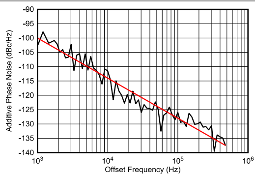
图 7-232. 6.85GHz 条件下的 RX 附加相位噪声
