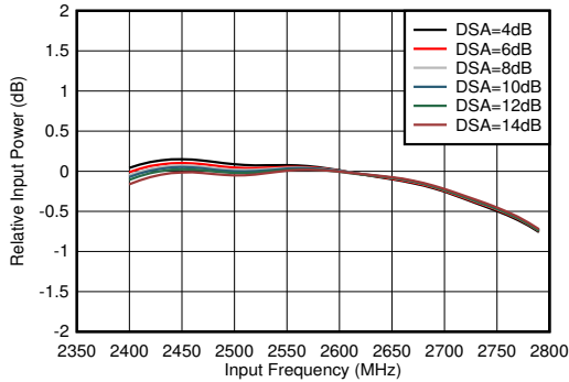
图 7-111. RX 带内增益平坦度， f_{\text{IN}} = 2600\text{MHz}
