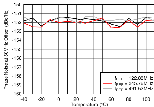
图 7-622. f_{OUT} = 2.6\text{GHz} 时 10GHz VCO 相位噪声 (50MHz 条件下) 与温度和 f_{REF} 间的关系
