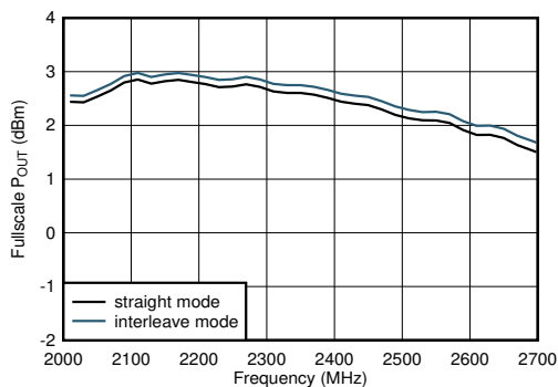
图 7-384. 5898.24MSPS 条件下 TX 满量程与射频频率间的关系
