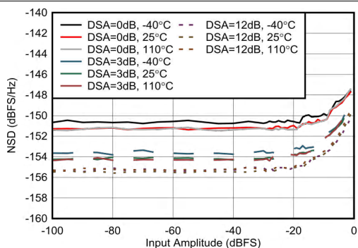
图 7-165. 3.76GHz 条件下 RX 噪声频谱密度与输入电平间的关系
