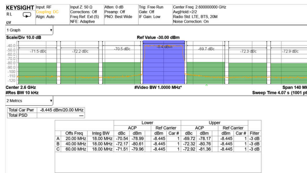
图 7-412. 2.6GHz (频带 41) 条件下的 TX 20MHz LTE 输出频谱
