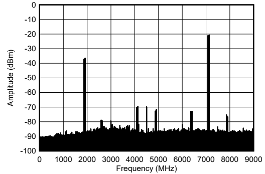
图 7-592. 7.1GHz、单音幅值为 -7dBFS (0 - F_{\text{DAC}} ) 条件下的双音输出频谱
