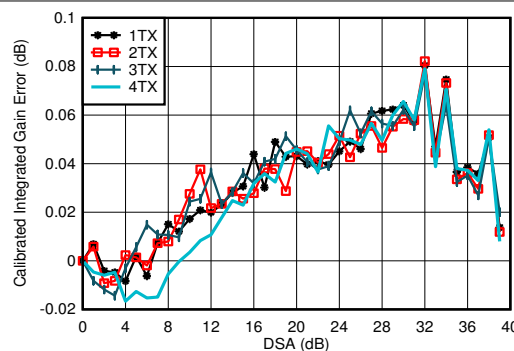
图 7-312. 0.85GHz 条件下 TX 校准差分增益误差与 DSA 设置和通道间的关系
