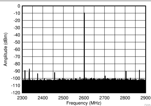
图 7-425. 2.6GHz 条件下双频带内固定杂散与数字振幅间的关系
