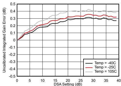
图 7-239. 30MHz 条件下的未校准 TX 积分增益误差 (INL)
