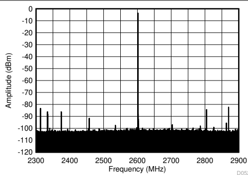
图 7-427. 2.6GHz ( \pm 300\text{MHz} ) 条件下的 TX 单音 (-12dBFS) 输出频谱
