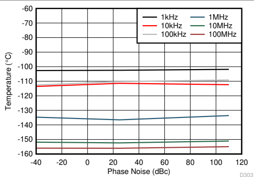
图 7-627. f_{OUT} = 2.6\text{GHz} 时 9GHz VCO 相位噪声与温度和偏移频率间的关系
