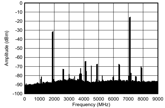
图 7-590. 7.1GHz、-12dBFS (0 - F_{\text{DAC}} ) 条件下的单音输出频谱
