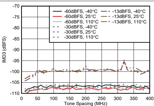
图 7-223. 6.851GHz 条件下 RX IMD3 与子载波间隔间的关系
