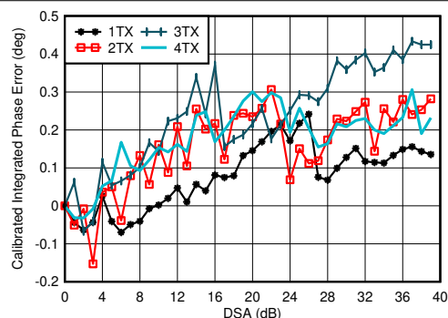
图 7-520. 4.9GHz 条件下 TX 校准差分相位误差与 DSA 设置和通道间的关系
