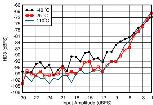
图 7-197. 4.9GHz 条件下 RX HD3 与输入电平和温度间的关系
