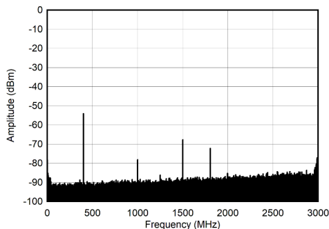
图 7-287. 400MHz 和 -60dBFS (奈奎斯特) 条件下的单音频谱
