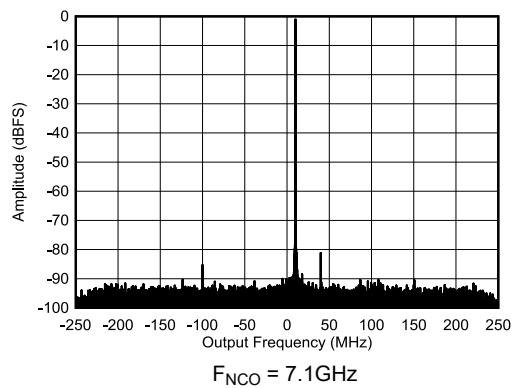
图 7-211. 7.11GHz 和 -1dBFS 条件下的单频 RX 输出 FFT
