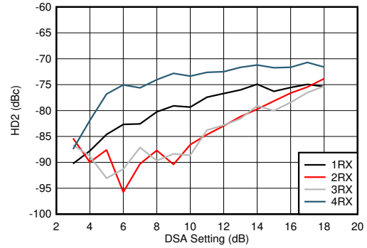
图 7-124. 2.6GHz 条件下 RX HD2 与 DSA 设置和通道间的关系
