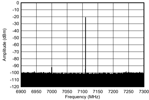
图 7-591. 7.1GHz、-12dBFS (带内) 条件下的单音输出频谱
