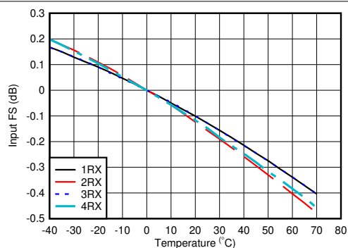
图 7-82. 1.75GHz 条件下 RX 输入满量程与温度和通道间的关系
