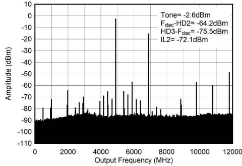
图 7-546. 4.9GHz (0 - f_{\text{DAC}} ) 条件下的 TX 单音 (-1dBFS) 输出频谱
