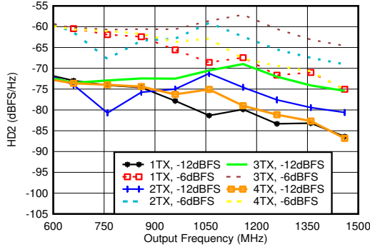
图 7-347. 0.85GHz 条件下 TX HD2 与数字振幅和输出频率间的关系
