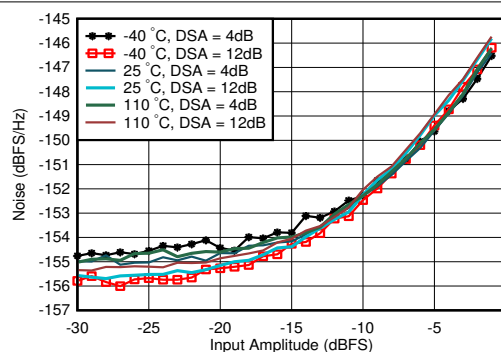
图 7-94. 1.75GHz 条件下 RX 噪声频谱密度与输入振幅和温度间的关系
