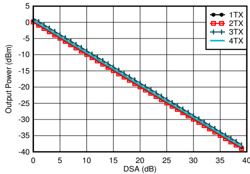
图 7-453. 3.5GHz 条件下 TX 输出功率与 DSA 设置间的关系
