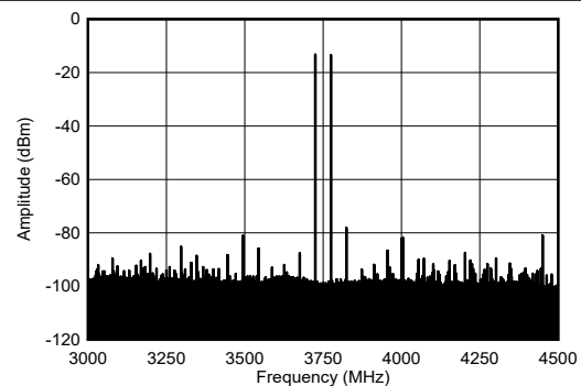
图 7-500. 3.75GHz、单音幅值为 -7dBFS ( \pm 600\text{MHz} ) 条件下的 TX 双音输出频谱
