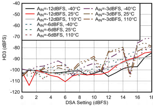
图 7-230. 6.851GHz 条件下 RX HD3 与 DSA 设置间的关系
