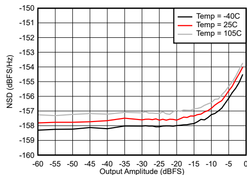
图 7-264. 30MHz 条件下噪声频谱密度与数字振幅间的关系
