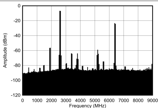
图 7-436. 2.6GHz (0- f_{\text{DAC}} ) 条件下的 TX 单音 (-1dBFS) 输出频谱
