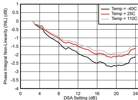
图 7-8. 30MHz 条件下 RX 未校准积分相位误差与 DSA 设置间的关系
