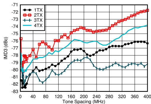
图 7-330. 0.85GHz 条件下 TX IMD3 与频率间隔和通道间的关系
