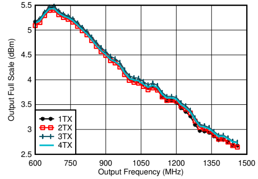
图 7-304. 8847.36MSPS 条件下 TX 满量程与射频频率和通道间的关系, 直接模式
