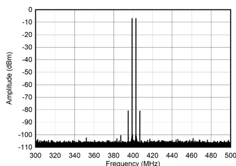
图 7-290. 400MHz 和 -7dBFS ( \pm 100\text{MHz} ) 条件下的双频频谱
