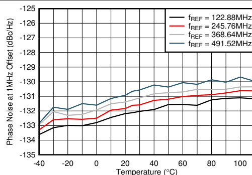
图 7-608. f_{OUT} = 2.6\text{GHz} 时 12GHz VCO 相位噪声 (1MHz 偏移条件下) 与温度和 f_{REF} 间的关系
