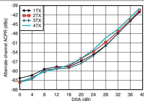
图 7-541. 4.9GHz 条件下 TX 20MHz LTE alt-ACPR 与 DSA 间的关系
