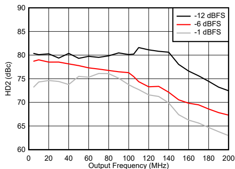
图 7-267. HD2 与频率 (0 - 200MHz) 间的关系
