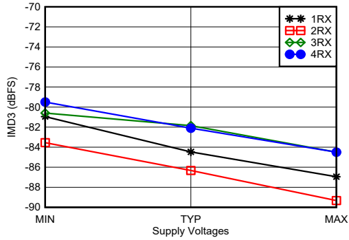
图 7-135. 2.6GHz 条件下 RX IMD3 与电源和通道间的关系
