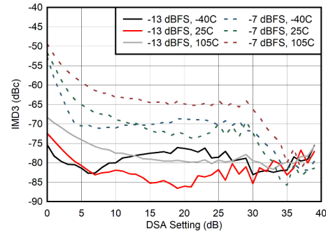
图 7-300. 400MHz 条件下 IMD3 与 DSA 设置间的关系
