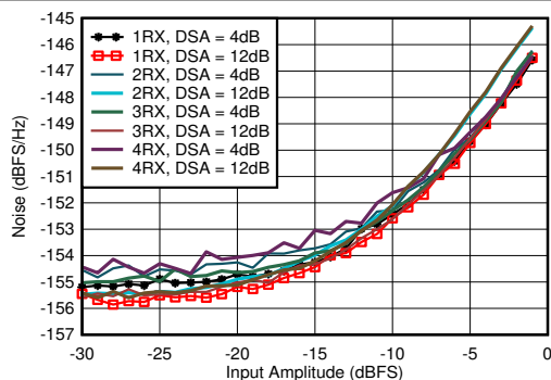
图 7-95. 1.75GHz 条件下 RX 噪声频谱密度与输入振幅和通道间的关系
