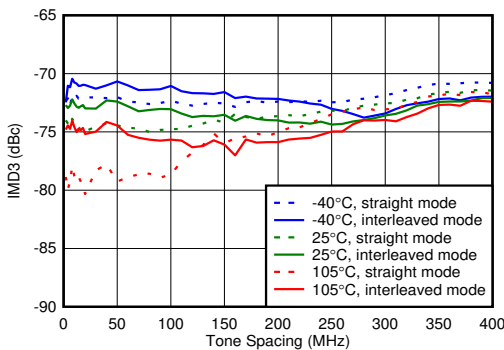
图 7-408. 2.6GHz 条件下 TX IMD3 与频率间隔和温度间的关系
