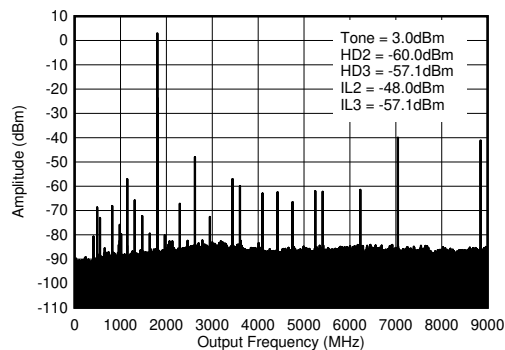
图 7-376. 1.8GHz ( 0 - f_{\text{DAC}} ) 条件下的 TX 单音 ( -1\text{dBFS} ) 输出频谱
