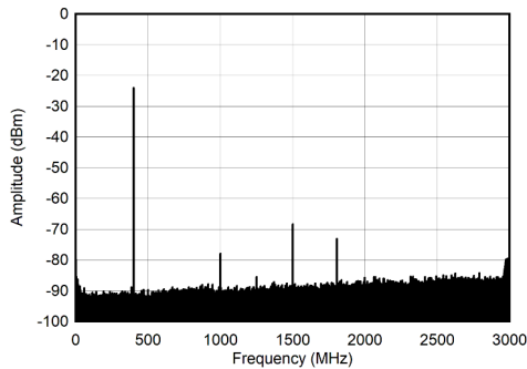
图 7-285. 400MHz 和 -30dBFS (奈奎斯特) 条件下的单音频谱
