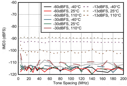
图 7-123. 2.6GHz (外部时钟) 条件下 RX IMD3 与子载波间隔间的关系
