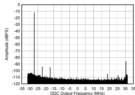
图 7-10. 5MHz 条件下的 RX 输出 FFT
