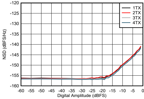
图 7-473. 3.75GHz 条件下 TX NSD 与数字振幅和通道间的关系
