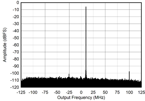
图 7-39. 405MHz 和 -6dBFS 条件下的 RX 输出 FFT
