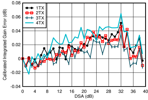
图 7-390. 2.6GHz 条件下 TX 校准差分增益误差与 DSA 设置和通道间的关系
