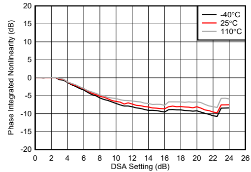
图 7-209. 6.851GHz 条件下的 RX 未校准积分相位误差
