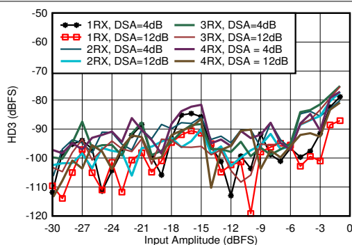
图 7-105. 1.9GHz 条件下 RX HD3 与输入电平和通道间的关系
