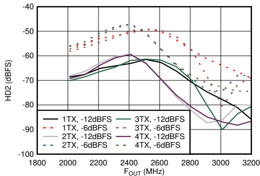
在 2.6GHz 条件下匹配, f_{\text{DAC}} = 11.79648\text{GSPPS} , 交错模式, 标准化为谐波频率下的输出功率
