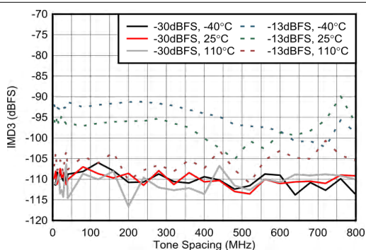
图 7-149. 3.6GHz 条件下 RX IMD3 与输入电平和温度间的关系
