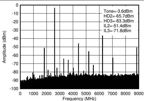
图 7-426. 2.6GHz (0 - f_{\text{DAC}} ) 条件下的 TX 单音 (-12dBFS) 输出频谱
