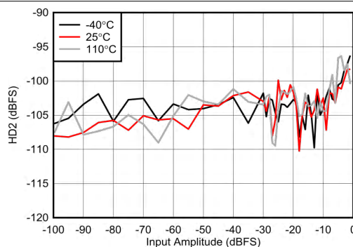
图 7-225. 6.851GHz 条件下 RX HD2 与输入振幅间的关系
