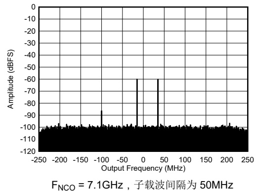
图 7-219. 7.1GHz、每个子载波 -60dBFS 条件下的双频 RX 输出 FFT
