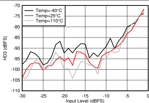
图 7-161. 3.6GHz 条件下 RX HD3 与输入电平和温度间的关系
