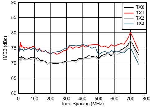
图 7-577. 7.1GHz 条件下 IMD3 与频率间隔和通道间的关系
