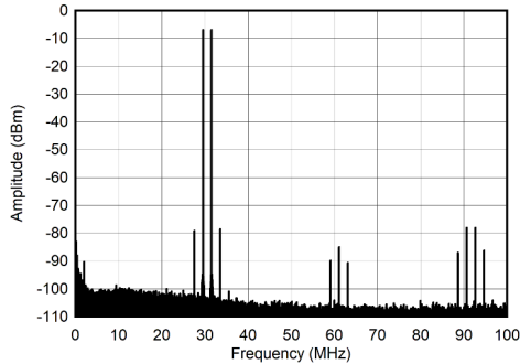
图 7-261. 30MHz 和 -13dBFS (0 - 100MHz) 条件下的双频频谱
