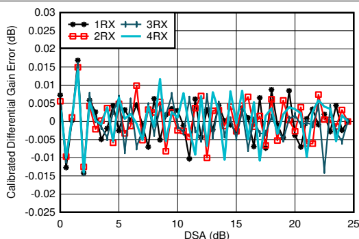
图 7-85. 1.75GHz 条件下 RX 校准差分振幅误差与 DSA 设置间的关系
