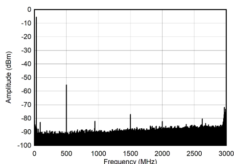
图 7-254. 30MHz 和 -12dBFS (奈奎斯特) 条件下的单音频谱
