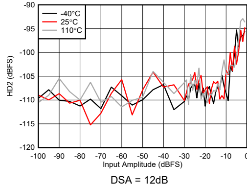
图 7-227. 6.851GHz 条件下 RX HD2 与输入振幅间的关系
