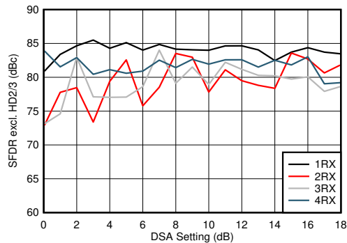
图 7-167. RX SFDR，在 3.6GHz 时不包括 HD2/3 与 DSA 设置和通道间的关系
