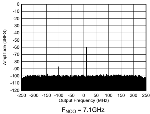
图 7-216. 7.1GHz 和 -60dBFS 条件下的单频 RX 输出 FFT
