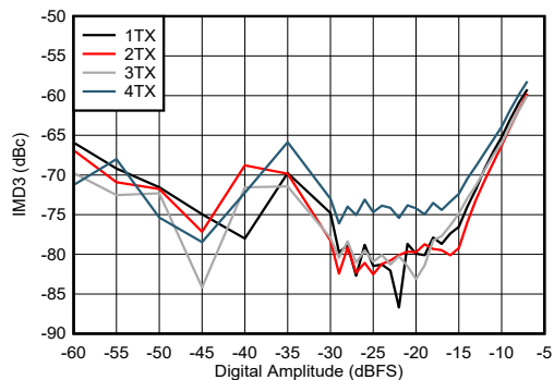
图 7-475. 3.5GHz 条件下 TX IMD3 与数字振幅和通道间的关系
