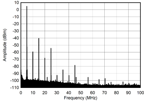
图 7-245. 5MHz 和 -1dBFS (0 - 100MHz) 条件下的单音频谱
