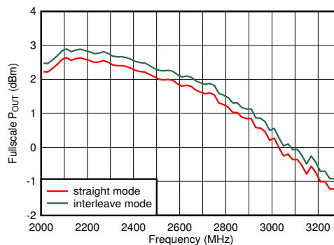
图 7-385. 8847.36MSPS 条件下 TX 满量程与射频频率间的关系
