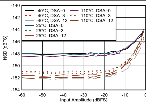
图 7-220. 6.851GHz 条件下 RX NSD 与输入振幅间的关系
