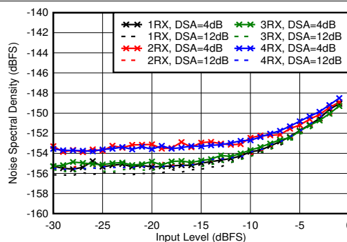
图 7-164. 3.6GHz 条件下 RX 噪声频谱密度与输入电平和 DSA 设置间的关系
