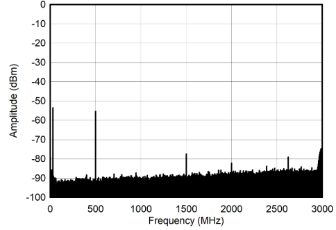
图 7-258. 30MHz 和 -60dBFS (奈奎斯特) 条件下的单音频谱
