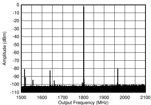
图 7-381. 1.8GHz ( \pm 300\text{MHz} ) 条件下的 TX 单音 ( -6\text{dBFS} ) 输出频谱
