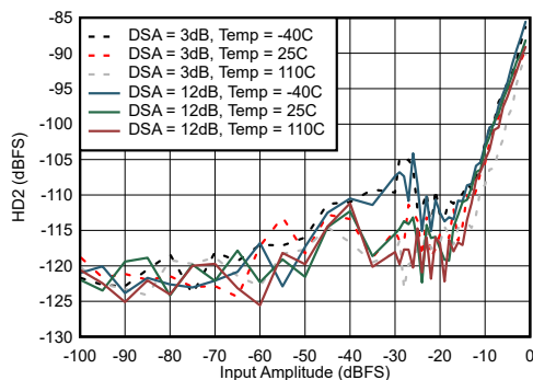
图 7-25. 30MHz 条件下 HD2 与输入振幅间的关系
