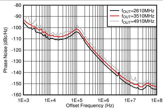
图 7-603. 110°C 条件下 12GHz VCO 相位噪声与偏移频率和 f_{OUT} 间的关系
