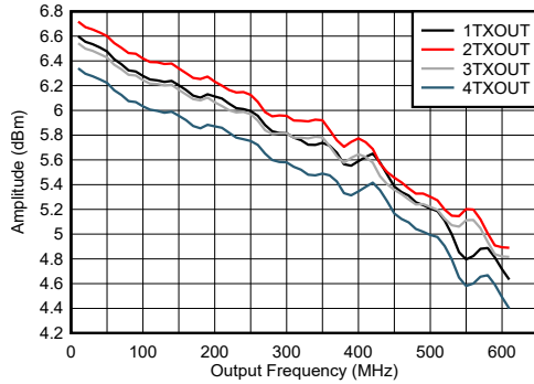
图 7-233. TX 输出满量程与输出频率间的关系: 5 MHz - 600 MHz
