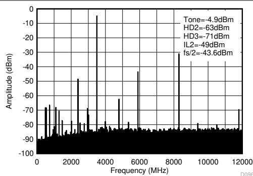
图 7-495. 3.5GHz (0 - f_{\text{DAC}} ) 条件下的 TX 单音 (-6dBFS) 输出频谱
