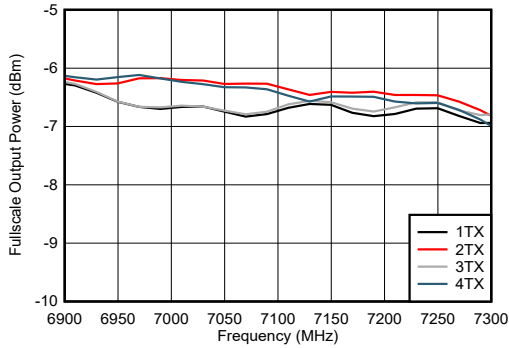
图 7-553. TX 满量程与射频频率和通道间的关系
