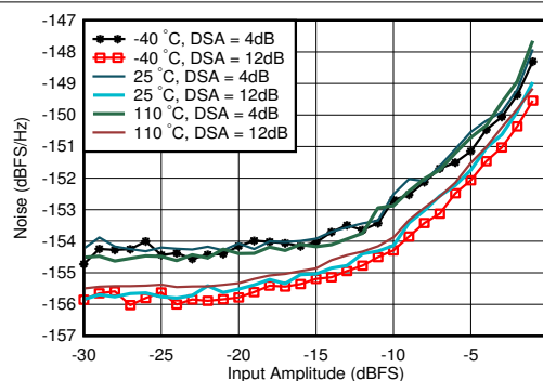
图 7-63. 0.8GHz 条件下 RX 噪声频谱密度与输入振幅和温度间的关系
