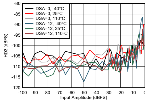
图 7-229. 6.851GHz 条件下 RX HD3 与输入振幅间的关系
