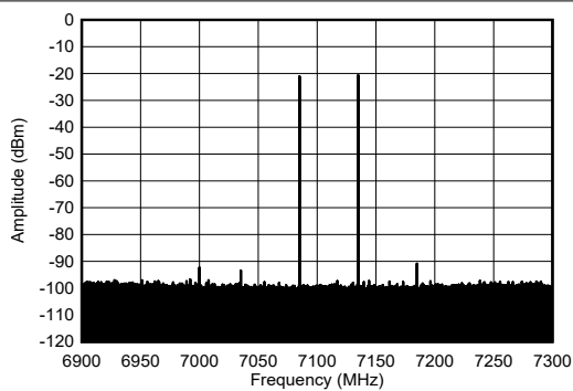
图 7-595. 7.1GHz、单音幅值为 -12dBFS (带内) 条件下的双音输出频谱
