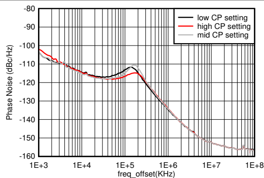
图 7-604. f_{OUT} = 2.6\text{GHz} 时 12GHz VCO 相位噪声与偏移频率和 CP 设置间的关系
