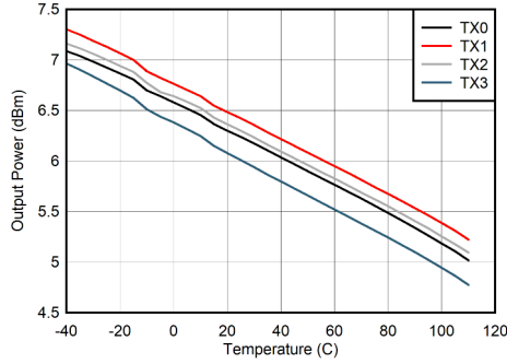
图 7-269. 400MHz 条件下 TX 输出满量程与温度间的关系
