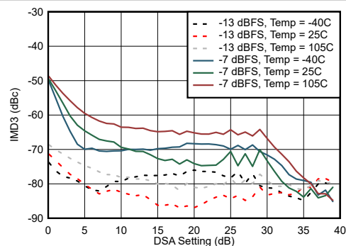
图 7-266. 30MHz 条件下 IMD3 与 DSA 设置间的关系
