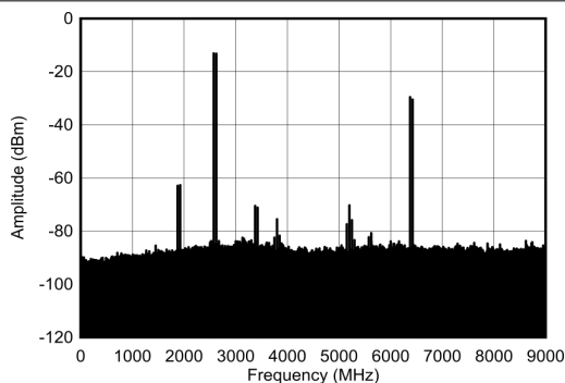
图 7-438. 2.6GHz、单音幅值为 -7dBFS (0 - f_{\text{DAC}} ) 条件下的 TX 双音输出频谱
