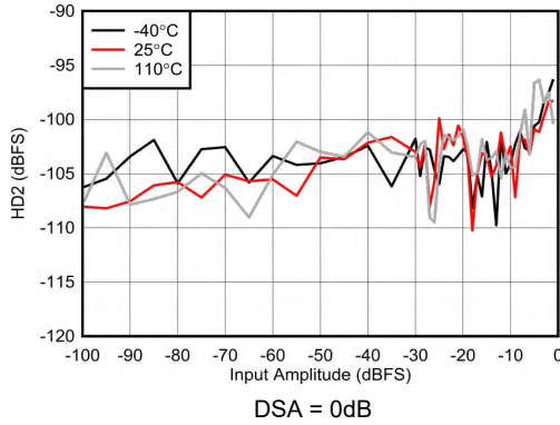
图 7-226. 6.851GHz 条件下 RX HD2 与输入振幅间的关系
