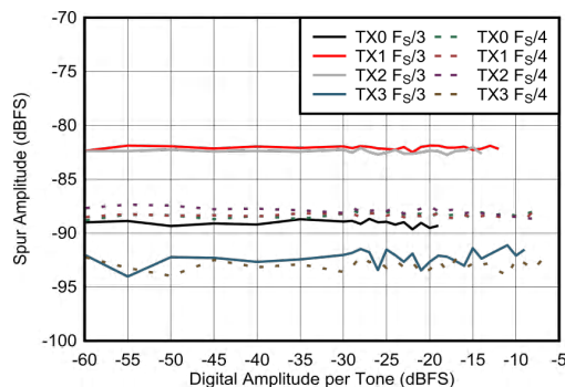
图 7-425. 2.6GHz 条件下双频带内固定杂散与数字振幅间的关系
