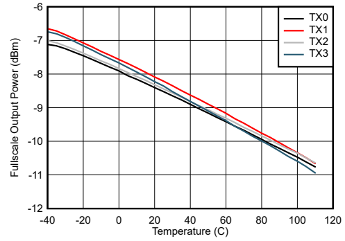
图 7-554. 7.1GHz 条件下 TX 满量程与温度和通道间的关系
