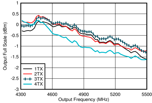
图 7-506. 11796.48MSPS 条件下的 TX 满量程与射频频率和通道间的关系
