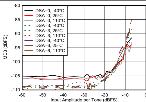
图 7-221. 6.851GHz 条件下 RX IMD3 与输入振幅间的关系
