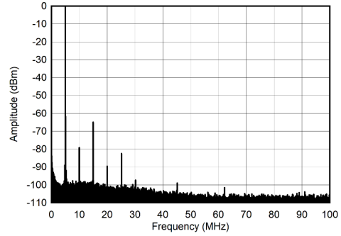
图 7-246. 5MHz 和 -6dBFS (0 - 100MHz) 条件下的单音频谱
