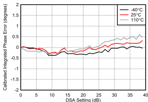
图 7-571. 7.1GHz 条件下校准积分相位误差与温度间的关系
