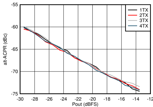
图 7-414. 2.6GHz 条件下 TX 20MHz LTE alt-ACPR 与数字电平间的关系
