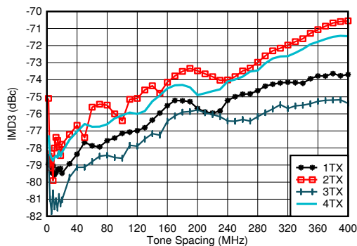
图 7-329. 0.85GHz 条件下 TX IMD3 与频率间隔和通道间的关系
