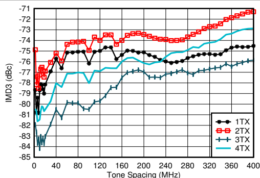
图 7-329. 0.85GHz 条件下 TX IMD3 与频率间隔和通道间的关系
