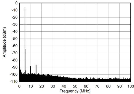
图 7-247. 5MHz 和 -12dBFS (0 - 100MHz) 条件下的单音频谱
