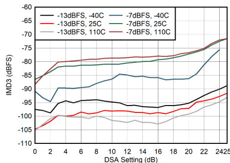
图 7-46. 400MHz 条件下 IMD3 与 DSA 设置间的关系
