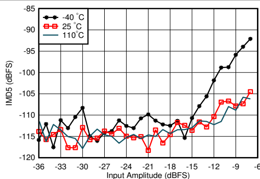
图 7-69. 0.8GHz 条件下 Rx IMD5 与输入电平和温度间的关系
