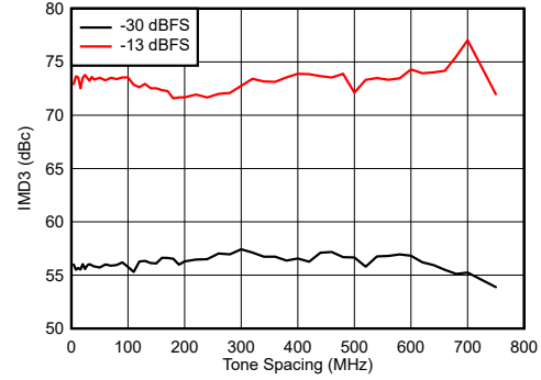
图 7-578. 7.1GHz 条件下 IMD3 与频率间隔和数字振幅间的关系
