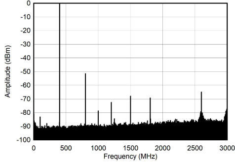
图 7-281. 400MHz 和 -6dBFS (奈奎斯特) 条件下的单音频谱
