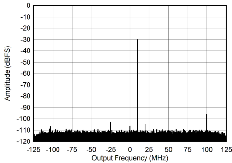
图 7-41. 405MHz 和 -30dBFS 条件下的 RX 输出 FFT
