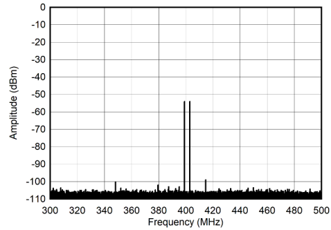
图 7-296. 400MHz 和 -60dBFS (±100MHz) 条件下的双频频谱
