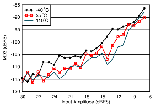
图 7-68. 0.8GHz 条件下 RX IMD3 与输入电平和温度间的关系
