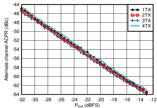
图 7-537. 4.9GHz 条件下 TX 20MHz LTE alt-ACPR 与数字电平间的关系
