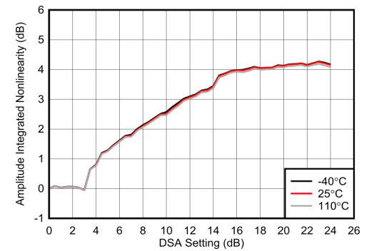
图 7-205. 6.851GHz 条件下的 RX 未校准积分振幅误差
