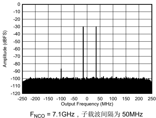
图 7-218. 7.1GHz、每个子载波 -30dBFS 条件下的双频 RX 输出 FFT
