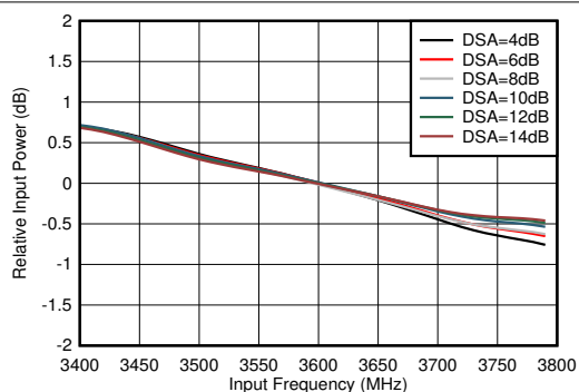
图 7-137. RX 带内增益平坦度， f_{\text{IN}} = 3600\text{MHz}
