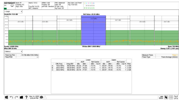
图 7-535. 4.9GHz 条件下的 TX 100MHz NR 输出频谱
