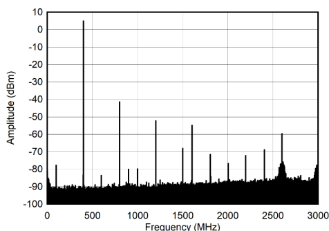
图 7-279. 400MHz 和 -1dBFS (奈奎斯特) 条件下的单音频频谱
