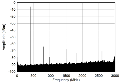
图 7-283. 400MHz 和 -12dBFS (奈奎斯特) 条件下的单音频谱
