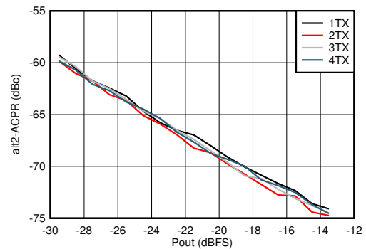
图 7-413. 2.6GHz 条件下 TX 20MHz LTE ACPR 与数字电平间的关系
