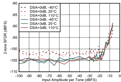
图 7-168. 3.7GHz 条件下 RX 2 子载波 SFDR 与输入振幅和 DSA 设置间的关系
