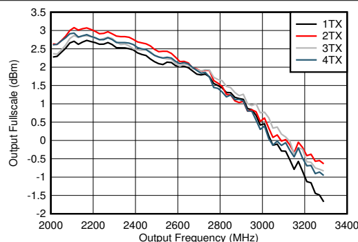
图 7-385. 8847.36MSPS 条件下 TX 满量程与射频频率间的关系
