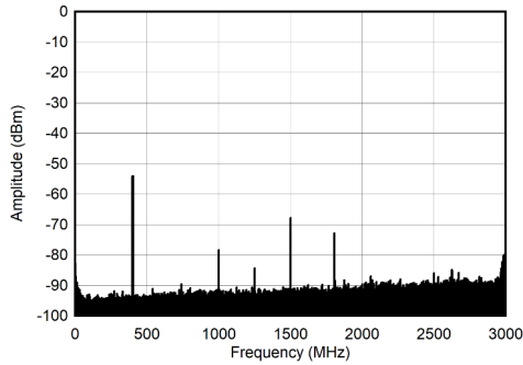
图 7-295. 400MHz 和 -60dBFS (奈奎斯特) 条件下的双频频谱
