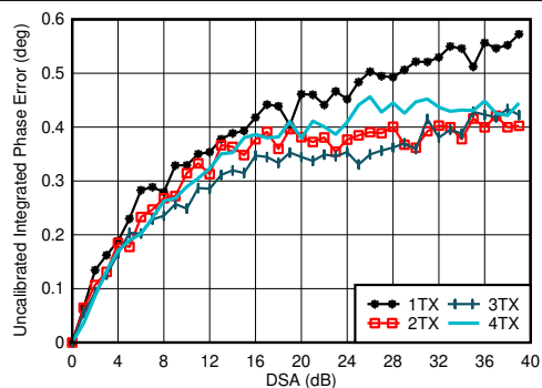
图 7-459. 3.5GHz 条件下 TX 未校准差分相位误差与 DSA 设置和通道间的关系
