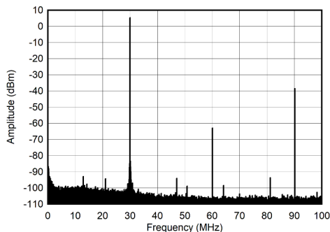
图 7-251. 30MHz 和 -1dBFS (0 - 100MHz) 条件下的单音频谱
