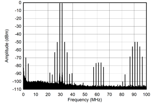
图 7-260. 30MHz 和 -7dBFS (0 - 100MHz) 条件下的双频频谱
