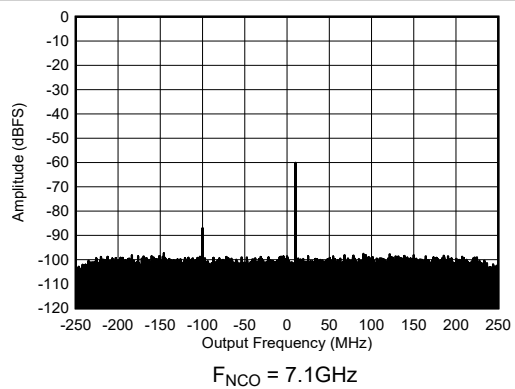
图 7-213. 7.11GHz 和 -6dBFS 条件下的单频 RX 输出 FFT
