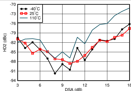
图 7-192. 4.9GHz 条件下 RX HD2 与 DSA 和温度间的关系
