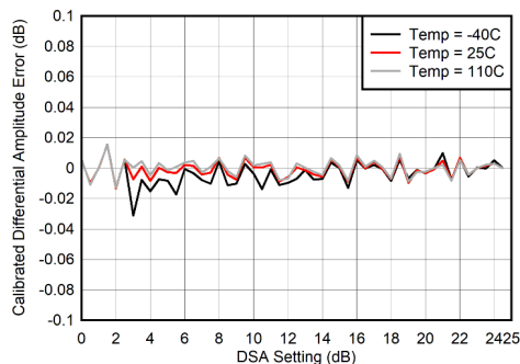
图 7-31. 400MHz 条件下 RX 校准差分振幅误差与 DSA 设置间的关系
