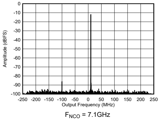
图 7-214. 7.1GHz 和 -12dBFS 条件下的单频 RX 输出 FFT
