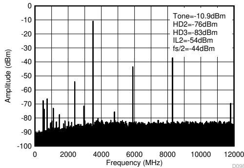
图 7-497. 3.5GHz (0 - f_{\text{DAC}} ) 条件下的 TX 单音 (-12dBFS) 输出频谱
