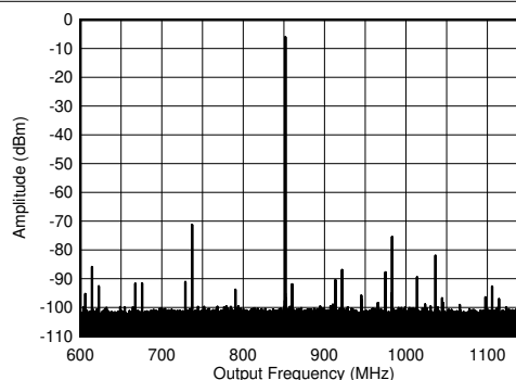
图 7-356. 0.85GHz ( \pm 300\text{MHz} ) 条件下的 TX 单音 (-1dBFS) 输出频谱
