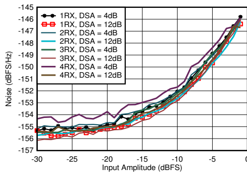
图 7-187. 4.9GHz 条件下 RX 噪声频谱密度与输入振幅和通道间的关系
