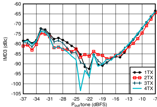
图 7-335. 0.85GHz 条件下 TX IMD3 与数字电平间的关系
