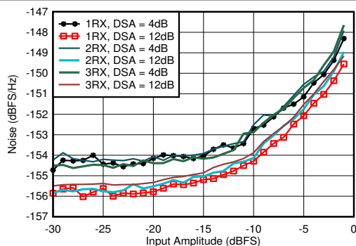
图 7-64. 0.8GHz 条件下 RX 噪声频谱密度与输入振幅和通道间的关系
