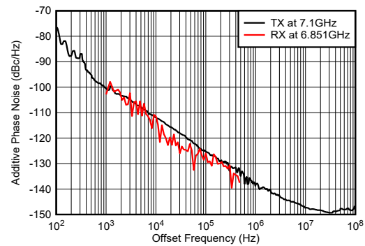
图 7-598. 7GHz 条件下的 TX 与 RX 附加相位噪声
