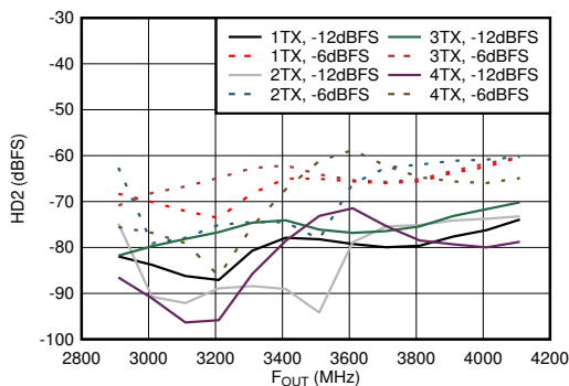
图 7-491. 3.5GHz 条件下 TX 单音 HD2 与频率和数字电平间的关系
