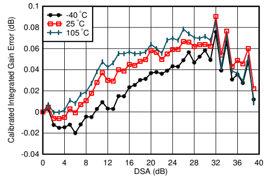
图 7-316. 0.85GHz 条件下 TX 校准差分增益误差与 DSA 设置和温度间的关系
