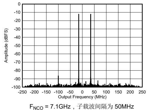
图 7-217. 7.1GHz、每个子载波 -12dBFS 条件下的双频 RX 输出 FFT
