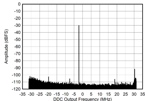
图 7-16. 30MHz 条件下的 RX 输出 FFT
