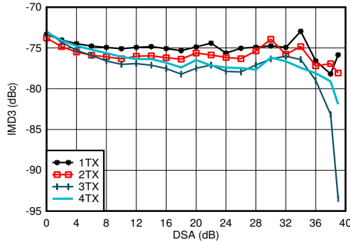
图 7-406. 2.6GHz 条件下 TX IMD3 与 DSA 设置间的关系
