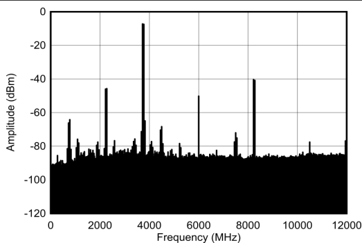
图 7-497. 3.5GHz (0 - f_{\text{DAC}} ) 条件下的 TX 单音 (-12dBFS) 输出频谱
