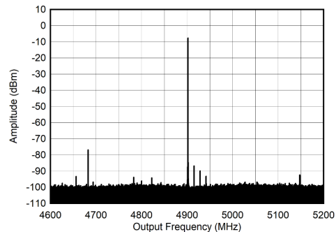
图 7-547. 4.9GHz ( \pm 300\text{MHz} ) 条件下的 TX 单音 (-1dBFS) 输出频谱
