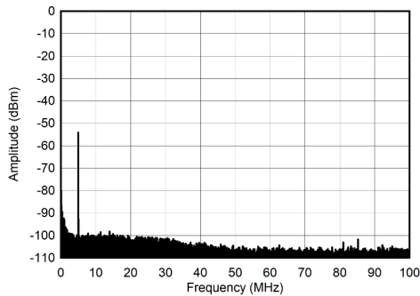
图 7-249. 5MHz 和 -60dBFS (0 - 100MHz) 条件下的单音频谱
