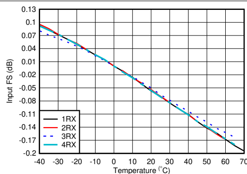
图 7-51. 800MHz 条件下 RX 输入满量程与温度和通道间的关系
