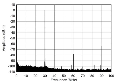
图 7-253. 30MHz 和 -6dBFS (0 - 100MHz) 条件下的单音频谱
