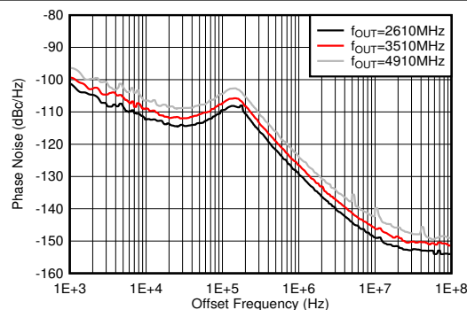
图 7-624. 25°C 条件下 9GHz VCO 相位噪声与偏移频率和 f_{OUT} 间的关系
