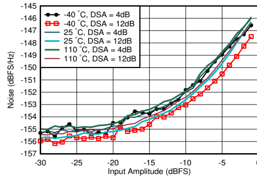
图 7-186. 4.9GHz 条件下 RX 噪声频谱密度与输入振幅和温度间的关系
