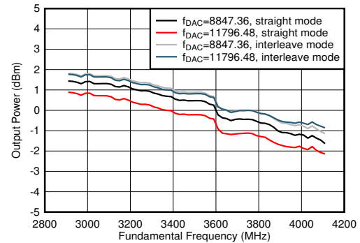
图 7-454. TX 输出功率与频率间的关系
