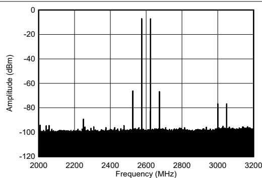
图 7-439. 2.6GHz、单音幅值为 -7dBFS ( \pm 600\text{MHz} ) 条件下的 TX 双音输出频谱
