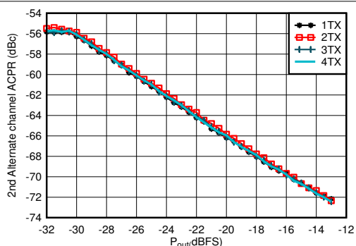
图 7-365. 1.8425GHz 条件下 TX 20MHz LTE ACPR 与数字电平间的关系
