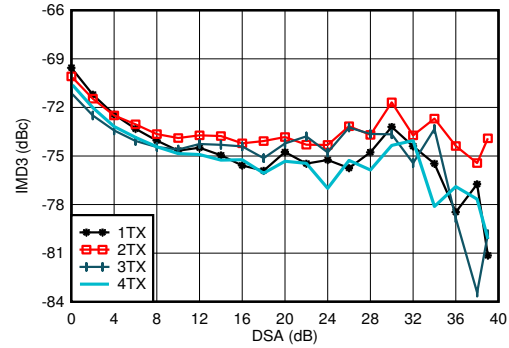
图 7-474. 3.5GHz 条件下 TX IMD3 与 DSA 设置间的关系
