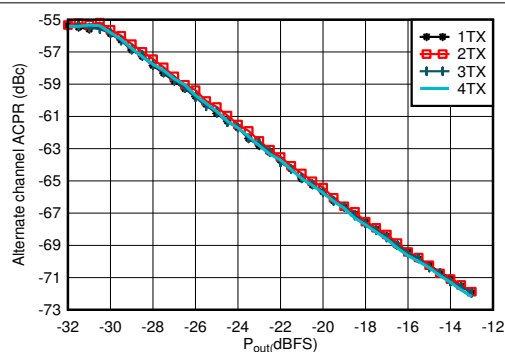
图 7-366. 1.8425GHz 条件下 TX 20MHz LTE alt-ACPR 与数字电平间的关系
