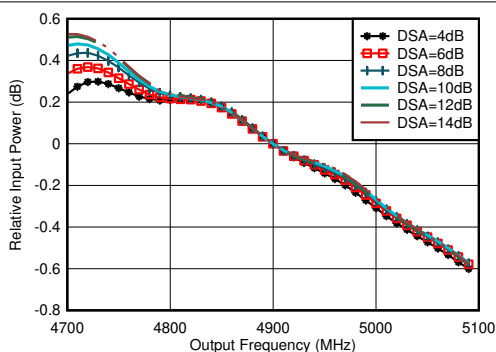
图 7-173. RX 带内增益平坦度， f_{\text{IN}} = 4900\text{MHz}
