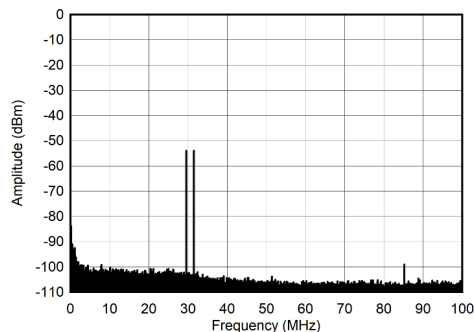
图 7-263. 30MHz 和 -60dBFS (0 - 100MHz) 条件下的双频频谱
