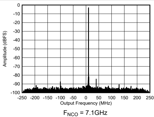
图 7-212. 7.11GHz 和 -3dBFS 条件下的单频 RX 输出 FFT
