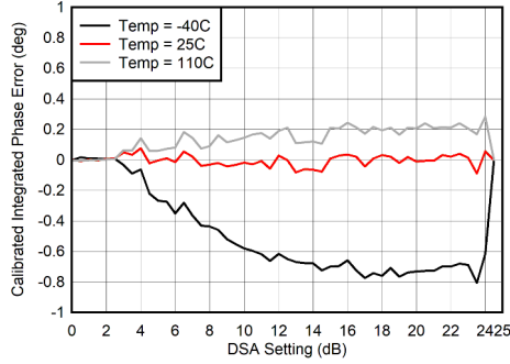
图 7-37. 400MHz 条件下 RX 校准积分相位误差与 DSA 设置间的关系
