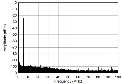
图 7-248. 5MHz 和 -30dBFS (0 - 100MHz) 条件下的单音频谱
