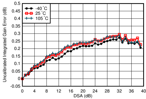
图 7-315. 0.85GHz 条件下 TX 未校准差分增益误差与 DSA 设置和温度间的关系
