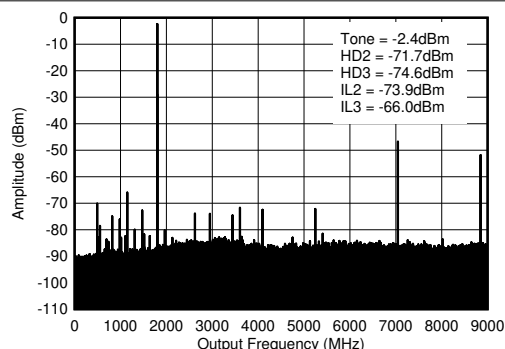
图 7-378. 1.8GHz ( 0 - f_{\text{DAC}} ) 条件下的 TX 单音 ( -12\text{dBFS} ) 输出频谱
