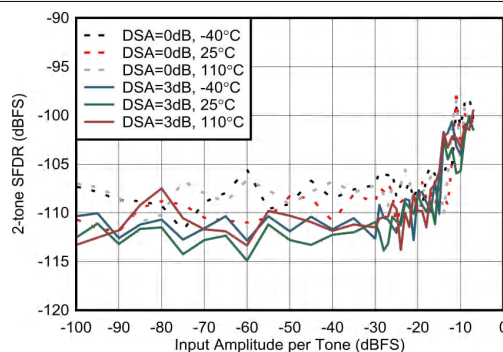
图 7-132. 2.6GHz 条件下 RX 带内 SFDR ( \pm 300\text{MHz} ) 与输入振幅和温度间的关系
