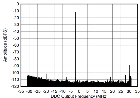
图 7-15. 30MHz 条件下的 RX 输出 FFT
