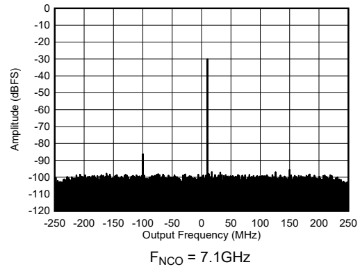
图 7-215. 7.1GHz 和 -30dBFS 条件下的单频 RX 输出 FFT
