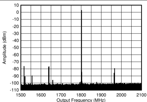
图 7-382. 1.8GHz ( 0 - f_{\text{DAC}} ) 条件下的 TX 单音 ( -1\text{dBFS} ) 输出频谱
