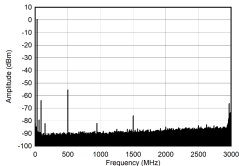
图 7-252. 30MHz 和 -6dBFS (奈奎斯特) 条件下的单音频谱
