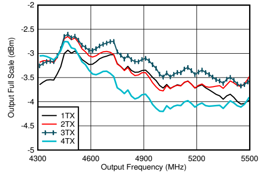
图 7-507. 5898.24MSPS、混合模式、第二奈奎斯特区域条件下 TX 满量程与射频频率和通道间的关系
