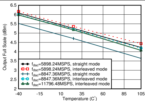
图 7-309. TX 输出满量程与温度间的关系
