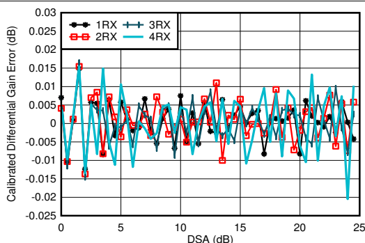
图 7-177. 4.9GHz 条件下 RX 校准差分振幅误差与 DSA 设置间的关系
