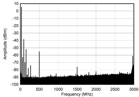
图 7-250. 30MHz 和 -1dBFS (奈奎斯特) 条件下的单音频谱
