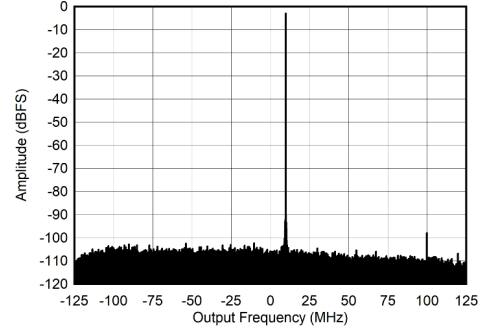
图 7-38. 405MHz 和 -3dBFS 条件下的 RX 输出 FFT
