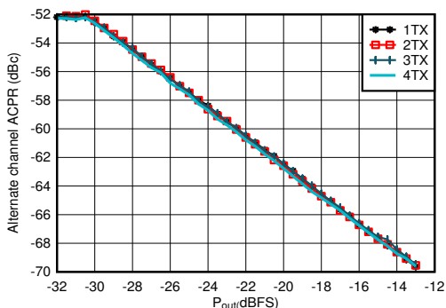
图 7-341. 0.85GHz 条件下 TX 20MHz LTE alt-ACPR 与数字电平间的关系
