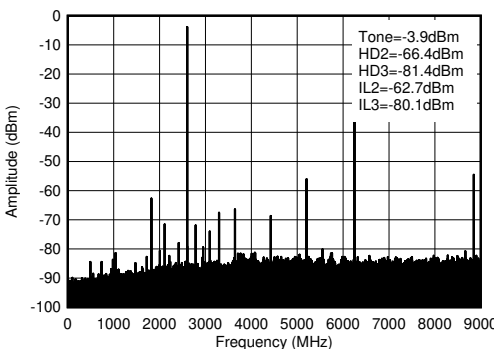
图 7-432. 2.6GHz (0 - f_{\text{DAC}} ) 条件下的 TX 单音 (-12dBFS) 输出频谱
