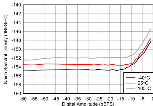
图 7-584. 7.1GHz 条件下 NSD 与数字振幅和温度间的关系
