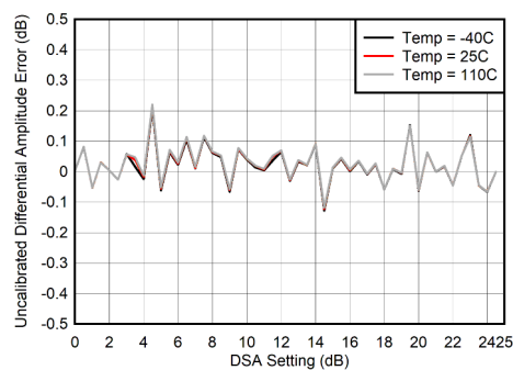
图 7-30. 30MHz 条件下 RX 未校准差分振幅误差与 DSA 设置间的关系
