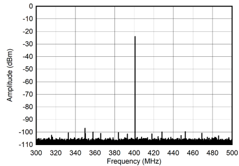
图 7-286. 400MHz 和 -30dBFS (±100MHz) 条件下的单音频谱
