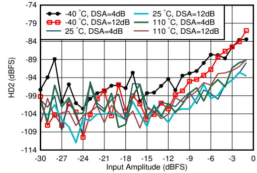
图 7-100. 1.9GHz 条件下 RX HD2 与 DSA 设置和温度间的关系
