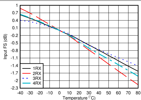
图 7-174. 4.9GHz 条件下 RX 输入满量程与温度和通道间的关系
