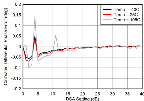
图 7-276. 400MHz 条件下的校准 TX 差分相位误差 (DNL)
