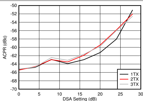
图 7-345. 0.85GHz 条件下 TX 100MHz NR ACPR 与 DSA 间的关系
