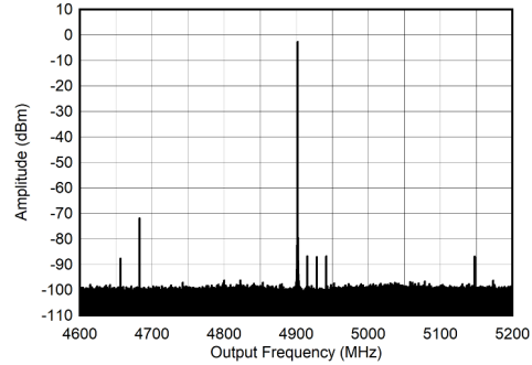
图 7-547. 4.9GHz ( \pm 300\text{MHz} ) 条件下的 TX 单音 (-1dBFS) 输出频谱
