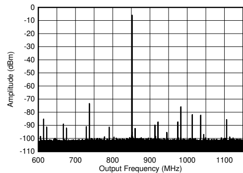
图 7-350. 0.85GHz 条件下 TX HD3 与数字振幅和输出频率间的关系
