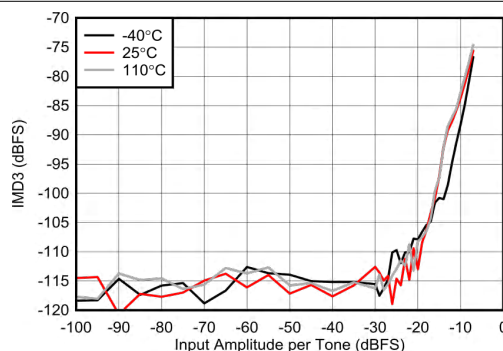
图 7-122. 2.6GHz (外部时钟) 条件下 RX IMD3 与输入电平间的关系
