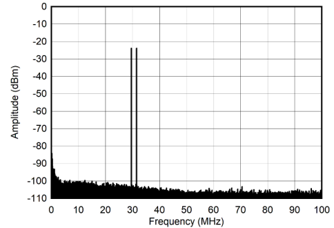
图 7-262. 30MHz 和 -30dBFS (0 - 100MHz) 条件下的双频频谱
