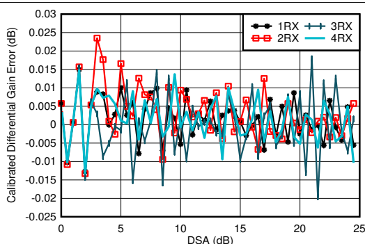
图 7-54. 0.8GHz 条件下 RX 校准差分振幅误差与 DSA 设置间的关系
