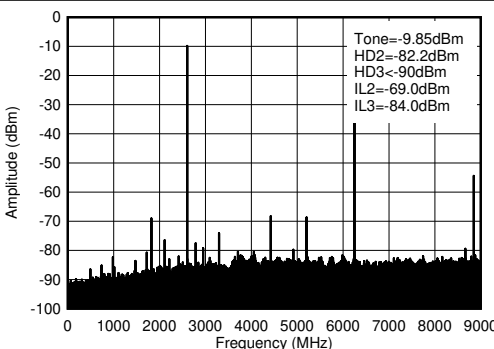
图 7-430. 2.6GHz (0- f_{\text{DAC}} ) 条件下的 TX 单音 (-1dBFS) 输出频谱
