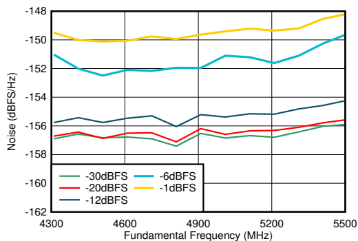
图 7-528. 4.9GHz (DSA = 0dB) 条件下 TX NSD 与输出频率和数字振幅间的关系
