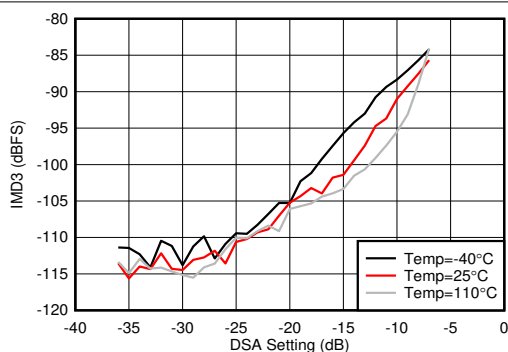
图 7-149. 3.6GHz 条件下 RX IMD3 与输入电平和温度间的关系
