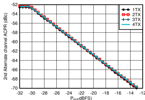
图 7-342. 0.85GHz 条件下 TX 20MHz LTE alt2-ACPR 与数字电平间的关系
