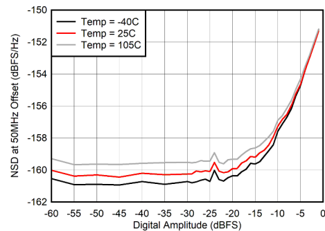
图 7-297. 400MHz 条件下的噪声频谱密度与数字振幅间的关系
