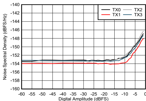
图 7-583. 7.1GHz 条件下 NSD 与数字振幅和通道间的关系
