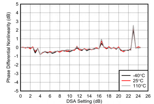
图 7-207. 6.851GHz 条件下的 RX 未校准差分相位误差
