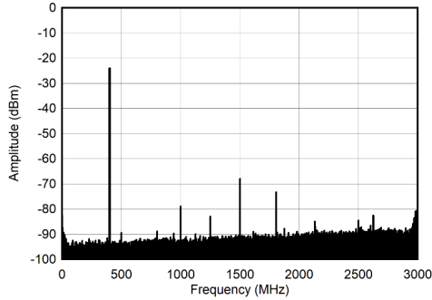
图 7-293. 400MHz 和 -30dBFS (奈奎斯特) 条件下的双频频谱
