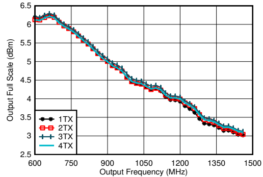
图 7-304. 8847.36MSPS 条件下 TX 满量程与射频频率和通道间的关系, 直接模式
