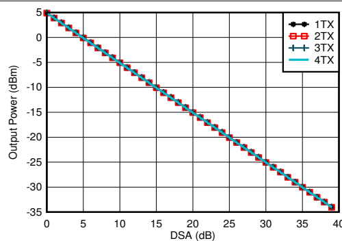
图 7-310. 0.85GHz 条件下 TX 输出功率与 DSA 设置和通道间的关系
