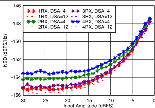
图 7-117. 2.6GHz 条件下 RX 噪声频谱密度与输入振幅和通道间的关系
