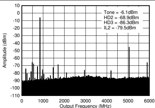
图 7-355. 0.85GHz (0- f_{\text{DAC}} ) 条件下的 TX 单音 (-1dBFS) 输出频谱
