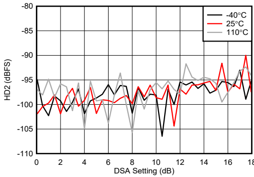
图 7-228. 6.851GHz 条件下 RX HD2 与 DSA 设置间的关系
