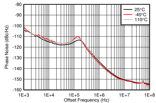
图 7-610. f_{OUT} = 2.6\text{GHz} 时 12GHz VCO 相位噪声 (5MHz 偏移条件下) 与温度和 f_{REF} 间的关系
