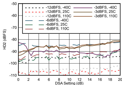
图 7-26. 30MHz 条件下 HD2 与 DSA 设置间的关系
