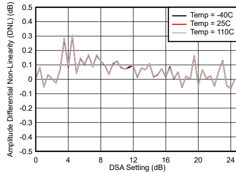
图 7-2. 30MHz 条件下 RX 未校准差分振幅误差与 DSA 设置间的关系
