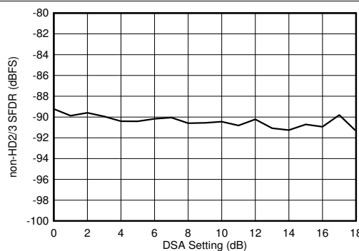
图 7-133. 2.6GHz 条件下 Rx 非 HD2/3 与 DSA 设置间的关系
