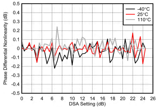
图 7-208. 6.851GHz 条件下的 RX 校准差分相位误差
