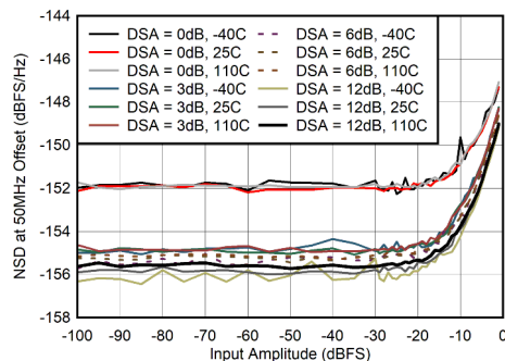
图 7-43. 400MHz 条件下 NSD 与输入振幅间的关系
