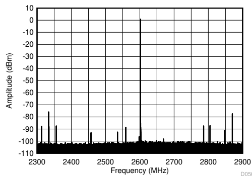
图 7-437. 2.6GHz ( \pm 300\text{MHz} ) 条件下的 TX 单音 (-1dBFS) 输出频谱
