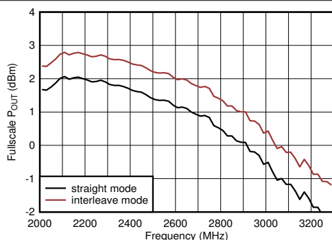
图 7-384. 5898.24MSPS 条件下 TX 满量程与射频频率间的关系
