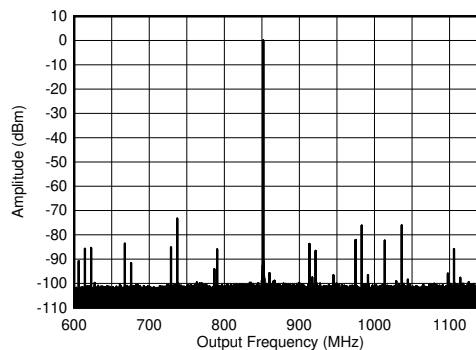
图 7-354. 0.85GHz ( \pm 300\text{MHz} ) 条件下的 TX 单音 (-6dBFS) 输出频谱
