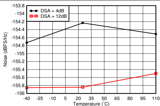
图 7-62. 0.8GHz 条件下 RX 噪声频谱密度与温度间的关系
