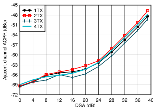
图 7-540. 4.9GHz 条件下 TX 20MHz LTE ACPR 与 DSA 间的关系
