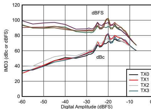
图 7-572. 7.1GHz 条件下 IMD3 与数字振幅和通道间的关系
