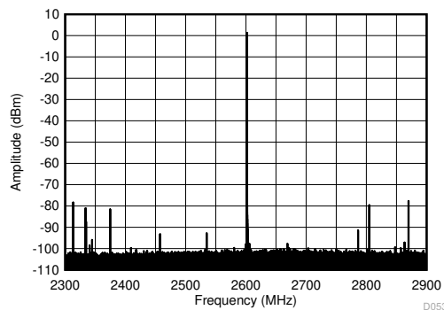
图 7-431. 2.6GHz ( \pm 300\text{MHz} ) 条件下的 TX 单音 (-1dBFS) 输出频谱
