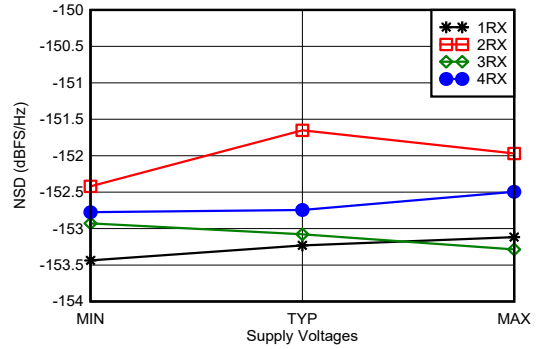
图 7-136. 2.6GHz 条件下 RX 噪声频谱密度与电源和通道间的关系
