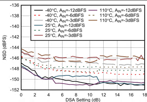
图 7-224. 6.851GHz 条件下 RX NSD 与 DSA 设置间的关系
