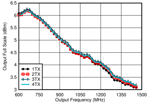
图 7-303. 5898.24MSPS 条件下 TX 满量程与射频频率和通道间的关系, 直接模式
