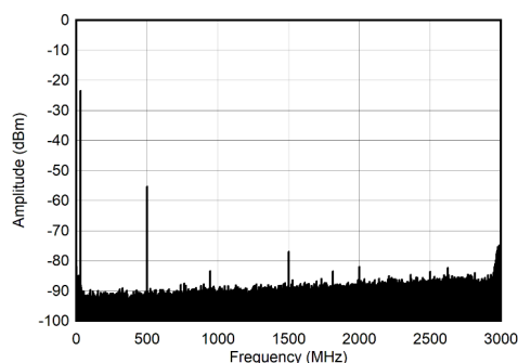
图 7-256. 30MHz 和 -30dBFS (奈奎斯特) 条件下的单音频谱
