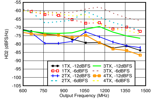
图 7-348. 0.85GHz 条件下 TX HD2 与数字振幅和输出频率间的关系
