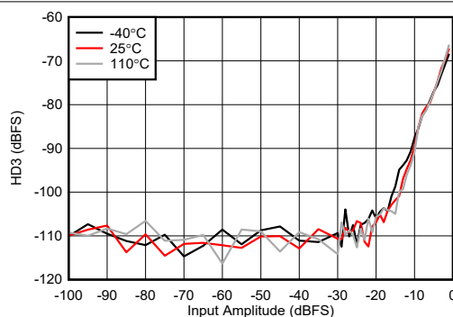
图 7-162. 3.76GHz 条件下 RX HD3 与输入电平间的关系
