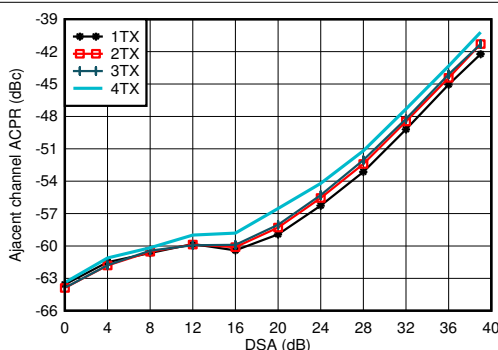
图 7-542. 4.9GHz 条件下 TX 100MHz NR ACPR 与 DSA 间的关系
