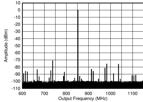
图 7-360. 0.85GHz ( \pm 300\text{MHz} ) 条件下的 TX 单音 (-6dBFS) 输出频谱
