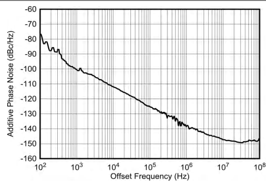
图 7-596. 7.1GHz 条件下的外部时钟附加相位噪声
