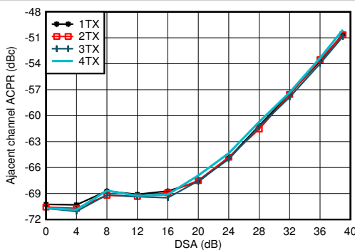
图 7-483. 3.5GHz 条件下的 TX 20MHz LTE ACPR 与 DSA 设置间的关系
