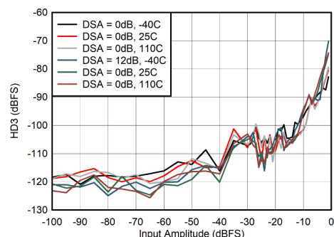
图 7-48. 400MHz 条件下 HD3 与输入振幅间的关系
