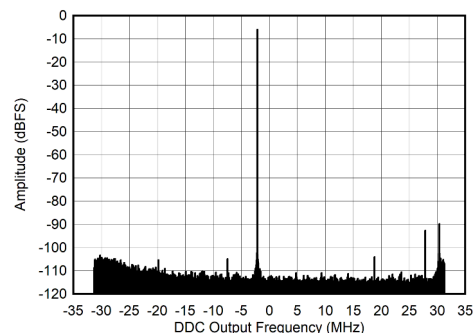
图 7-14. 5MHz 条件下的 RX 输出 FFT
