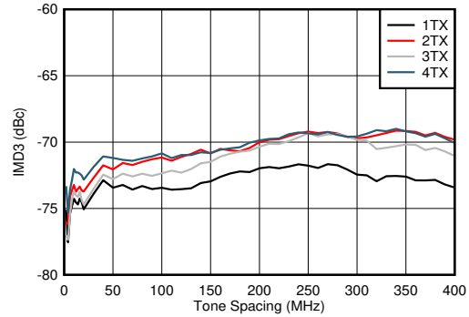
图 7-407. 2.6GHz 条件下 TX IMD3 与频率间隔和通道间的关系
