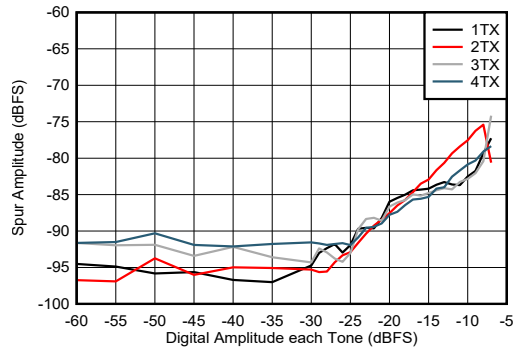
图 7-479. 3.75GHz 条件下双频带内 SFDR 与数字振幅间的关系
