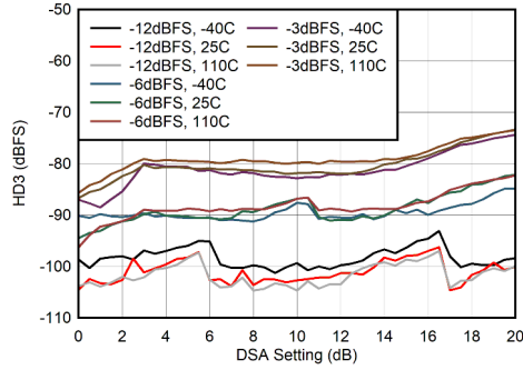
图 7-49. 400MHz 条件下 HD3 与 DSA 设置间的关系
