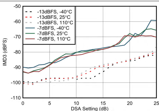
图 7-222. 6.851GHz 条件下 RX IMD3 与 DSA 设置间的关系
