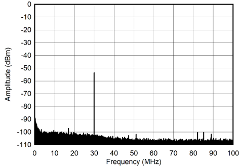
图 7-259. 30MHz 和 -60dBFS (0 - 100MHz) 条件下的单音频谱
