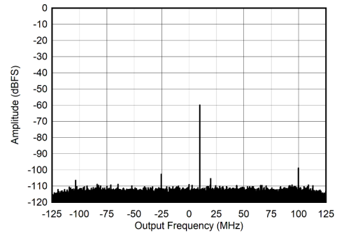
图 7-42. 405MHz 和 -60dBFS 条件下的 RX 输出 FFT
