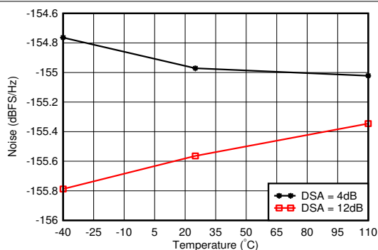
图 7-93. 1.75GHz 条件下 RX 噪声频谱密度与温度间的关系
