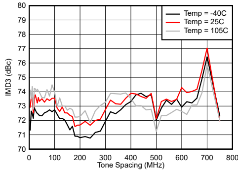
图 7-579. 7.1GHz 条件下 IMD3 与频率间隔和温度间的关系
