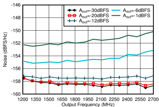
图 7-363. 1.8GHz 条件下 TX 单音输出噪声与频率和振幅间的关系
