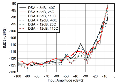
图 7-45. 400MHz 条件下 IMD3 与输入振幅间的关系
