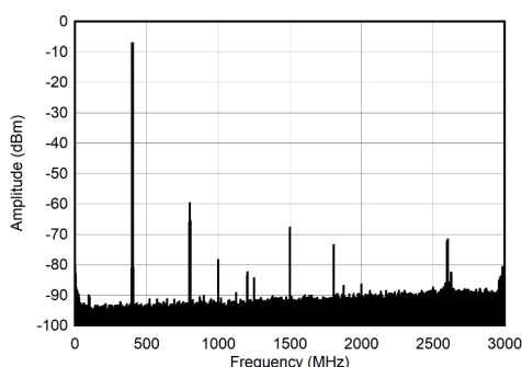
图 7-289. 400MHz 和 -7dBFS (奈奎斯特) 条件下的双频频谱
