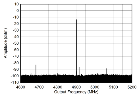
图 7-549. 4.9GHz ( \pm 300\text{MHz} ) 条件下的 TX 单音 (-6dBFS) 输出频谱
