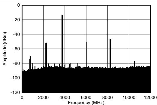
图 7-499. 3.75GHz、单音幅值为 -7dBFS (0 - f_{\text{DAC}} ) 条件下的 TX 双音输出频谱
