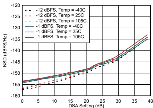
图 7-265. 30MHz 条件下的噪声频谱密度与 DSA 设置间的关系
