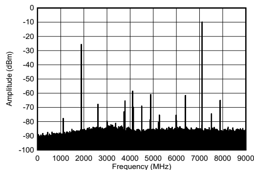
图 7-586. 7.1GHz、-1dBFS (0 - F_{\text{DAC}} ) 条件下的单音输出频谱
