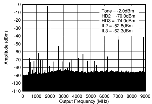
图 7-372. 1.8GHz (0 - f_{\text{DAC}} ) 条件下的 TX 单音 (-12dBFS) 输出频谱
