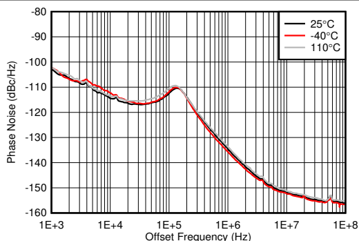
图 7-621. f_{OUT} = 2.6\text{GHz} 时 10GHz VCO 相位噪声 (5MHz 条件下) 与温度和 f_{REF} 间的关系
