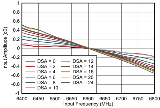
图 7-202. RX 带内增益平坦度
