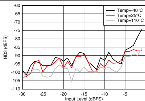
图 7-130. 2.6GHz 条件下 RX HD3 与输入电平和温度间的关系
