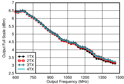
图 7-303. 5898.24MSPS 条件下 TX 满量程与射频频率和通道间的关系, 直接模式
