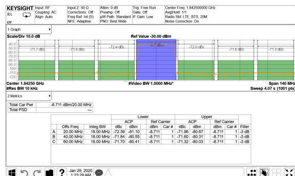
图 7-364. 1.8425GHz 条件下的 TX 20MHz LTE 输出频谱
