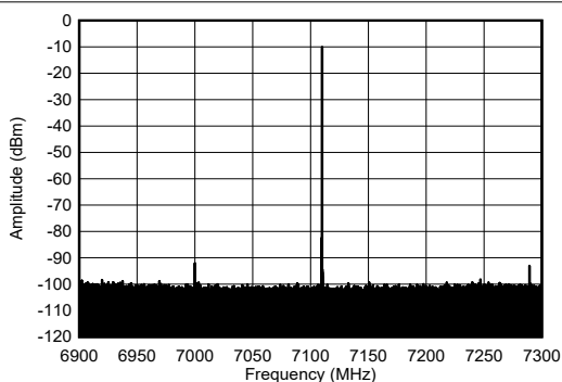
图 7-587. 7.1GHz、-1dBFS (带内) 条件下的单音输出频谱
