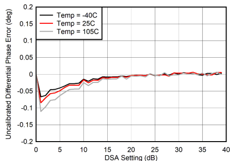
图 7-275. 400MHz 条件下的未校准 TX 差分相位误差 (DNL)
