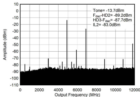
图 7-548. 4.9GHz (0 - f_{\text{DAC}} ) 条件下的 TX 单音 (-6dBFS) 输出频谱
