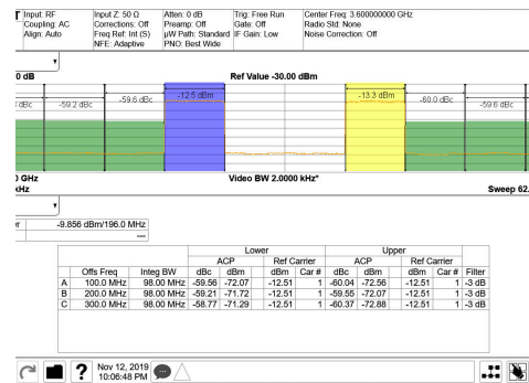
图 7-482. 3.45GHz 和 3.75GHz 条件下的 TX 2 载波 100MHz NR 输出频谱
