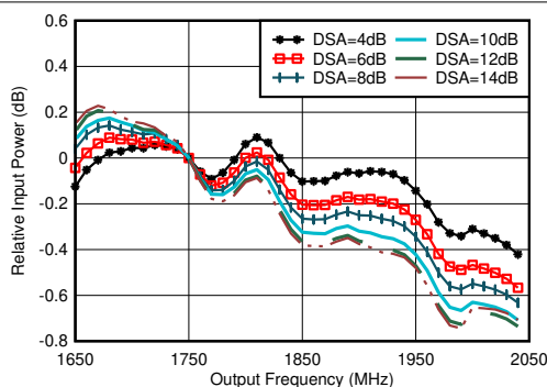
图 7-81. RX 带内增益平坦度， f_{\text{IN}} = 1750\text{MHz}
