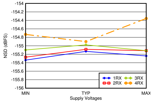
图 7-80. 0.8GHz 条件下 RX 噪声频谱密度与电源和通道间的关系
