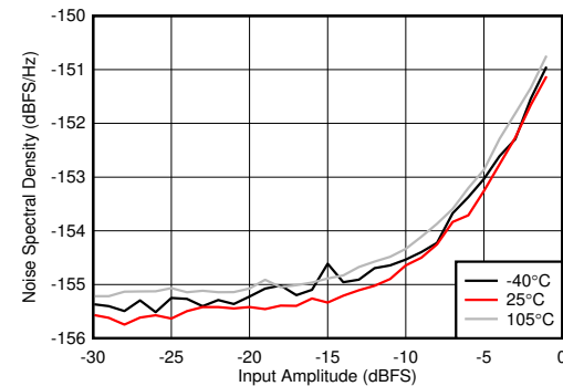
图 7-116. 2.6GHz 条件下 RX 噪声频谱密度与输入振幅和温度间的关系
