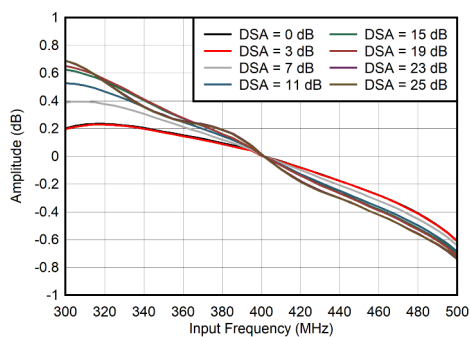
图 7-29. RX 带内增益平坦度， f_{\text{IN}} = 400\text{MHz}
