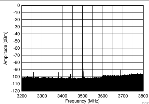
图 7-494. 3.5GHz ( \pm 300\text{MHz} ) 条件下的 TX 单音 (-1dBFS) 输出频谱
