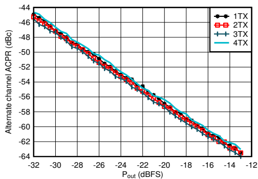
图 7-536. 4.9GHz 条件下 TX 20MHz LTE ACPR 与数字电平间的关系
