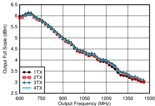
图 7-305. 5898.24MSPS 条件下 TX 满量程与射频频率和通道间的关系, 交错模式
