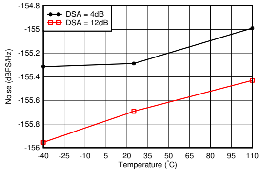
图 7-185. 4.9GHz 条件下 RX 噪声频谱密度与温度间的关系
