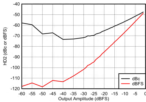
图 7-301. 400MHz 条件下 HD2 与振幅间的关系
