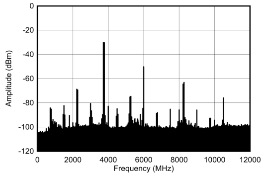
图 7-503. 3.75GHz、单音幅值为 -30dBFS ( 0 - f_{\text{DAC}} ) 条件下的 TX 双音输出频谱
