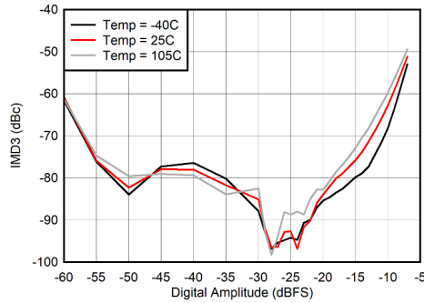
图 7-299. 400MHz 条件下 IMD3 与数字振幅间的关系
