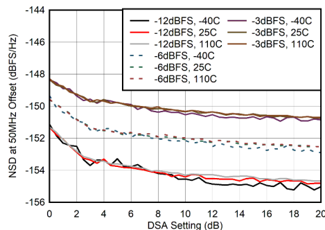
图 7-44. 400MHz 条件下 NSD 与 DSA 设置间的关系
