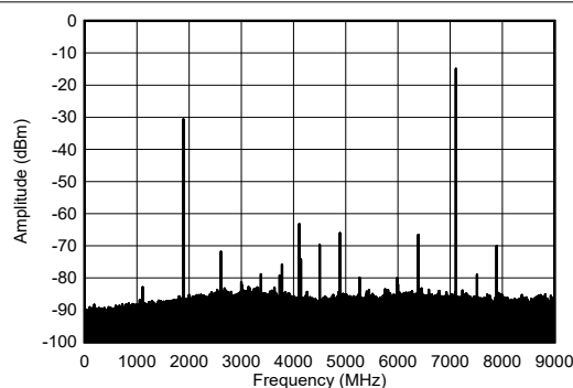
图 7-588. 7.1GHz、-6dBFS (0 - F_{\text{DAC}} ) 条件下的单音输出频谱
