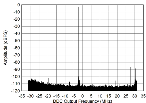
图 7-13. 5MHz 条件下的 RX 输出 FFT
