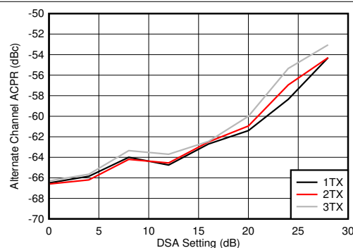
图 7-344. 0.85GHz 条件下 TX 20MHz LTE alt-ACPR 与 DSA 间的关系
