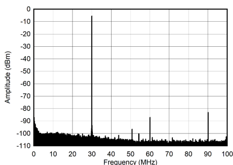
图 7-255. 30MHz 和 -12dBFS (0 - 100MHz) 条件下的单音频谱
