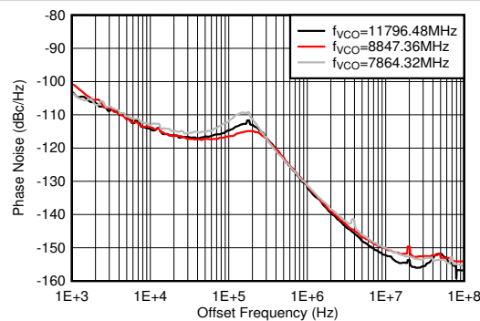
图 7-597. 12GHz 条件下 PLL 和外部时钟的相位噪声与偏移频率间的关系
