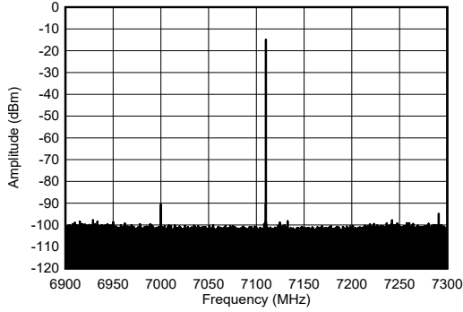
图 7-589. 7.1GHz、-6dBFS (带内) 条件下的单音输出频谱
