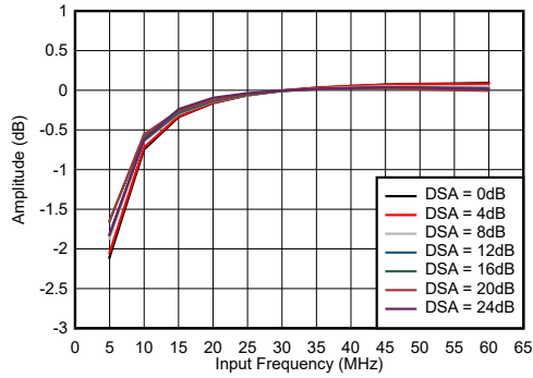
图 7-1. RX 带内增益平坦度， f_{\text{IN}} = 30\text{MHz}
