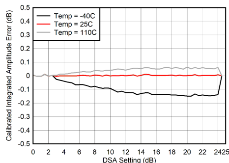
图 7-33. 400MHz 条件下 RX 校准积分振幅误差与 DSA 设置间的关系
