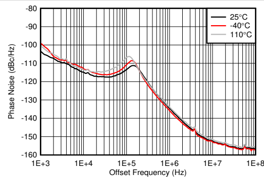
图 7-600. f_{\text{OUT}} = 1910\text{MHz} 时 12GHz VCO 相位噪声与偏移频率和温度间的关系
