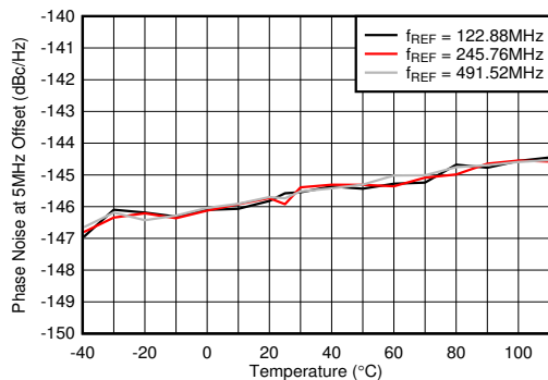
图 7-621. f_{OUT} = 2.6\text{GHz} 时 10GHz VCO 相位噪声 (5MHz 条件下) 与温度和 f_{REF} 间的关系
