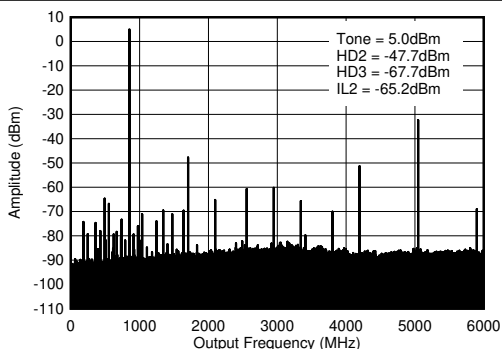
图 7-353. 0.85GHz (0- f_{\text{DAC}} ) 条件下的 TX 单音 (-6dBFS) 输出频谱
