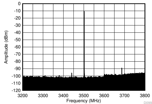
图 7-498. 3.5GHz ( \pm 300\text{MHz} ) 条件下的 TX 单音 (-12dBFS) 输出频谱
