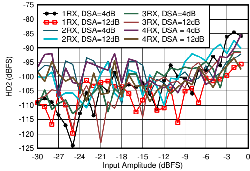
图 7-99. 1.9GHz 条件下 RX HD2 与 DSA 设置和通道间的关系
