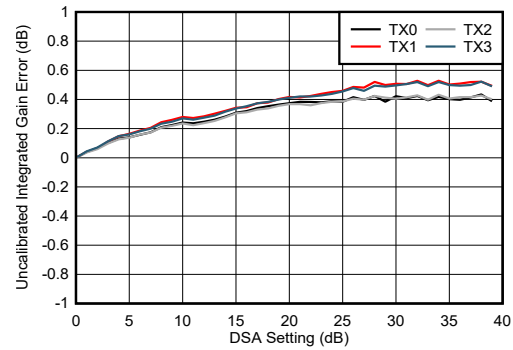
图 7-560. 7.1GHz 条件下未校准积分增益误差与通道间的关系
