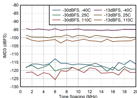
图 7-47. 400MHz 条件下 IMD3 与子载波间隔间的关系
