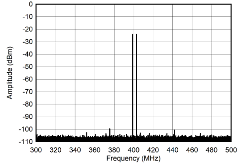
图 7-294. 400MHz 和 -30dBFS (±100MHz) 条件下的双频频谱
