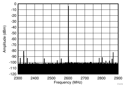
图 7-433. 2.6GHz ( \pm 300\text{MHz} ) 条件下的 TX 单音 (-12dBFS) 输出频谱
