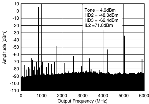
图 7-359. 0.85GHz (0- f_{\text{DAC}} ) 条件下的 TX 单音 (-6dBFS) 输出频谱
