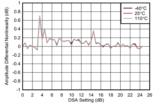
图 7-203. 6.851GHz 条件下的 RX 未校准差分振幅误差
