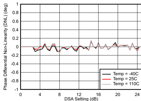
图 7-7. 30MHz 条件下 RX 校准差分相位误差与 DSA 设置间的关系
