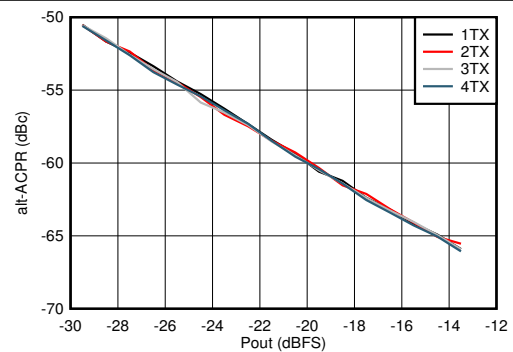
图 7-415. 2.6GHz 条件下 TX 20MHz LTE alt2-ACPR 与数字电平间的关系
