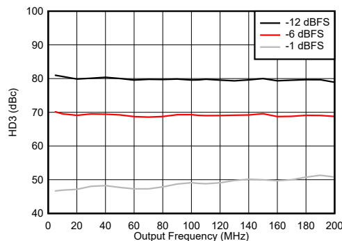
图 7-268. HD3 与频率 (0 - 200MHz) 间的关系
