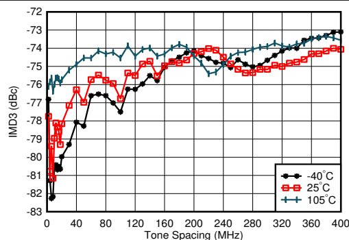
图 7-332. 0.85GHz 条件下 TX IMD3 与频率间隔和温度间的关系
