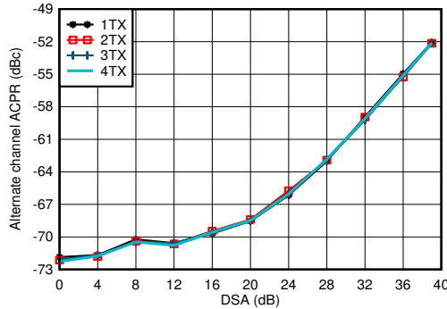
图 7-369. 1.8GHz 条件下 TX 20MHz LTE alt-ACPR 与 DSA 间的关系
