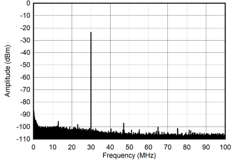
图 7-257. 30MHz 和 -30dBFS (0 - 100MHz) 条件下的单音频谱
