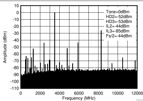
图 7-493. 3.5GHz (0 - f_{\text{DAC}} ) 条件下的 TX 单音 (-1dBFS) 输出频谱
