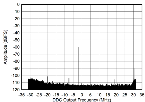
图 7-19. 30MHz 条件下的 RX 输出 FFT
