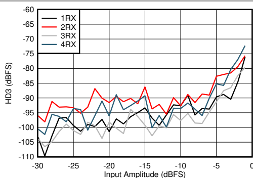
图 7-129. 2.6GHz 条件下 RX HD3 与输入电平和通道间的关系
