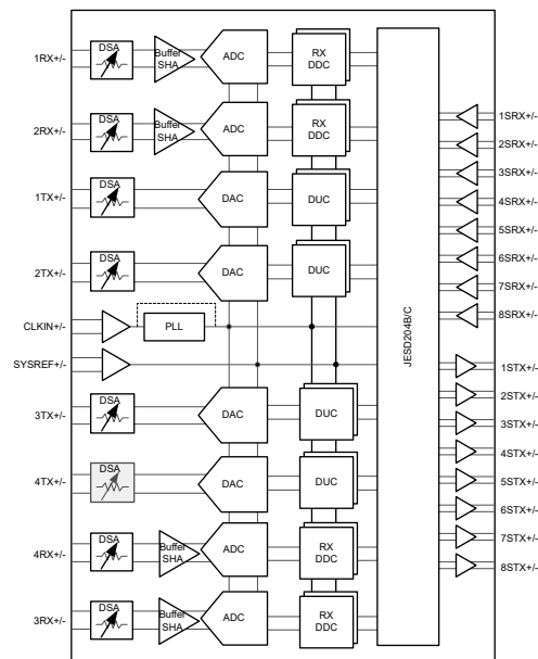
功能方框图
