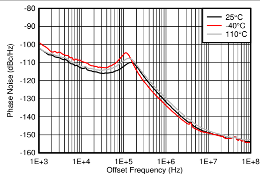
图 7-628. f_{OUT} = 1910\text{MHz} 时 8GHz VCO 相位噪声与偏移频率和温度间的关系
