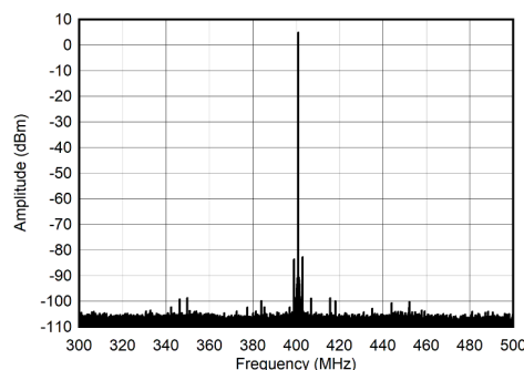
图 7-280. 400MHz 和 -1dBFS (±100MHz) 条件下的单音频频谱
