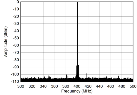
图 7-282. 400MHz 和 -6dBFS (±100MHz) 条件下的单音频谱
