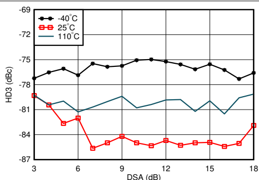
图 7-74. 0.8GHz 条件下 RX HD3 与 DSA 设置和温度间的关系
