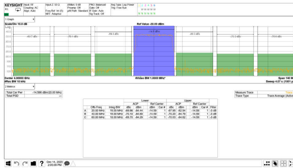
图 7-534. 4.9GHz 条件下的 TX 20MHz LTE 输出频谱
