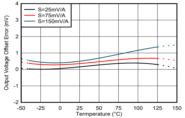
图 6-4. 偏移量误差与温度间的关系：TMCS1133Cxx 器件选项
