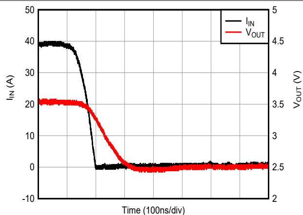
图 6-12. 电压输出阶跃响应 (下降)
