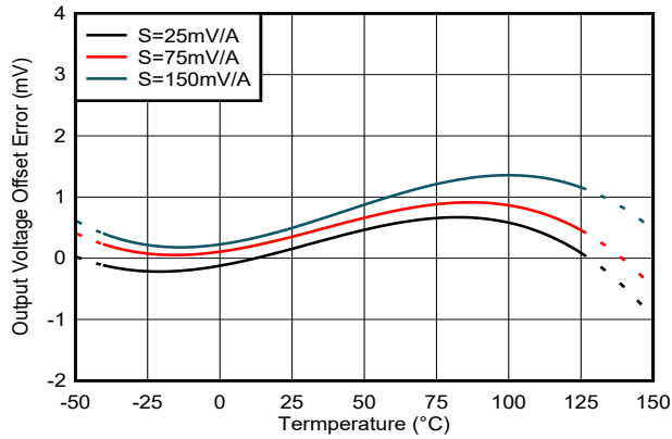
图 6-3. 偏移量误差与温度间的关系：TMCS1133Bxx 器件选项
