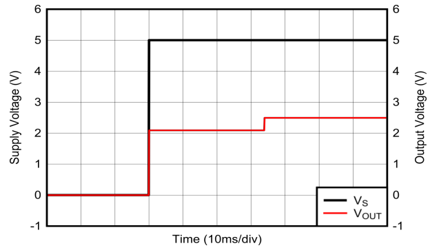
图 6-14. 启动瞬态响应
