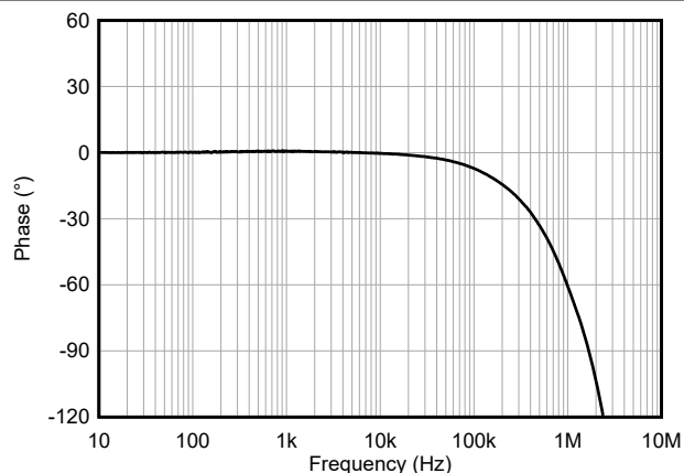
图 6-8. 相位与频率间的关系 (所有增益)
