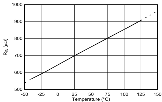
图 6-17. 输入导体电阻与温度间的关系
