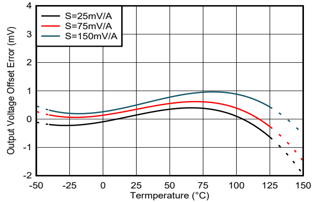
图 6-2. 偏移量误差与温度间的关系：TMCS1133Axx 器件选项
