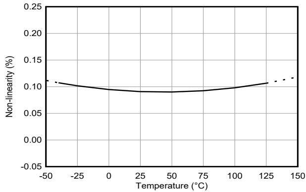
图 6-5. 非线性与温度间的关系
