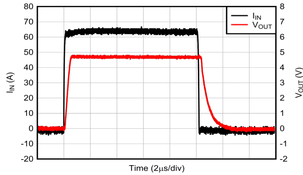
图 6-13. 电流过载响应
