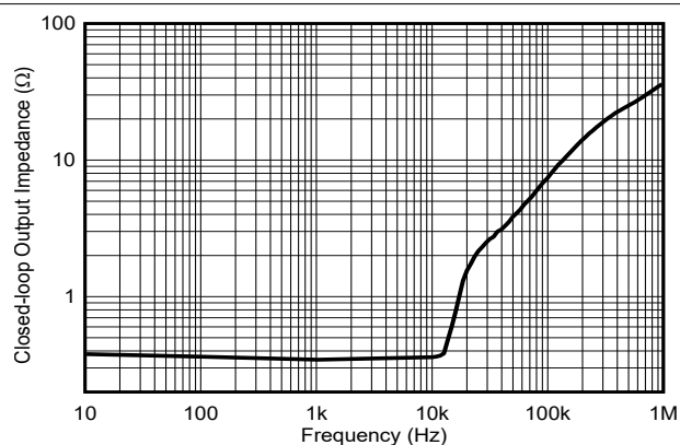
图 6-10. 输出阻抗与频率间的关系
