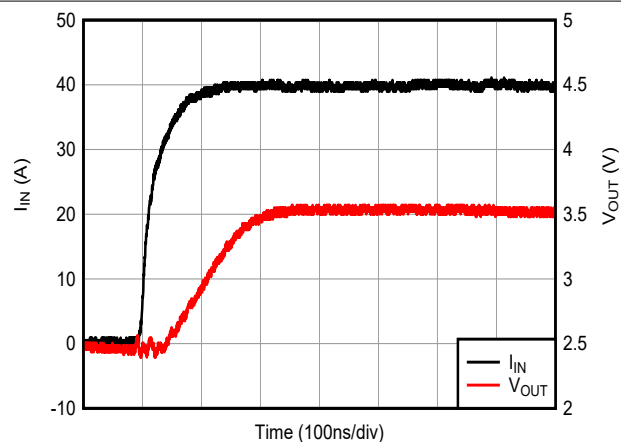
图 6-11. 电压输出阶跃响应 (上升)
