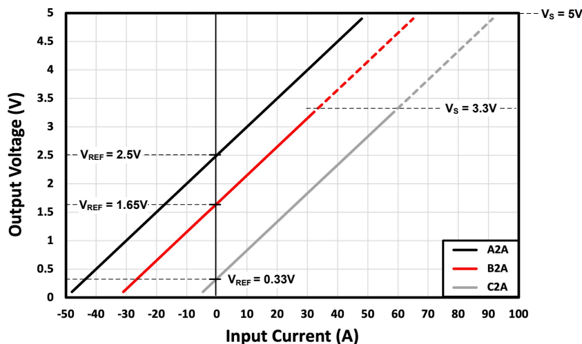
图 8-4. TMCS1126x2A-Q1 的输出电压与输入电流之间的关系
