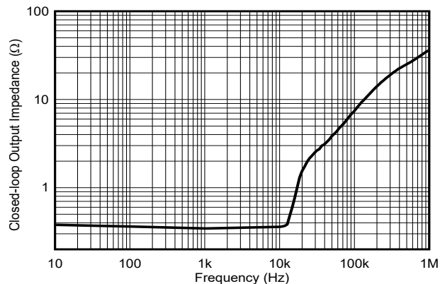
图 6-8. 输出阻抗与频率间的关系
