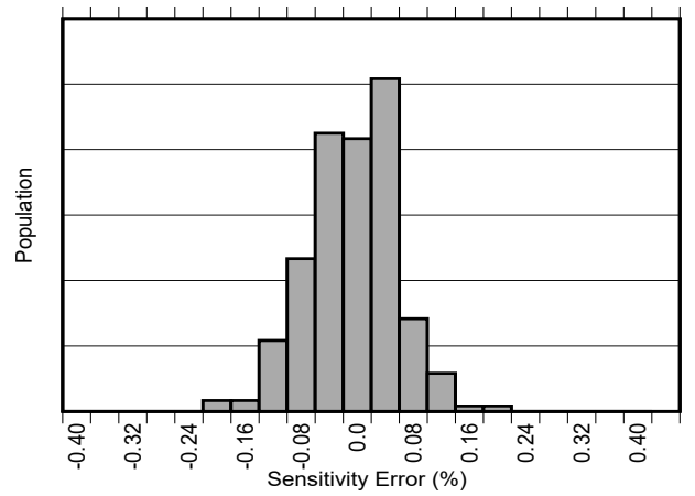
图 6-4. 灵敏度误差产生分布图：A 级
