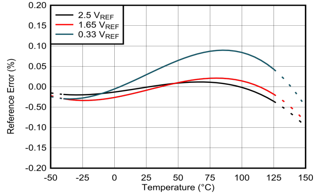
图 6-2. 基准误差与温度间的关系
