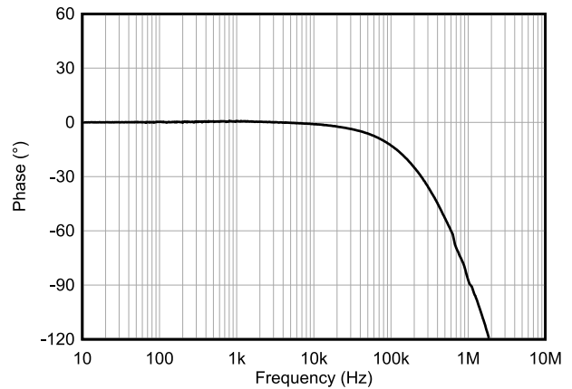
图 6-6. 相位与频率间的关系 (所有增益)
