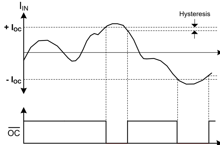
图 8-7. 过流检测图
