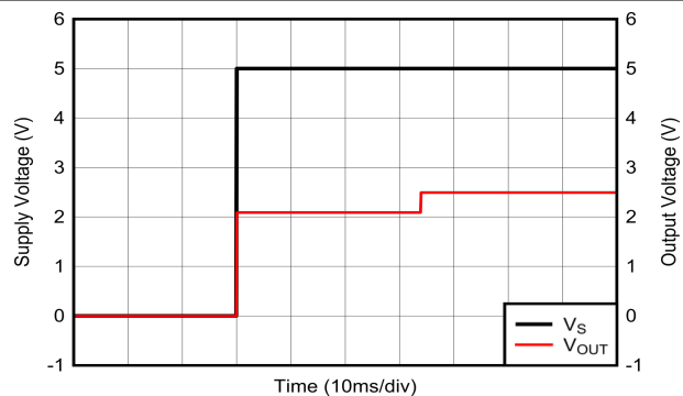
图 6-12. 启动瞬态响应
