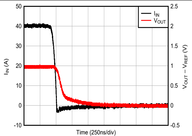
图 6-10. 电压输出阶跃响应 (下降)
