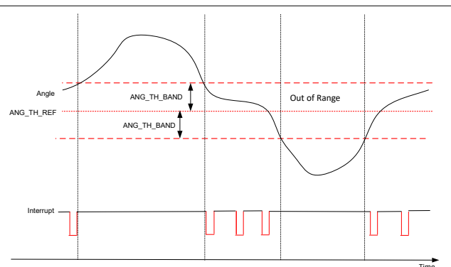
图 7-9. MAG_THR_DIR = 1b、THR_SEL=01b、INT_STATE=1b 时的角度限值交叉检查
