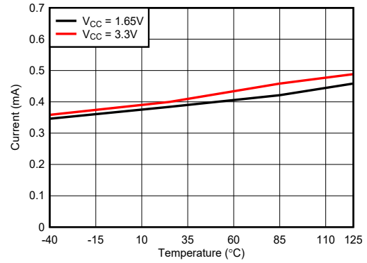
图 5-3. I_{STANDBY} 与温度间的关系
