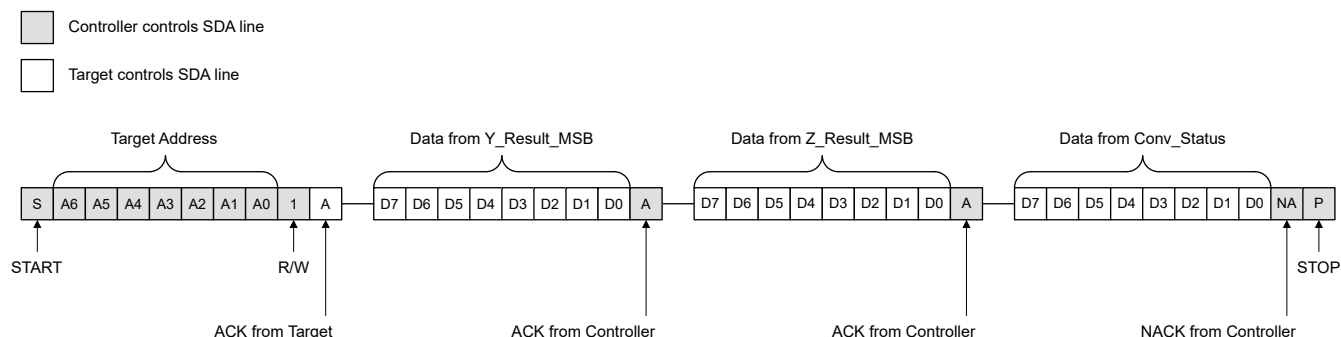
图 6-23. 禁用 CRC、启用 Y 和 Z 轴时 8 位数据的 I 2 C 读取命令
