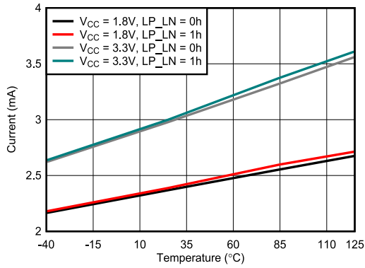
图 5-2. I_{ACTIVE} 与温度间的关系
