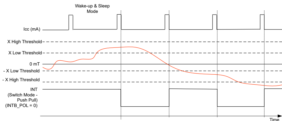
图 6-7. 通过 \overline{INT} 实现全极开关
