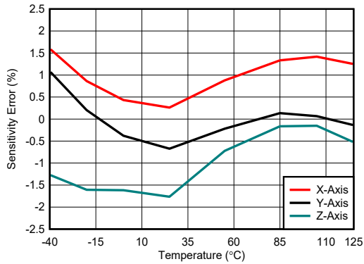
图 5-6. A2 灵敏度误差与温度间的关系, V_{CC} = 3.3V
