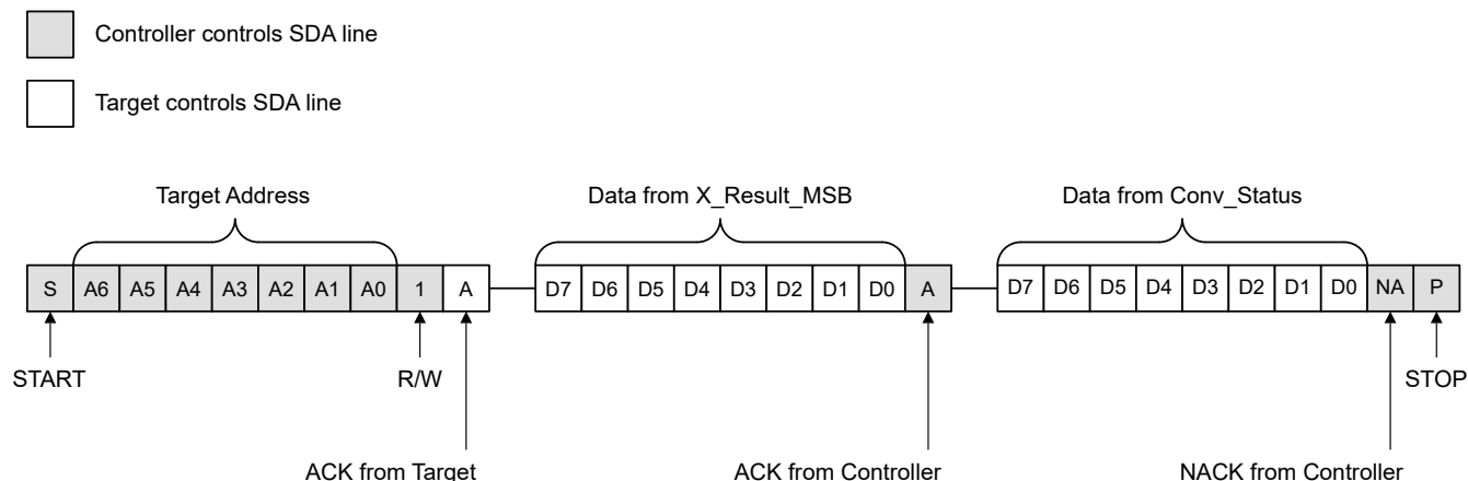
图 6-22. 禁用 CRC、启用 X 轴时 8 位数据的 I 2 C 读取命令
