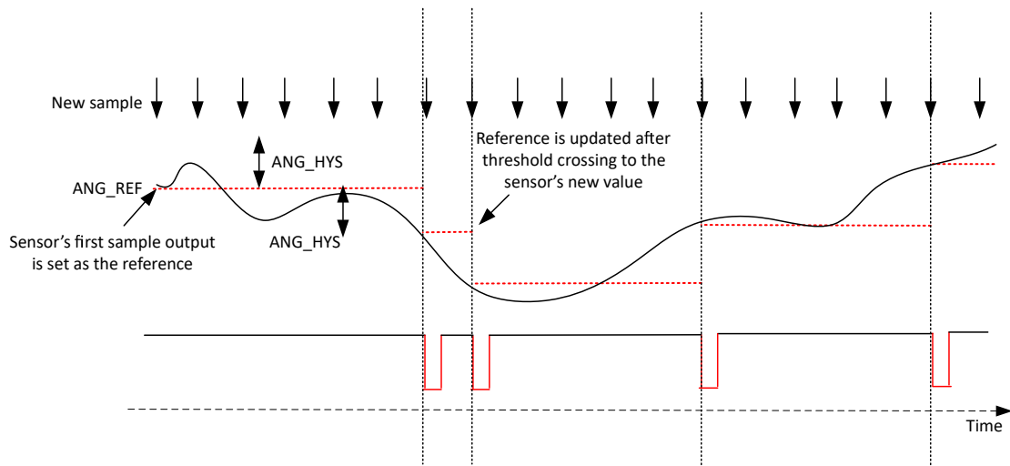
图 6-9. 角度测量的变化时唤醒，WOC_SEL = 1h，INT_State = 1h
