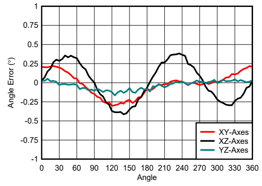
图 5-7. A2 角度误差与角度间的关系, V_{CC} = 3.3V , T_A = 25^\circ C
