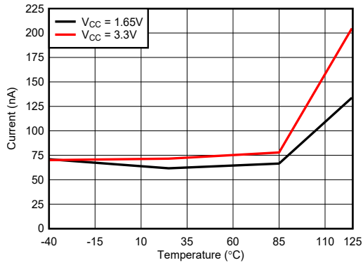
图 5-4. I_{SLEEP} 与温度间的关系
