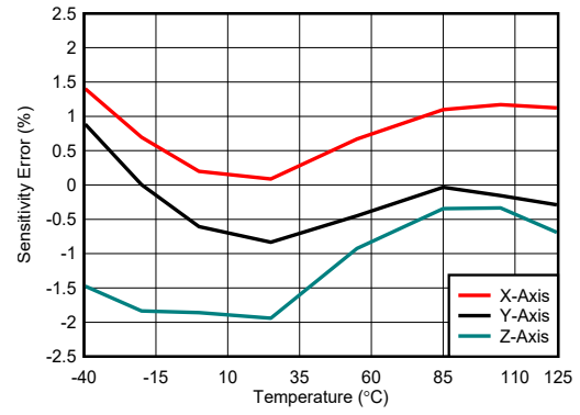
图 5-5. A2 灵敏度误差与温度间的关系, V_{CC} = 1.8V
