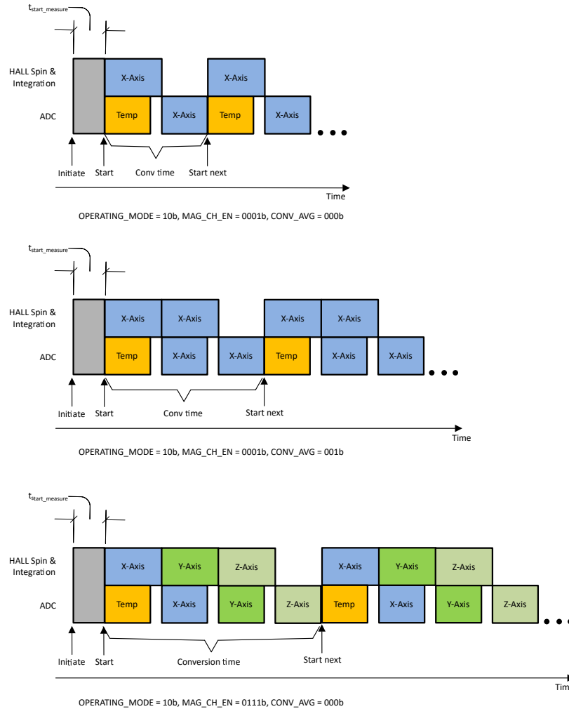
图 7-1. 连续转换模式
