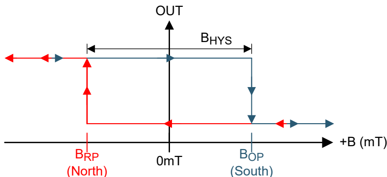
图 7-3. 双极锁存低电平有效功能
