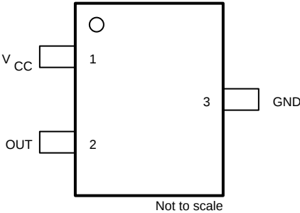
图 5-1. DBZ 封装（预发布），3 引脚 SOT-23（顶视图）
