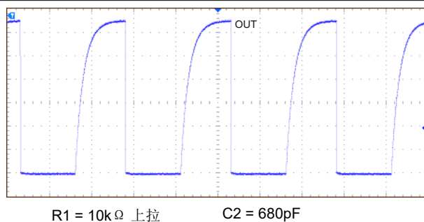
图 8-3. 10kHz 开关磁场
