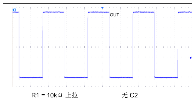
图 8-2. 10kHz 开关磁场
