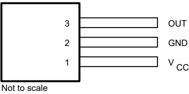
图 5-2. LPG 封装，3 引脚 To-92（顶视图）
