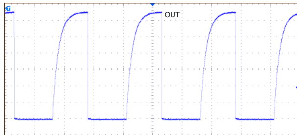
图 9-3. 10-kHz Switching Magnetic Field
