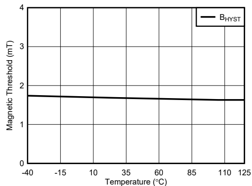
图 7-4. TMAG5115A B_{HYS} vs T_A
