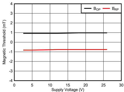
图 7-3. TMAG5115A B_{OP} and B_{RP} vs V_{CC}
