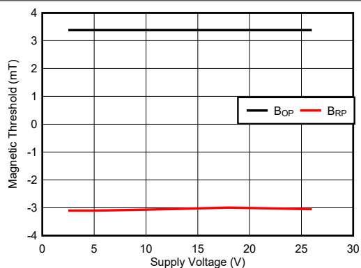
图 7-7. TMAG5115B B OP and B RP vs V CC
