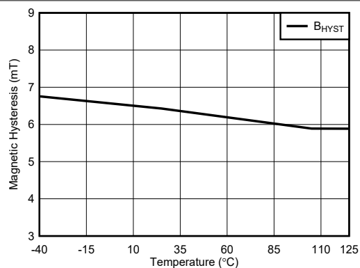
图 7-8. TMAG5115B B HYST vs T A
