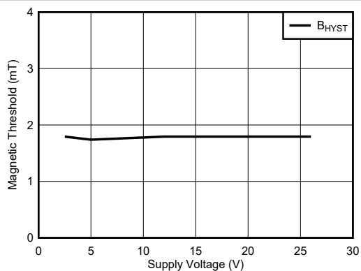
图 7-5. TMAG5115A B_{HYS} vs V_{CC}
