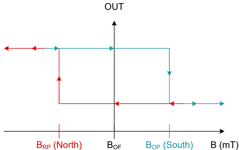
图 8-2. TMAG5115 B_{OP} > 0
