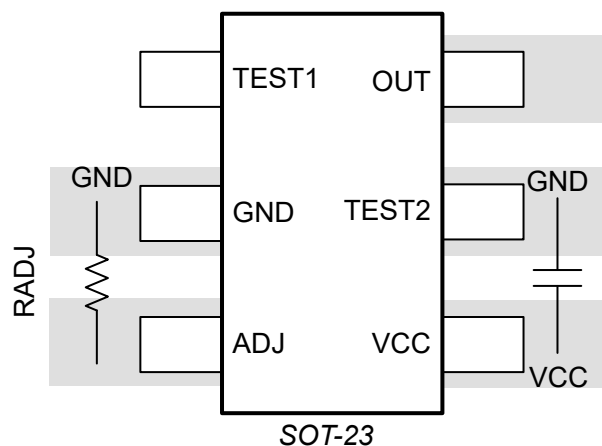
图 7-9. SOT-23 Layout Example
