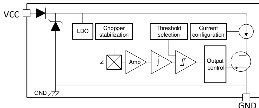
图 8-1. Block Diagram
