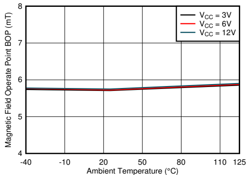
图 7-7. BOP vs. Temperature
