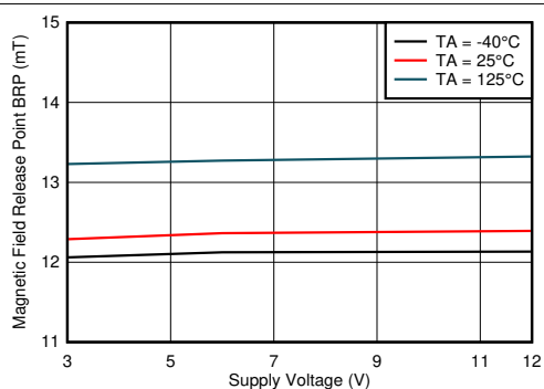
图 7-22. B_{RP} vs. V_{CC}
