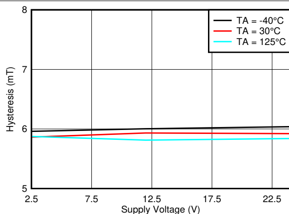
图 7-43. Hysteresis_Z 与 V CC
