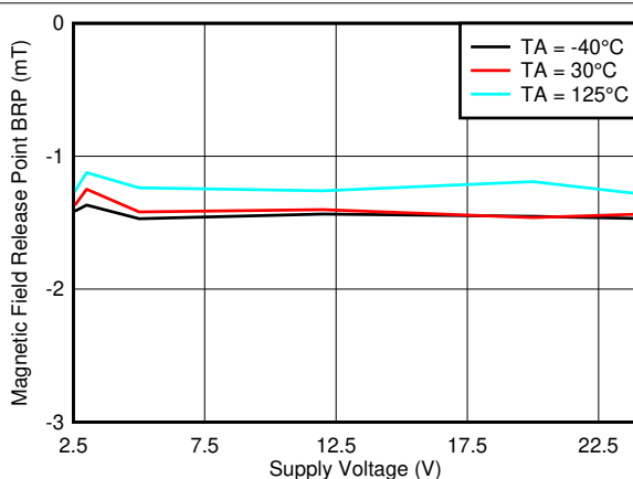
图 7-9. BRP_X 阈值与 VCC
