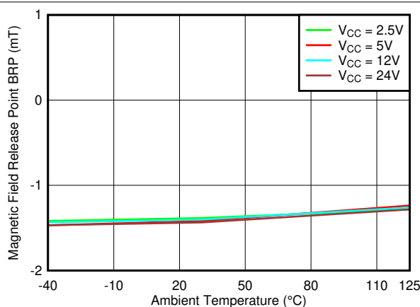
图 7-10. BRP_X 阈值与温度
