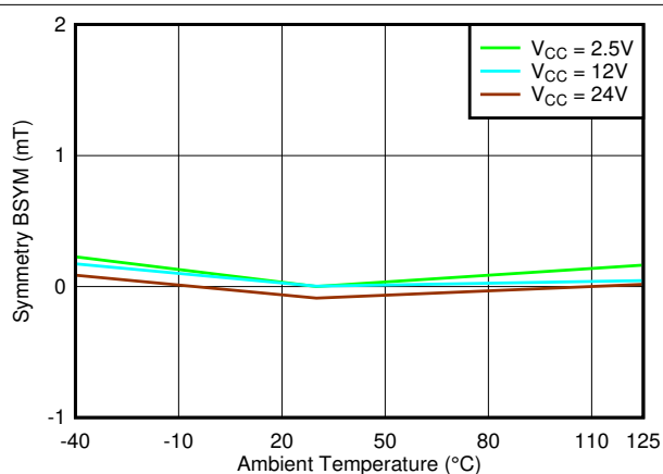
图 7-62. B_{SYM(Y)} 与温度
