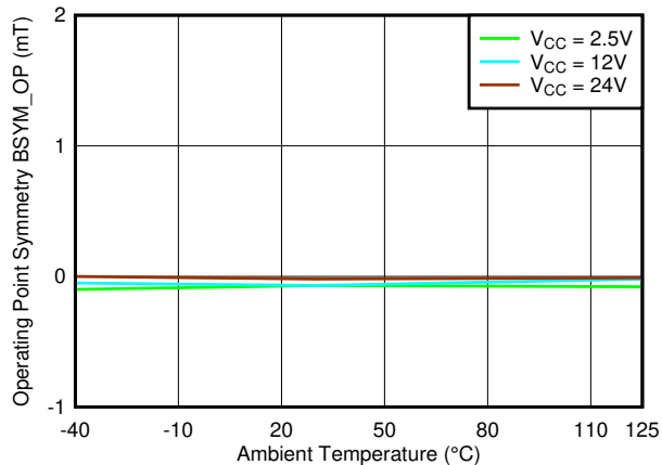
图 7-34. B_{SYM\_OP(XY)} 与温度
