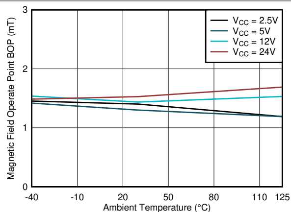
图 7-8. BOP_X 阈值与温度
