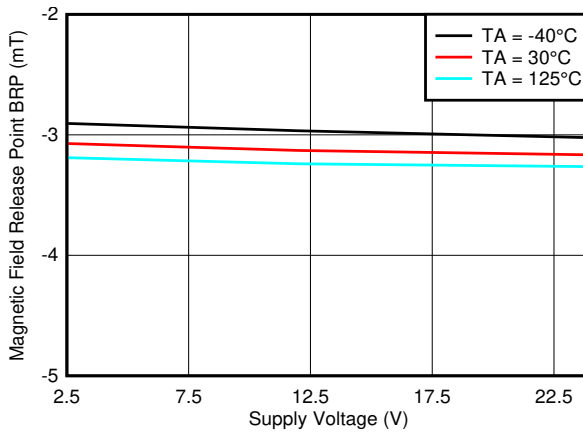
图 7-47. B_{RP\_X} 阈值与 V_{CC}
