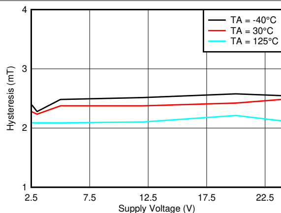
图 7-5. Hysteresis_Z 与 V_{CC}
