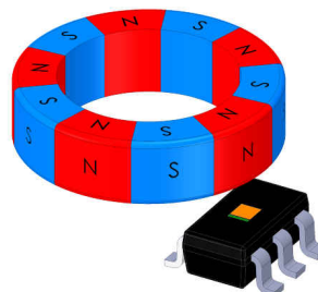
图 8-14. ZX 侧边缘 2
