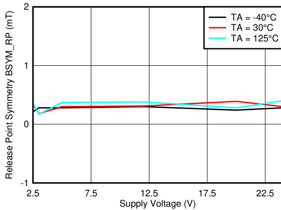
图 7-27. BSYM_RP(ZX) 与 VCC
