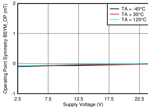
图 7-33. B_{SYM\_OP(XY)} 与 V_{CC}
