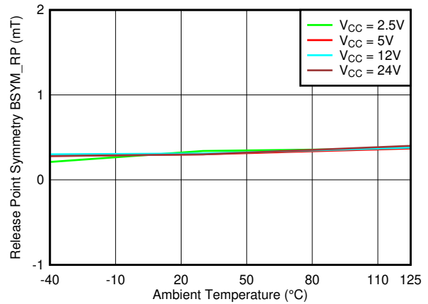
图 7-28. BSYM_RP(ZX) 与温度
