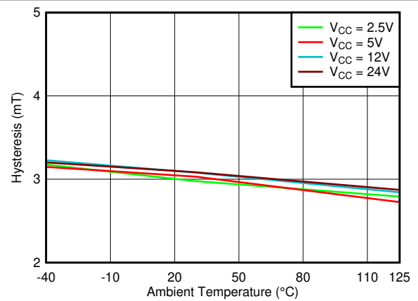
图 7-18. Hysteresis_Y 与温度
