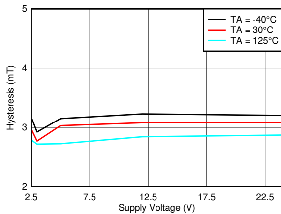
图 7-17. Hysteresis_Y 与 V CC
