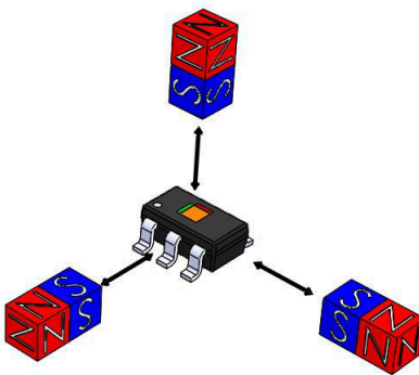
图 8-4. 轴极性
