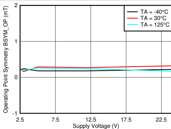
图 7-29. BSYM_OP(ZY) 与 VCC
