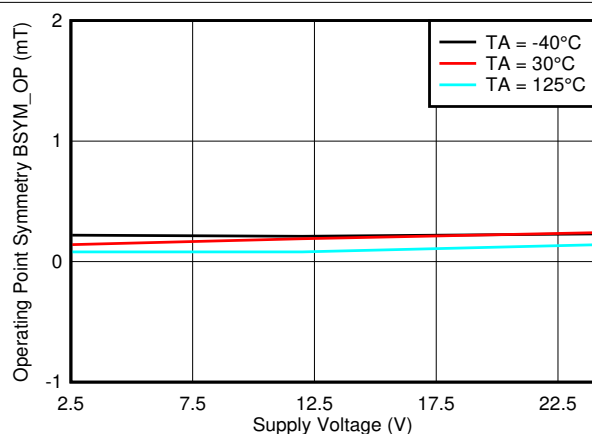
图 7-67. B_{SYM\_OP(ZY)} 与 V_{CC}
