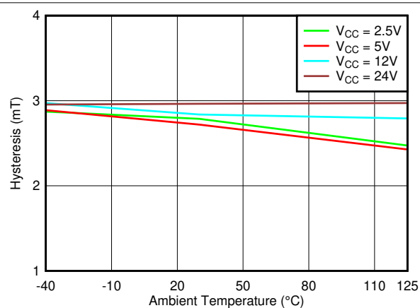
图 7-12. Hysteresis_X 与温度
