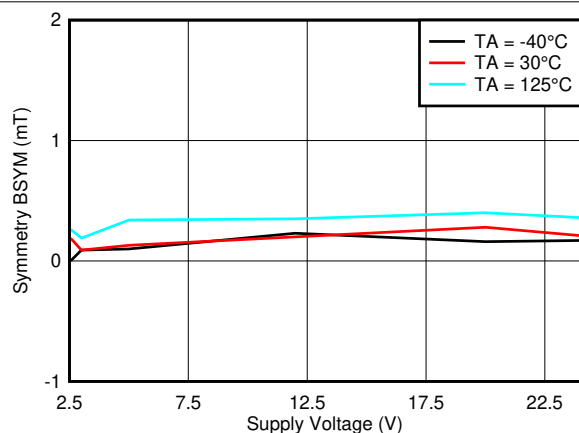
图 7-19. B_{SYM(Z)} 与 V_{CC}
