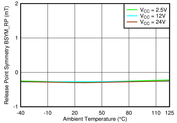
图 7-74. B_{SYM\_RP(XY)} 与温度
