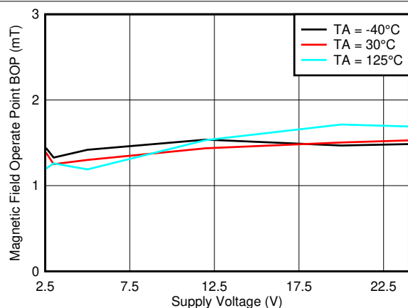
图 7-7. BOP_X 阈值与 VCC
