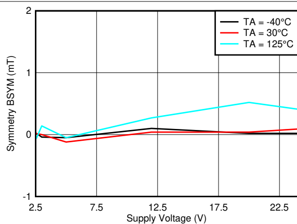
图 7-21. B_{SYM(X)} 与 V_{CC}
