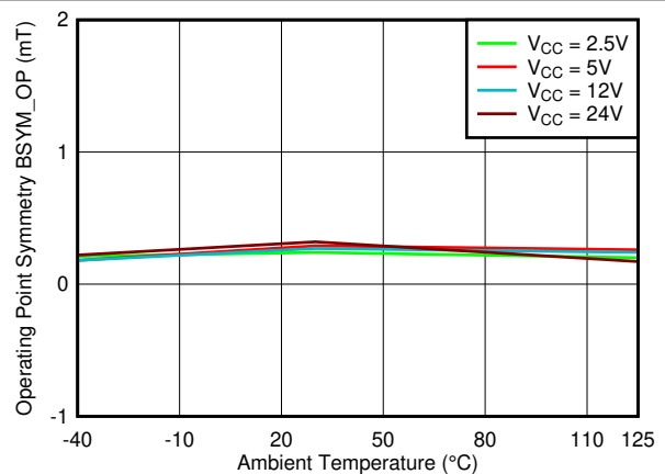
图 7-30. BSYM_OP(ZY) 与温度
