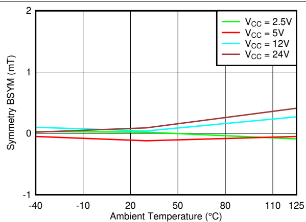
图 7-22. B_{SYM(X)} 与温度
