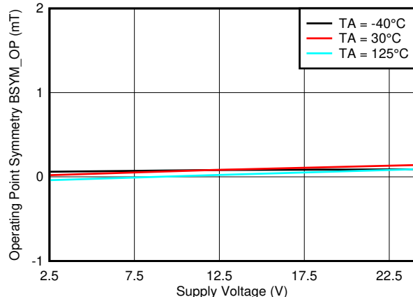
图 7-63. B_{SYM\_OP(ZX)} 与 V_{CC}
