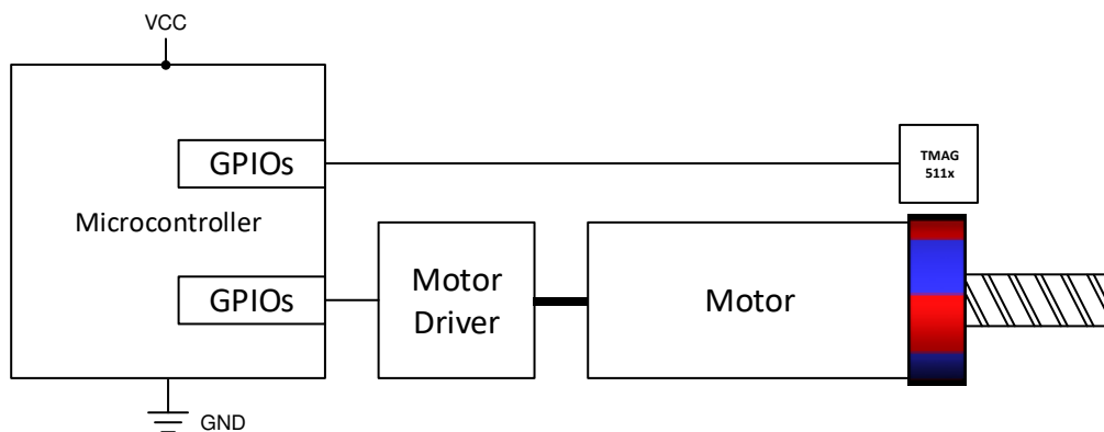
图 9-1. 增量编码
