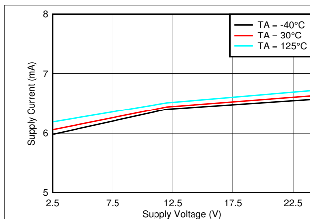
图 7-75. 电源电流与 V_{CC}
