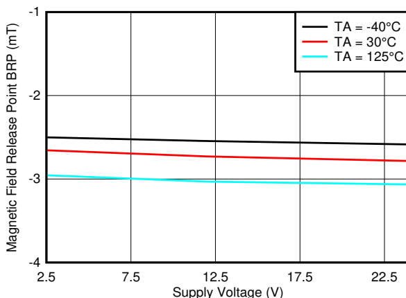
图 7-53. B_{RP\_Y} 阈值与 V_{CC}
