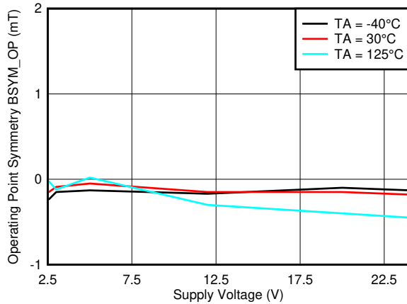
图 7-25. BSYM_OP(ZX) 与 VCC
