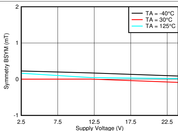
图 7-61. B_{SYM(Y)} 与 V_{CC}
