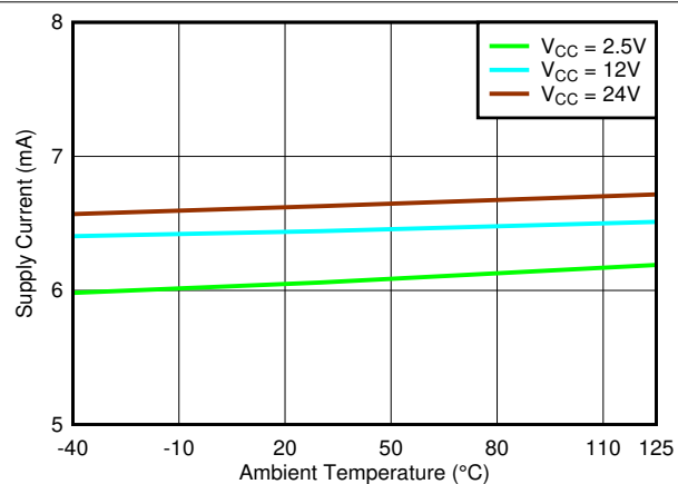
图 7-76. 电源电流与温度间的关系
