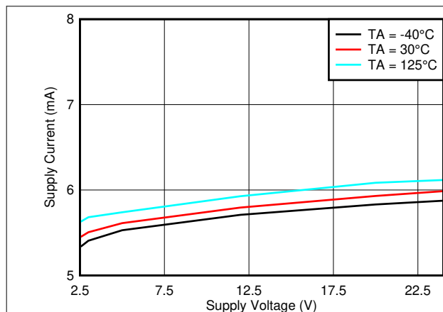
图 7-37. 电源电流与 V_{CC}
