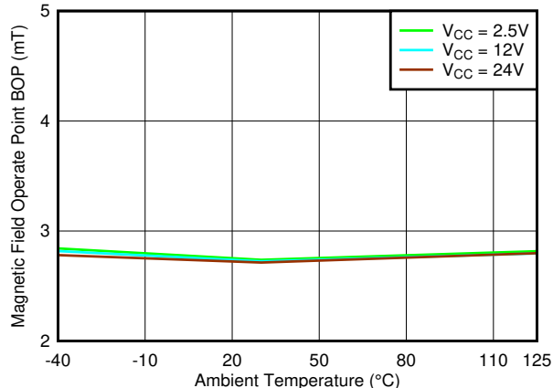
图 7-52. B_{OP\_Y} 阈值与温度
