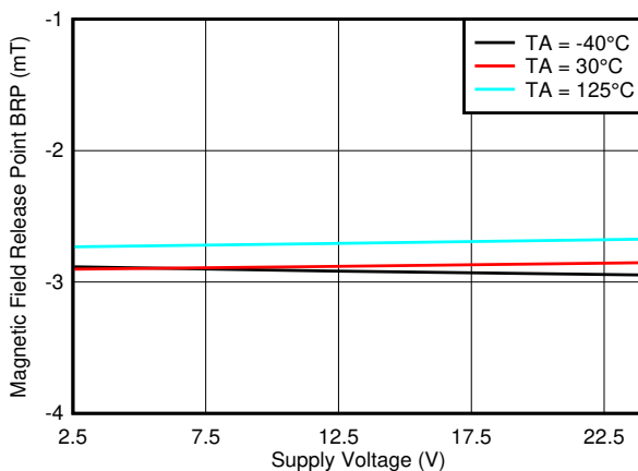
图 7-41. B RP_Z 阈值与 V CC
