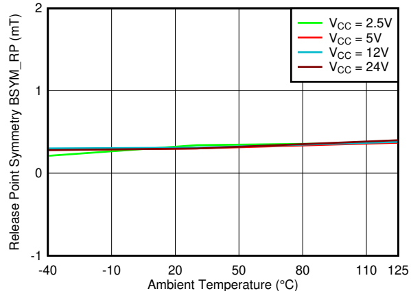
图 7-32. B_{SYM\_RP(ZY)} 与温度
