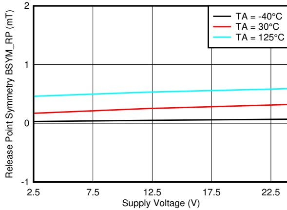
图 7-69. B_{SYM\_RP(ZY)} 与 V_{CC}
