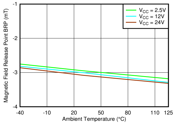
图 7-48. B_{RP\_X} 阈值与温度
