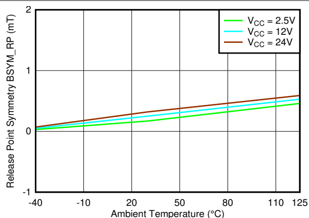
图 7-66. B_{SYM\_RP(ZX)} 与温度
