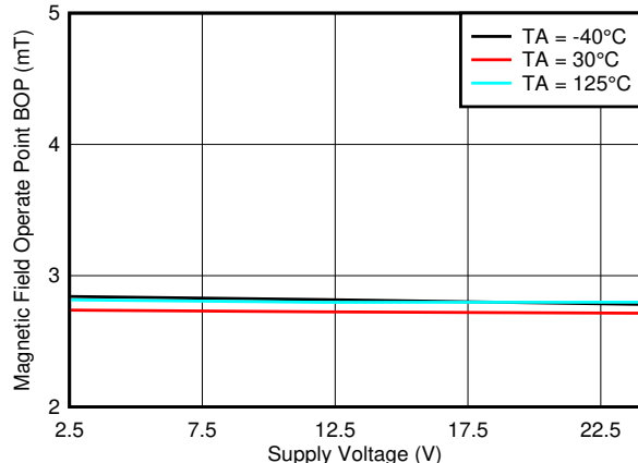
图 7-51. B_{OP\_Y} 阈值与 V_{CC}
