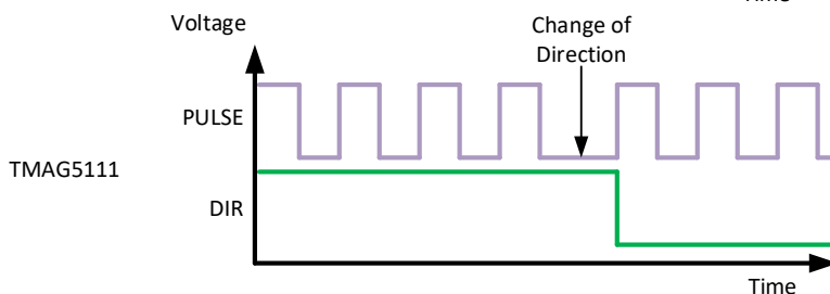
器件输出
