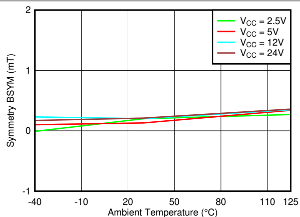
图 7-20. B_{SYM(Z)} 与温度
