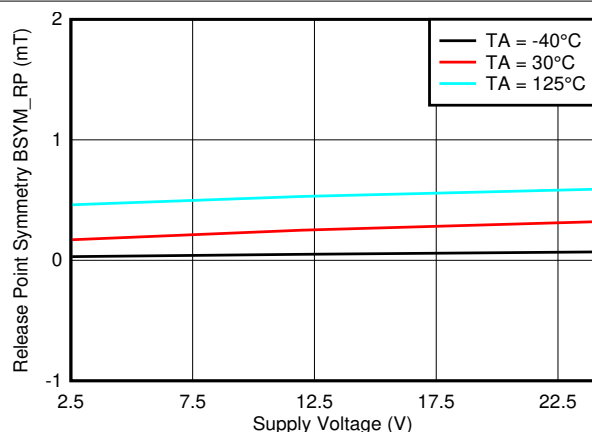
图 7-65. B_{SYM\_RP(ZX)} 与 V_{CC}
