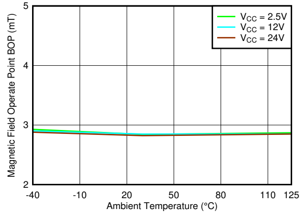
图 7-46. B_{OP\_X} 阈值与温度
