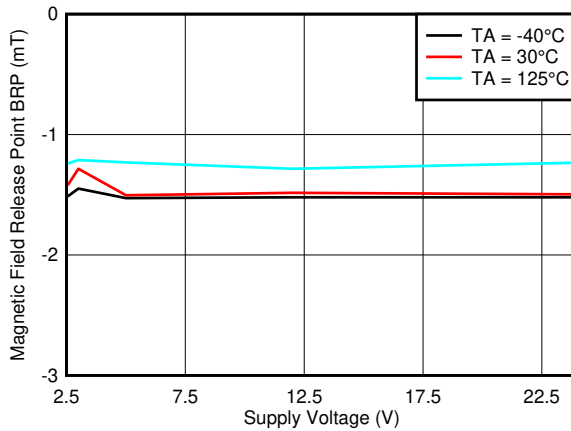
图 7-15. B RP_Y 阈值与 V CC
