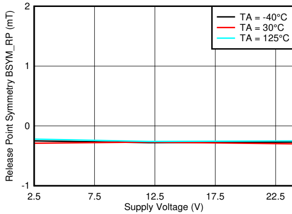
图 7-73. B_{SYM\_RP(XY)} 与 V_{CC}
