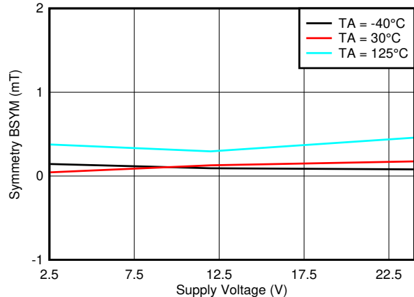
图 7-57. B_{SYM(Z)} 与 V_{CC}
