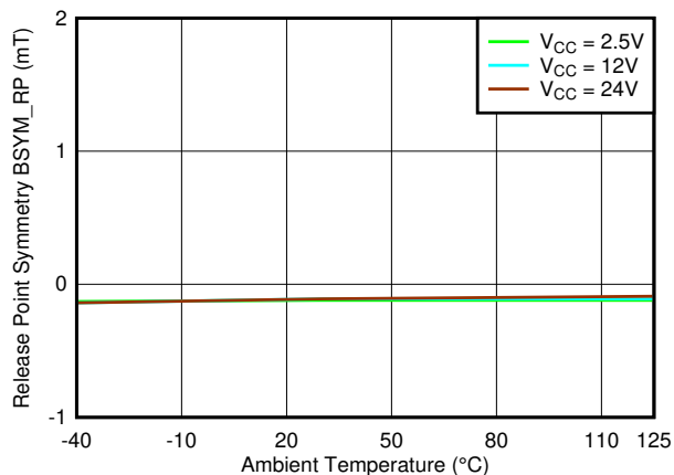
图 7-36. B_{SYM\_RP(XY)} 与温度
