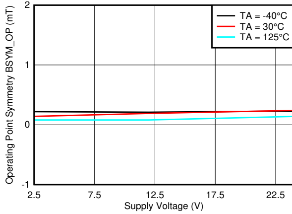
图 7-71. B_{SYM\_OP(XY)} 与 V_{CC}
