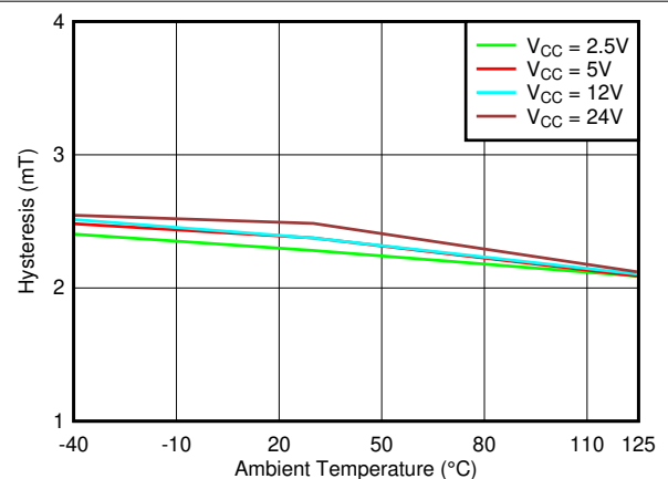
图 7-6. Hysteresis_Z 与温度
