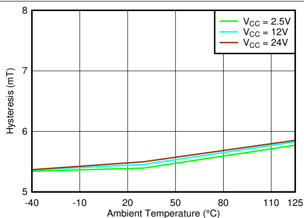
图 7-56. Hysteresis_Y 与温度
