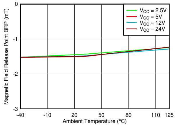
图 7-16. B RP_Y 阈值与温度
