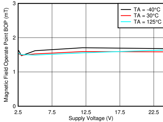
图 7-13. B OP_Y 阈值与 V CC
