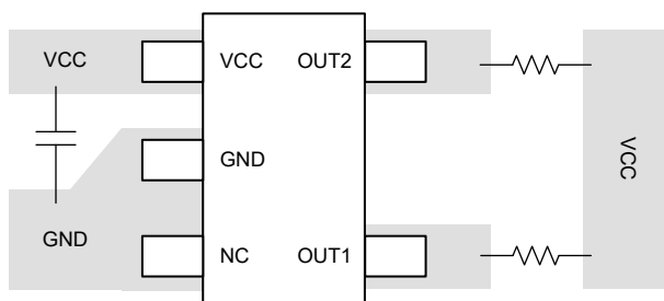
图 11-1. 布局示例
