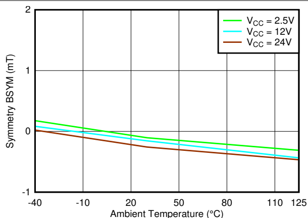
图 7-60. B_{SYM(X)} 与温度
