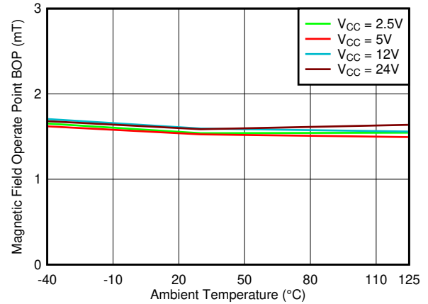
图 7-14. B OP_Y 阈值与温度
