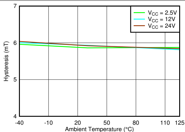
图 7-44. Hysteresis_Z 与温度
