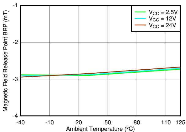
图 7-42. B RP_Z 阈值与温度
