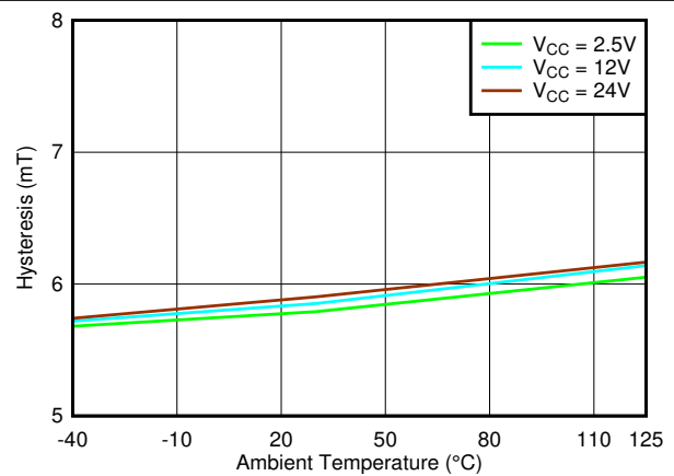
图 7-50. Hysteresis\_X 与温度
