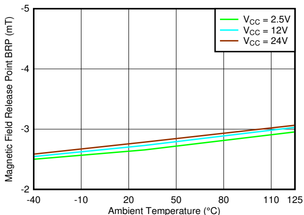
图 7-54. B_{RP\_Y} 阈值与温度
