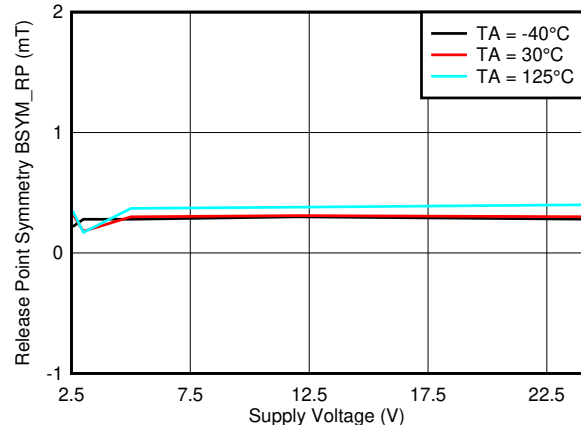
图 7-31. B_{SYM\_RP(ZY)} 与 V_{CC}
