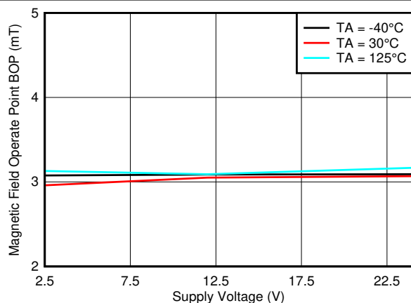
图 7-39. B OP_Z 阈值与 V CC
