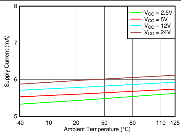
图 7-38. 电源电流与温度间的关系
