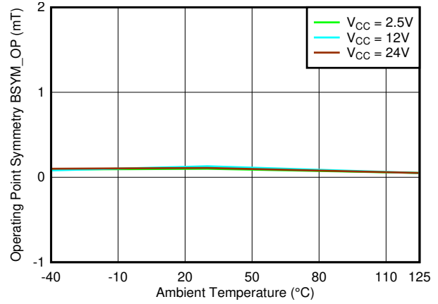
图 7-72. B_{SYM\_OP(XY)} 与温度
