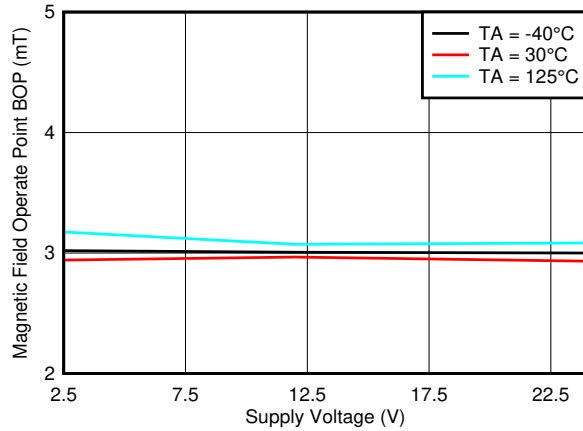
图 7-45. B_{OP\_X} 阈值与 V_{CC}
