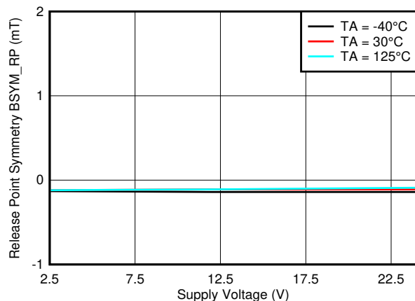
图 7-35. B_{SYM\_RP(XY)} 与 V_{CC}
