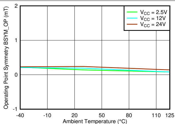
图 7-68. B_{SYM\_OP(ZY)} 与温度
