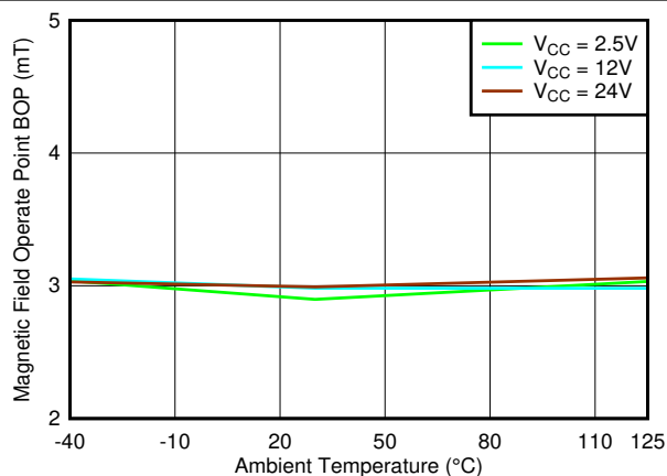
图 7-40. B OP_Z 阈值与温度
