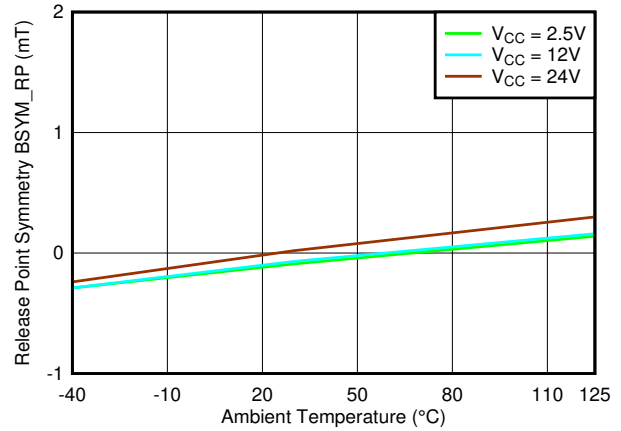
图 7-70. B_{SYM\_RP(ZY)} 与温度
