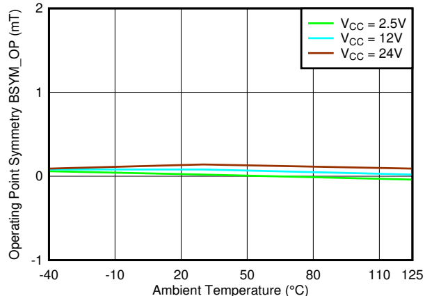
图 7-64. B_{SYM\_OP(ZX)} 与温度
