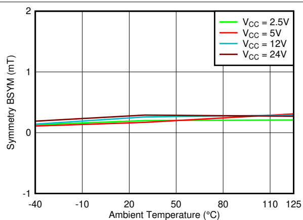
图 7-24. B_{SYM(Y)} 与温度
