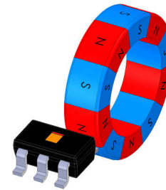
图 8-10. ZY 外边缘 1
