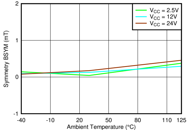
图 7-58. B_{SYM(Z)} 与温度
