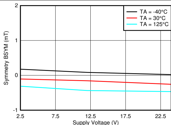
图 7-59. B_{SYM(X)} 与 V_{CC}
