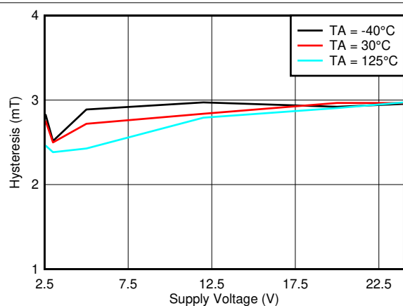
图 7-11. Hysteresis_X 与 VCC
