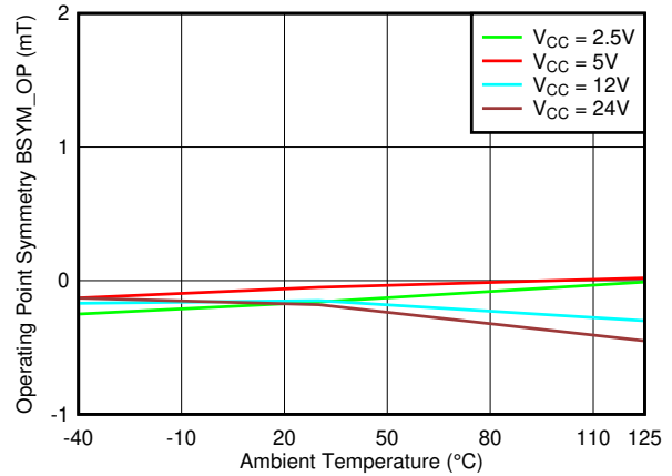
图 7-26. BSYM_OP(ZX) 与温度
