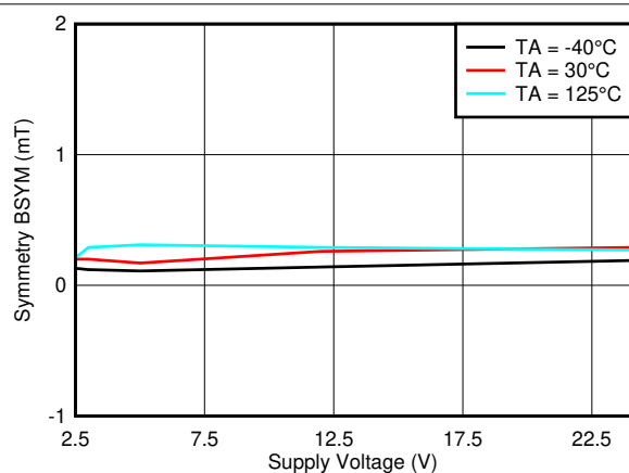
图 7-23. B_{SYM(Y)} 与 V_{CC}
