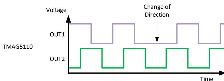
图 9-2. TMAG5110 输出响应
