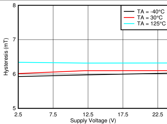
图 7-49. Hysteresis\_X 与 V_{CC}
