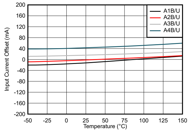
图 7-2. TMCS1108 输入失调电流与温度间的关系
