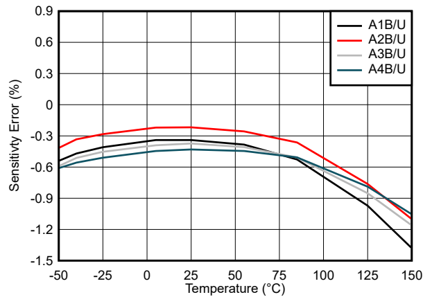
图 7-1. TMCS1108 灵敏度误差与温度间的关系
