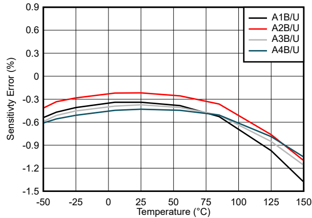
图 7-1. TMCS1107 灵敏度误差与温度间的关系
