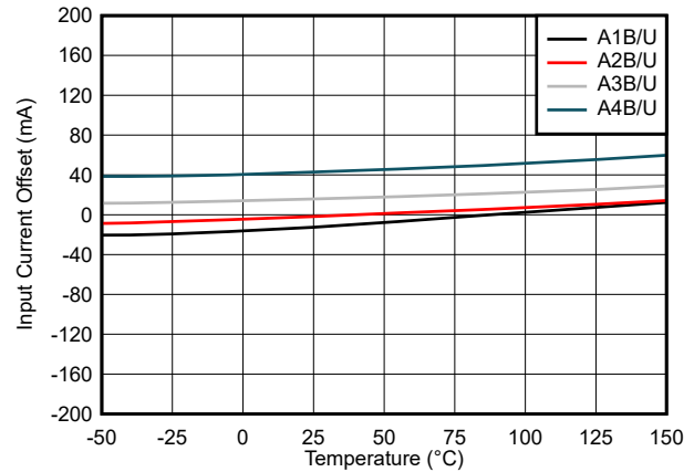
图 7-2. TMCS1107 输入失调电流与温度间的关系
