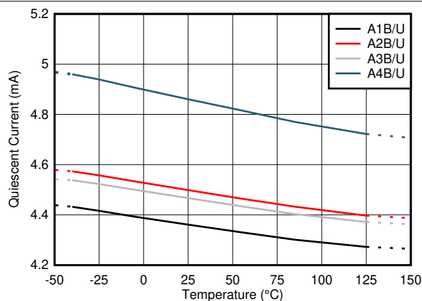
图 7-7. 静态电流与温度间的关系
