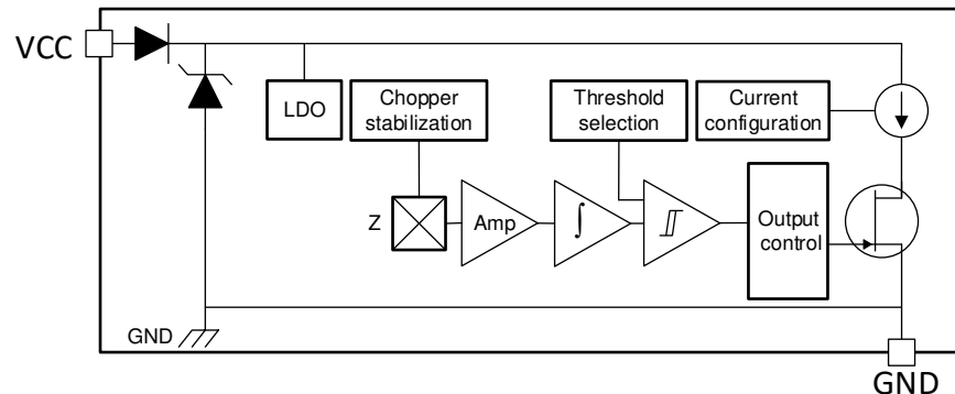
图 8-1. Block Diagram
