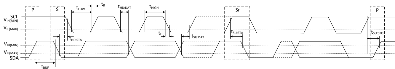
图 6-1. I 2 C 时序图
