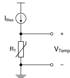
图 8-2. 线性热敏电阻的电流偏置电路
