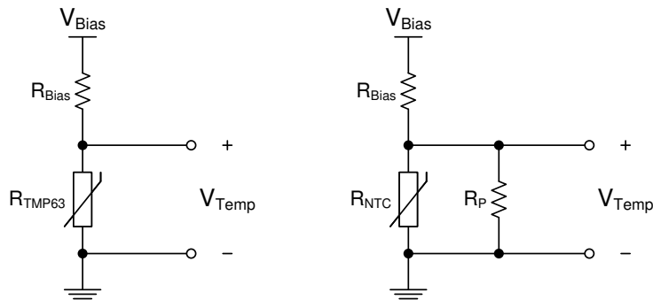
图 8-7. TMP63-Q1 与带线性化电阻 ( R_P ) 分压器电路的 NTC
