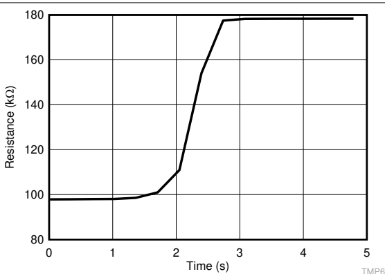
图 6-7. 阶跃响应
