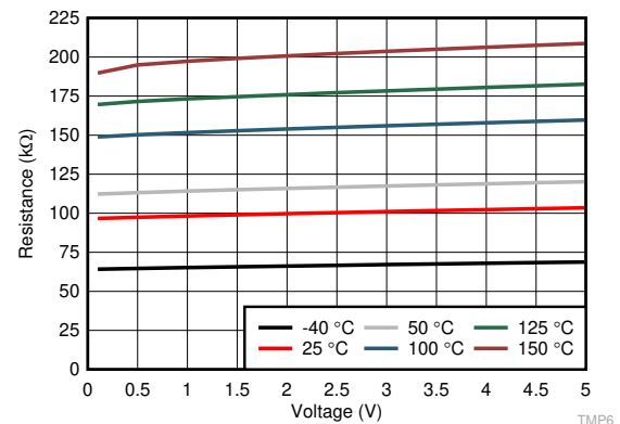
图 6-6. 电源相关电阻与偏置电压间的关系
