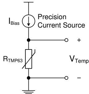
图 8-6. 带电流源的偏置电路
