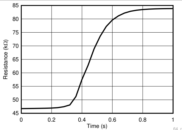
图 7-8. DEC 热响应时间
