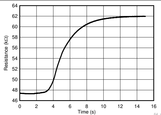
图 7-8. DEC 热响应时间
