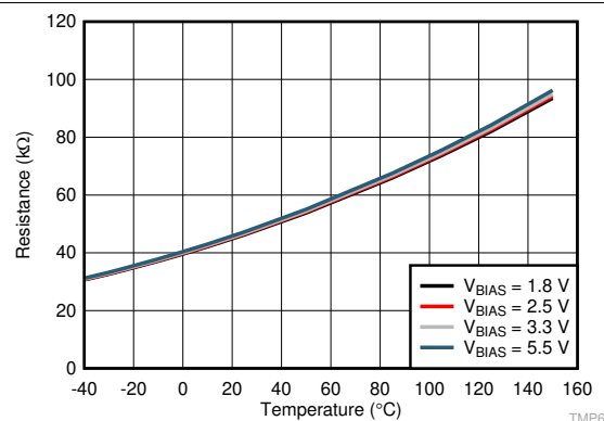
图 7-2. 使用多个偏置电压的电阻与环境温度间的关系
