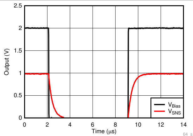
图 7-7. 阶跃响应
