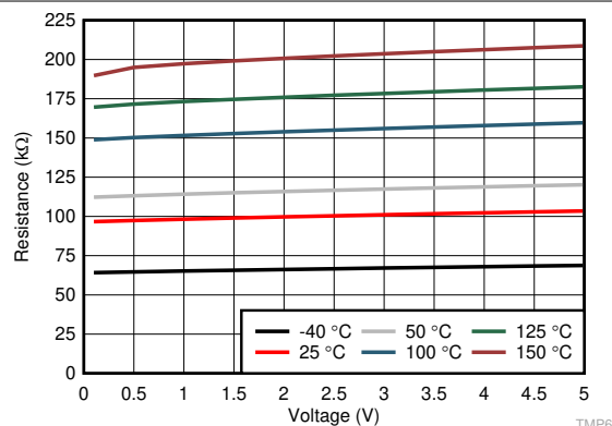
图 7-6. 电源相关电阻与偏置电压间的关系
