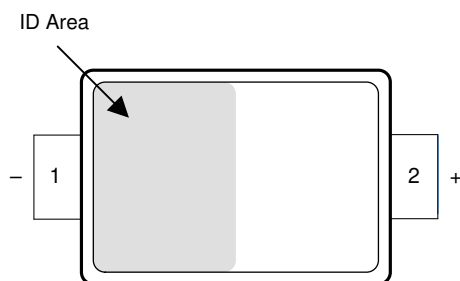
图 6-2. DYA 封装 2 引脚 SOT-5X3 顶视图
