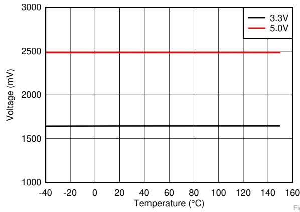
图 5-1. 静态电压与温度之间的关系
