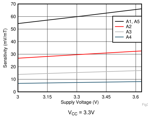
图 5-3. 灵敏度与电源电压之间的关系
