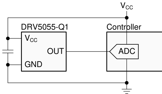
典型原理图
