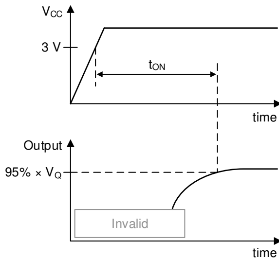
图 6-4. t_{ON} 定义
