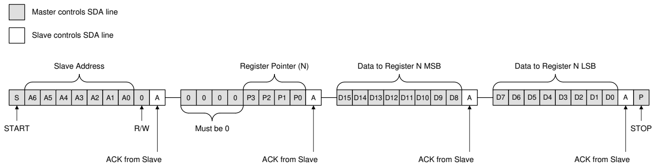
图 7-9. 写入字命令时序图
