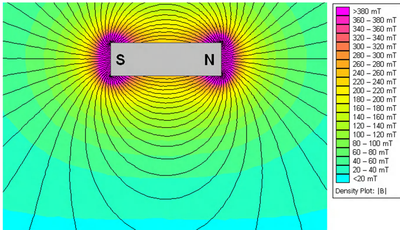
图 7-3. 仿真磁通
