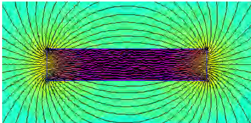
图 9-5. 典型磁通线
