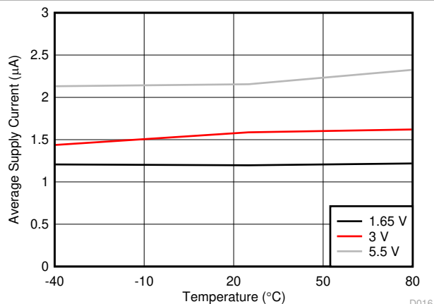
图 7-1. I_{CC(AVG)} 与温度间的关系 (20Hz 版本)
