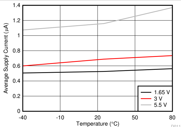
图 7-2. I_{CC(AVG)} 与温度间的关系 (5Hz 版本)
