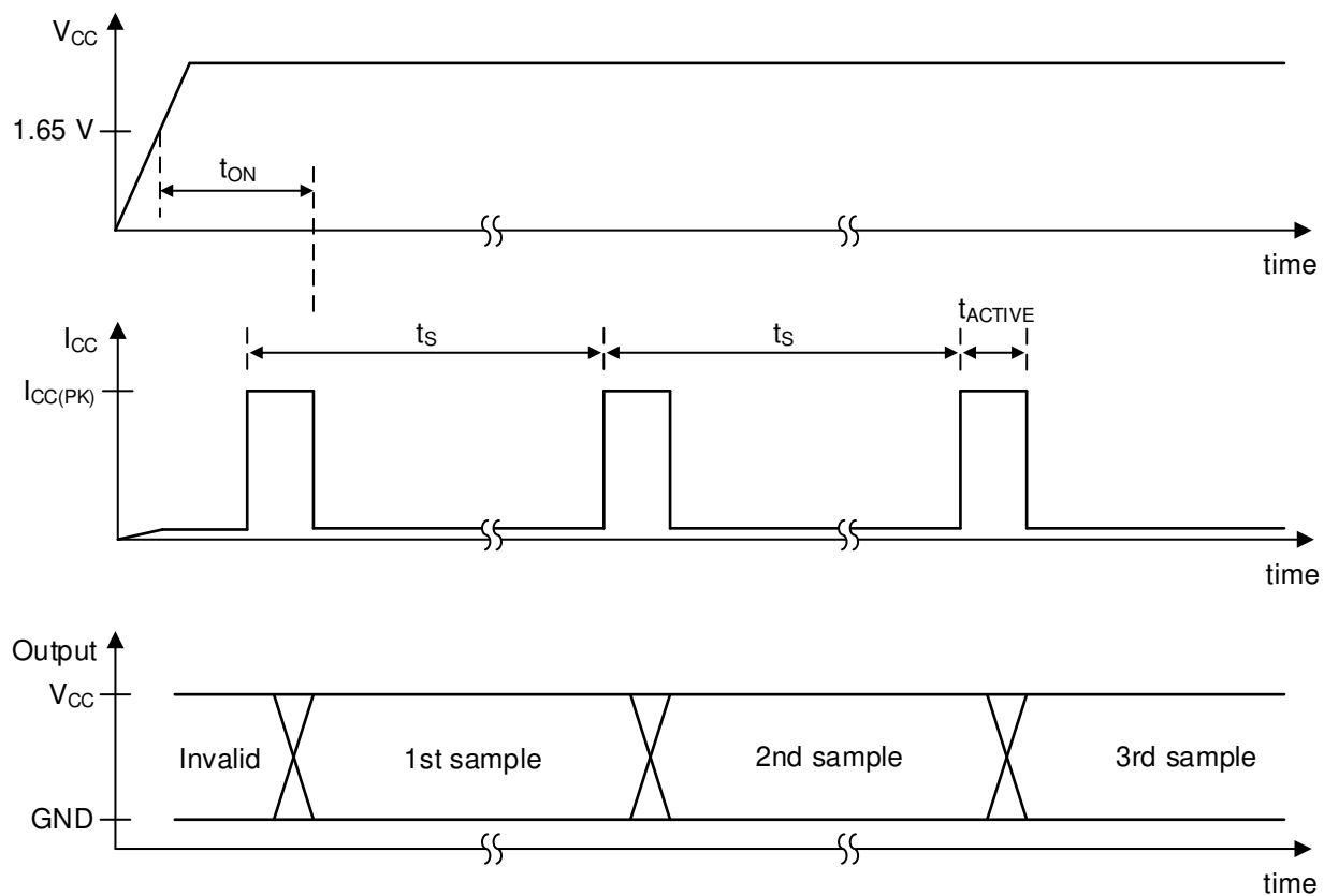
图 8-7. 时序图
