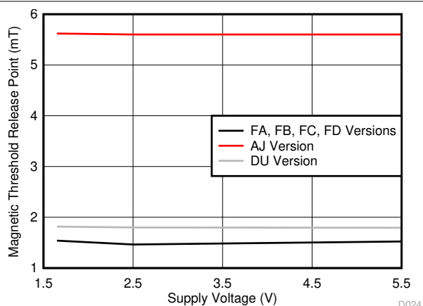
图 7-6. |B_{RP}| 与 V_{CC} 间的关系
