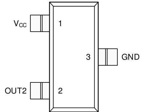
图 6-2. DU 版本 DBZ 封装 3 引脚 SOT-23 顶视图
