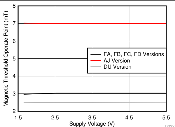
图 7-5. |B_{OP}| 与 V_{CC} 间的关系
