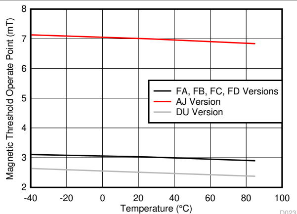
图 7-3. |B_{OP}| 与温度间的关系
