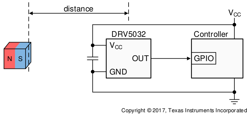
图 9-1. 典型应用图
