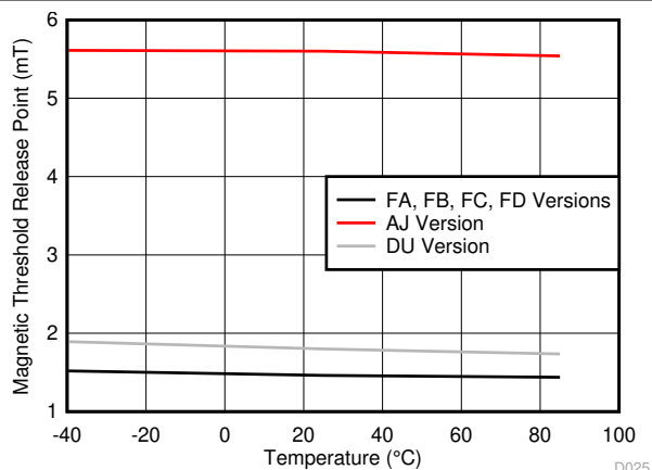
图 7-4. |B_{RP}| 与温度间的关系
