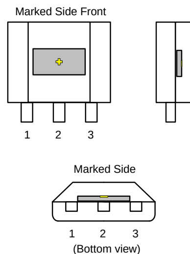
图 25. TO-92 (LPG) 封装
