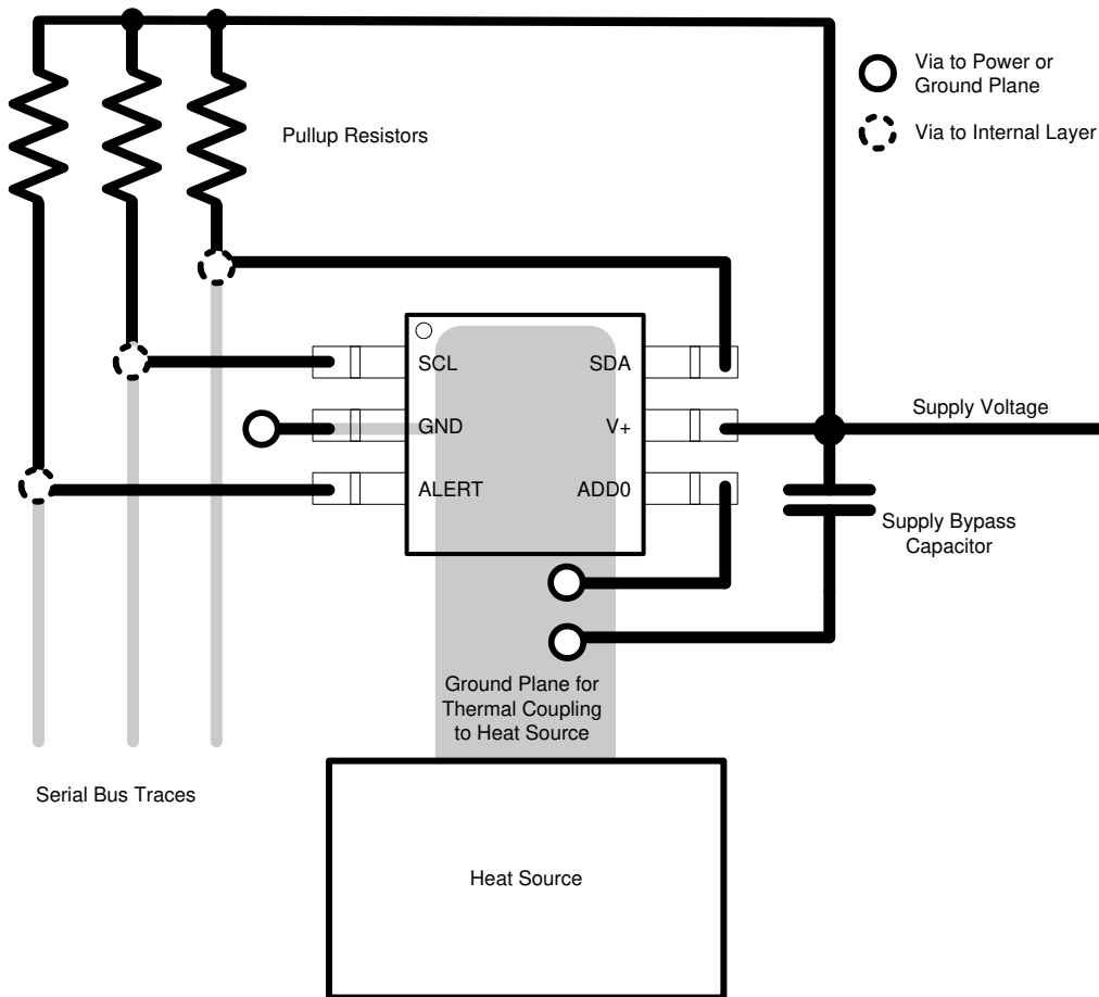
图 10-1. TMP102-Q1 布局示例
