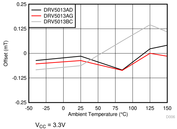
图 6-10. 偏移与温度之间的关系
