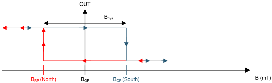
图 7-2. DRV5013 - B_{OP} > 0
