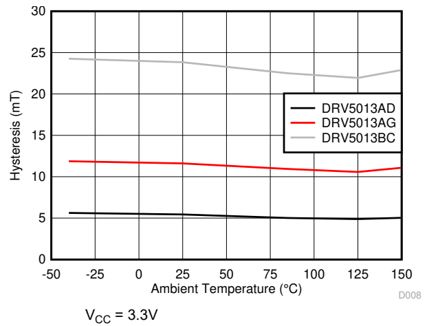
图 6-8. 迟滞与温度之间的关系
