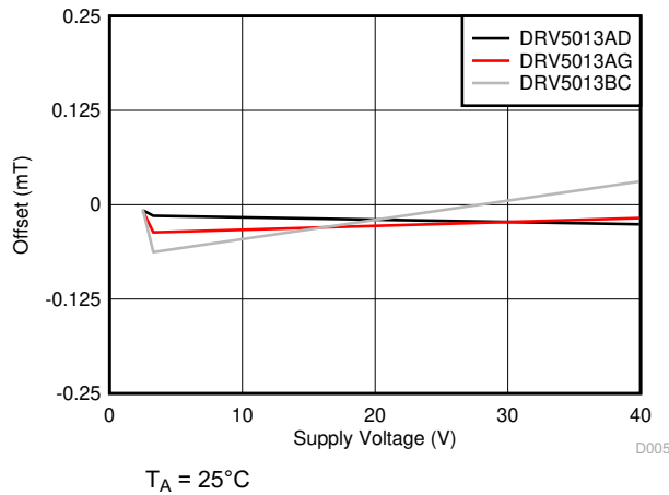
图 6-9. 偏移与 V_{CC} 之间的关系
