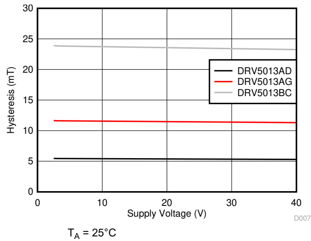
图 6-7. 迟滞与 V_{CC} 之间的关系
