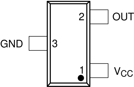
图 5-1. DBZ 封装 3 引脚 SOT-23 顶视图
