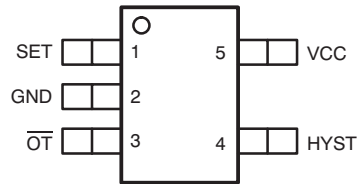
DBV 封装 SOT 23-5 (顶视图)
