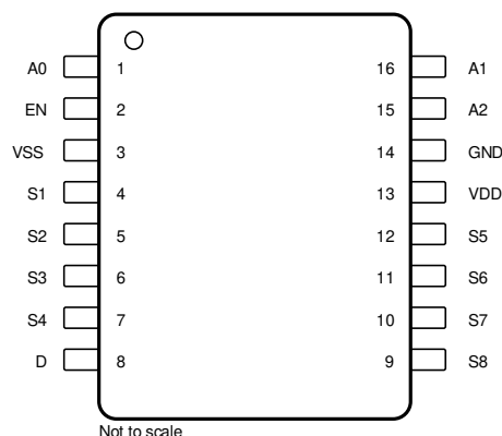
图 5-1. TMUX7208M : PW 封装, 16 引脚 TSSOP (顶视图)
