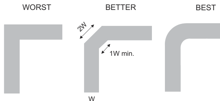
图 9-4. 布线示例
