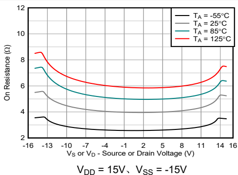
图 6-5. 导通电阻与温度间的关系
