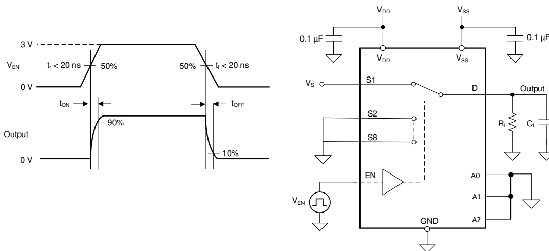
图 7-5. 导通和关断时间测量设置
