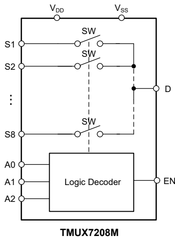
简化版方框图
