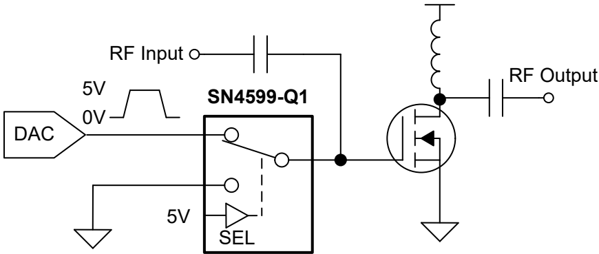
图 8-3. 功率放大器输入控制
