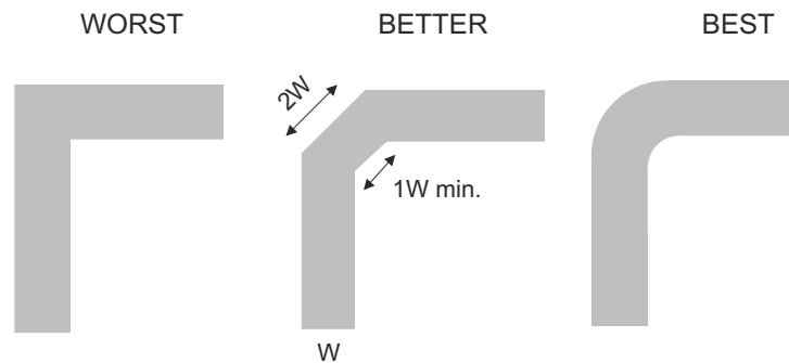
图 8-5. 布线示例
