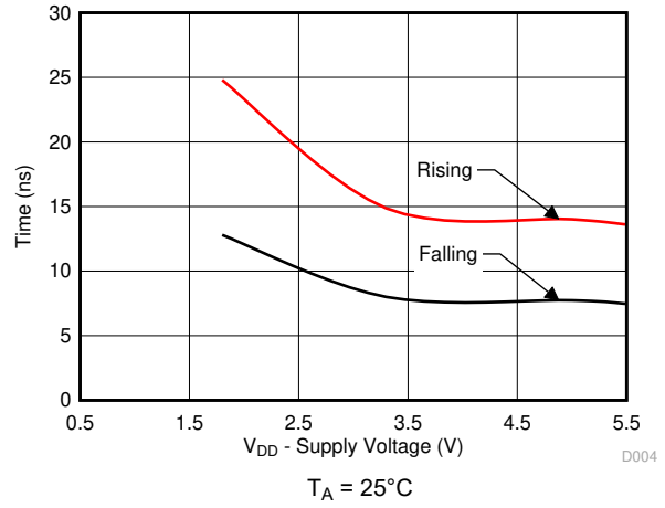
图 5-2. T_{\text{transition}} 与电源电压之间的关系
