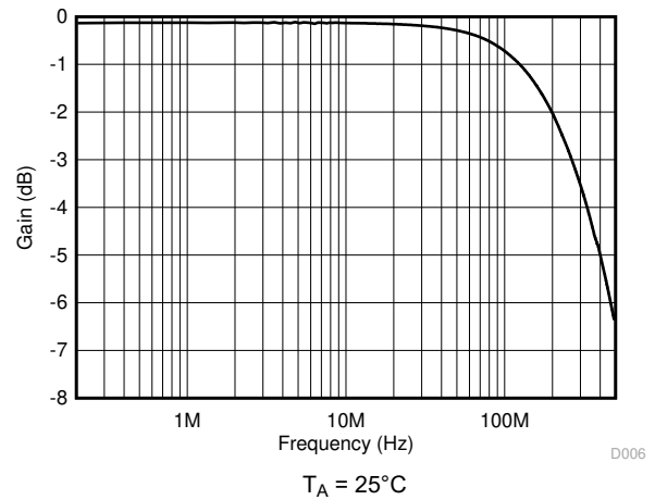
图 5-4. 频率响应
