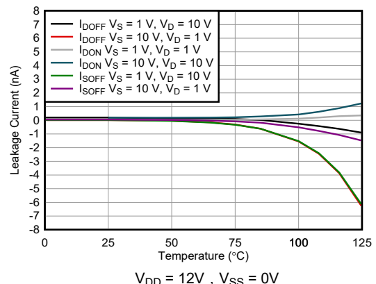
图 5-12. 漏电流与温度间的关系
