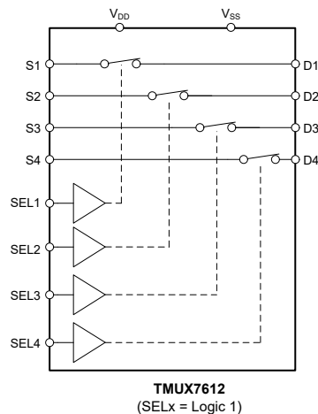
TMUX7612 方框图
