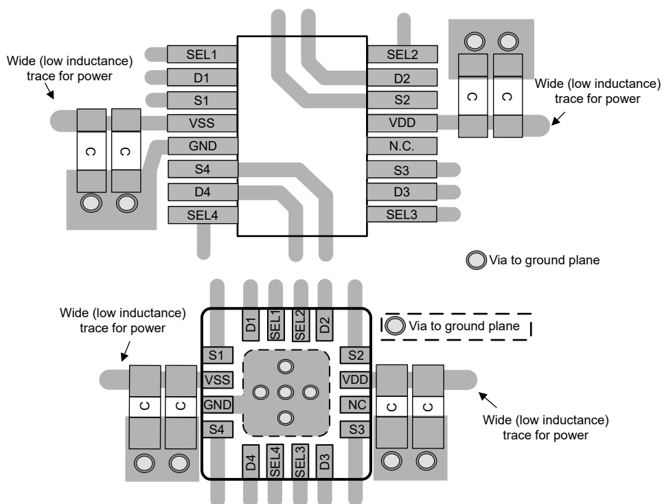
图 8-6. TMUX7612 Layout Example
