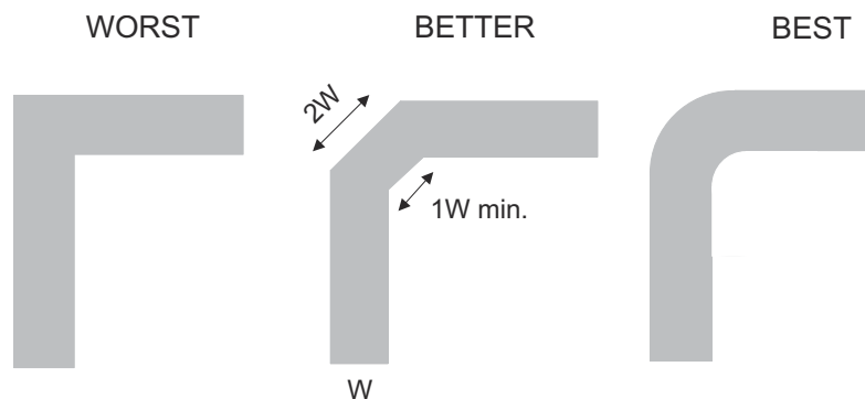
图 8-5. Trace Example
