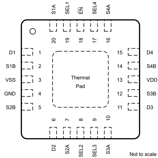
图 5-2. TMUX6234 RRQ Package, 20-Pin WQFN (Top View)
