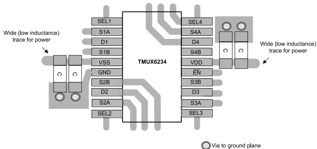
图 11-2. TMUX6234PW Layout Example
