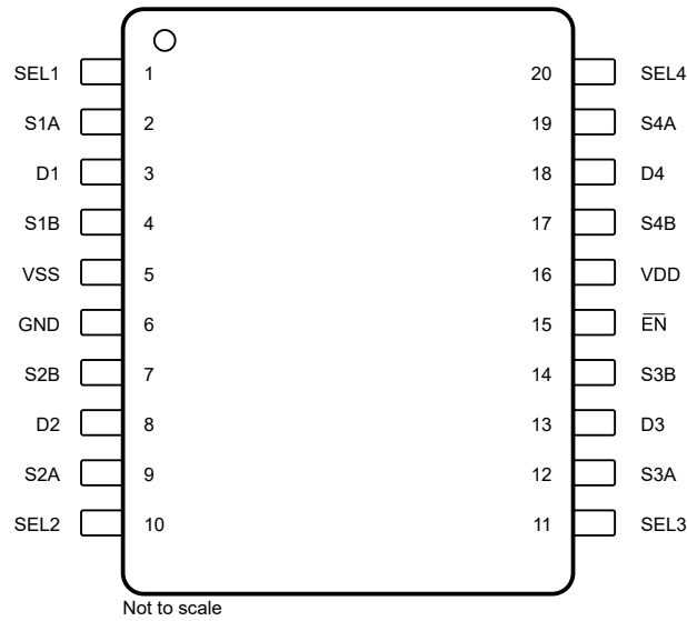
图 5-1. TMUX6234 PW Package, 20-Pin TSSOP (Top View)
