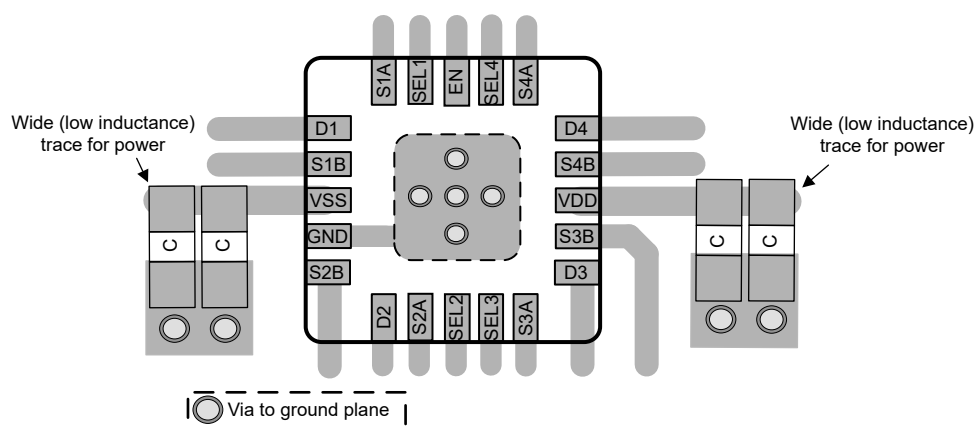
图 11-3. TMUX6234RRQ Layout Example
