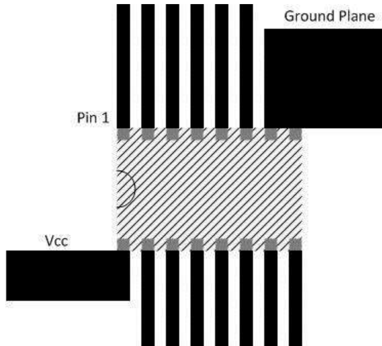
图 8-2. Layout Example Schematic
