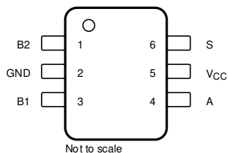
图 5-2. DCK 封装 6 引脚 SC70 顶视图
