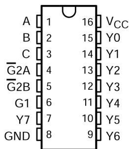
图 3-1. M Package (Top View)
