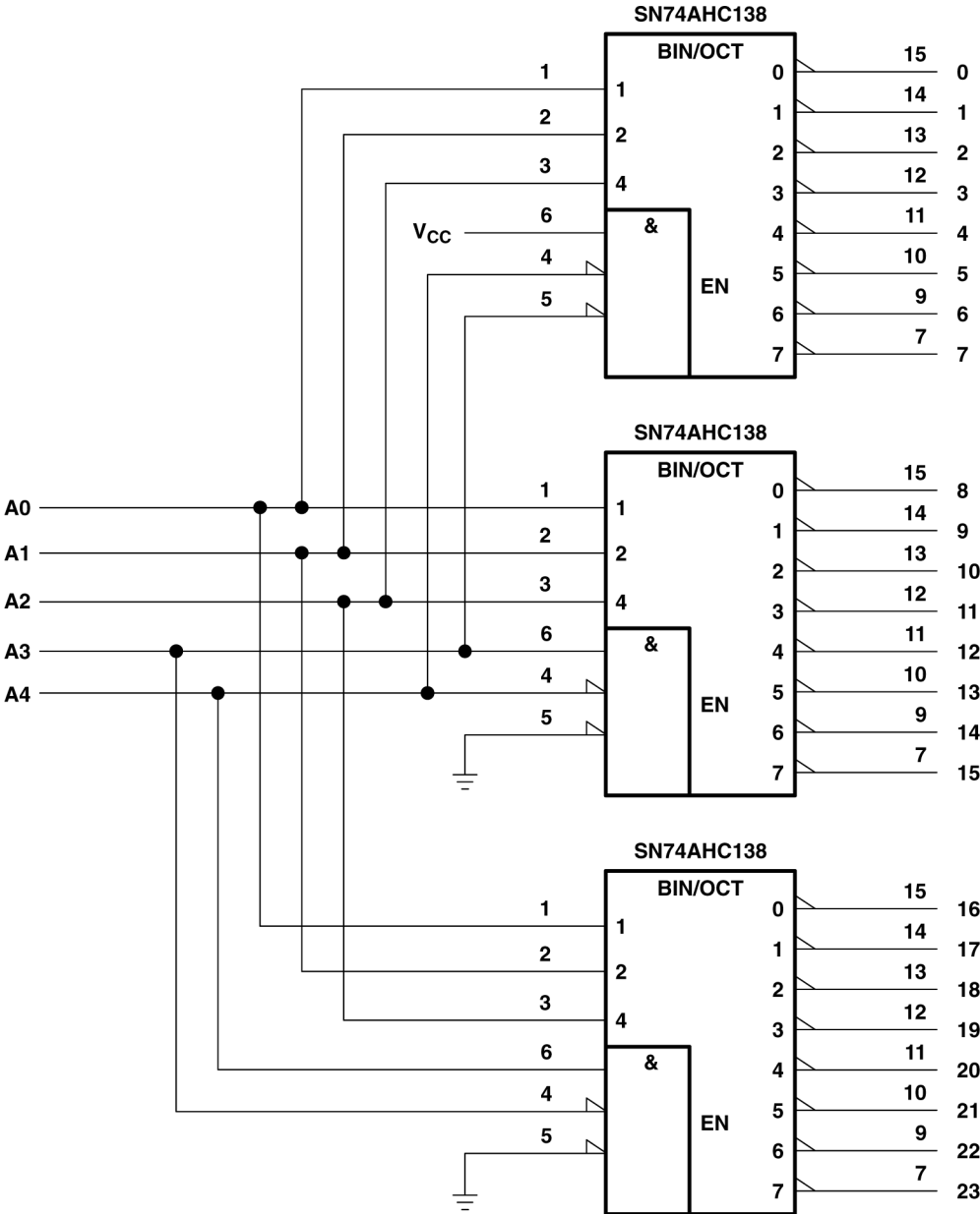
图 7-1. 24 位解码方案
