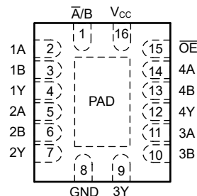
图 5-2. BQB 封装，16 引脚 WQFN（透明顶视图）
