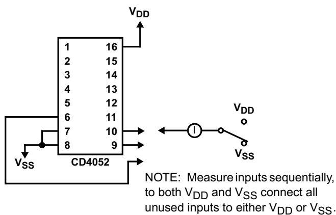
图 7-12. Input Current
