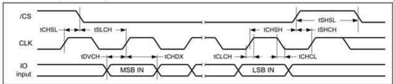
图 6-5. SPI Timing
