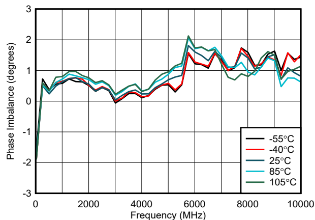
图 5-32. 相位不平衡
