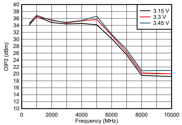
图 5-8. 整个 V_{DD} 范围内的 OIP3
