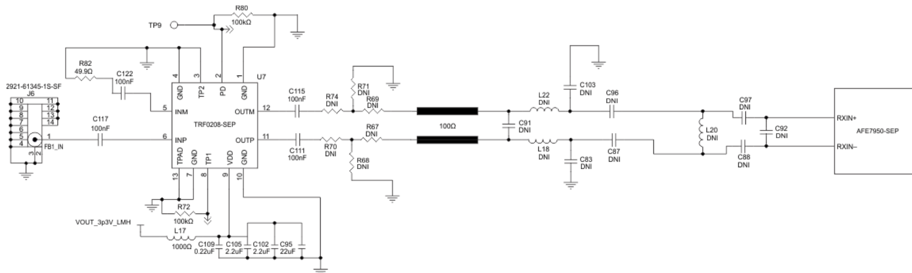
图 7-4. TRF0208-SEP 在采用 AFE7950-SEP 的接收链中
