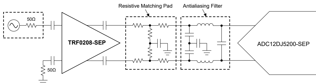
图 7-1. 与 ADC12DJ5200-SEP 连接
